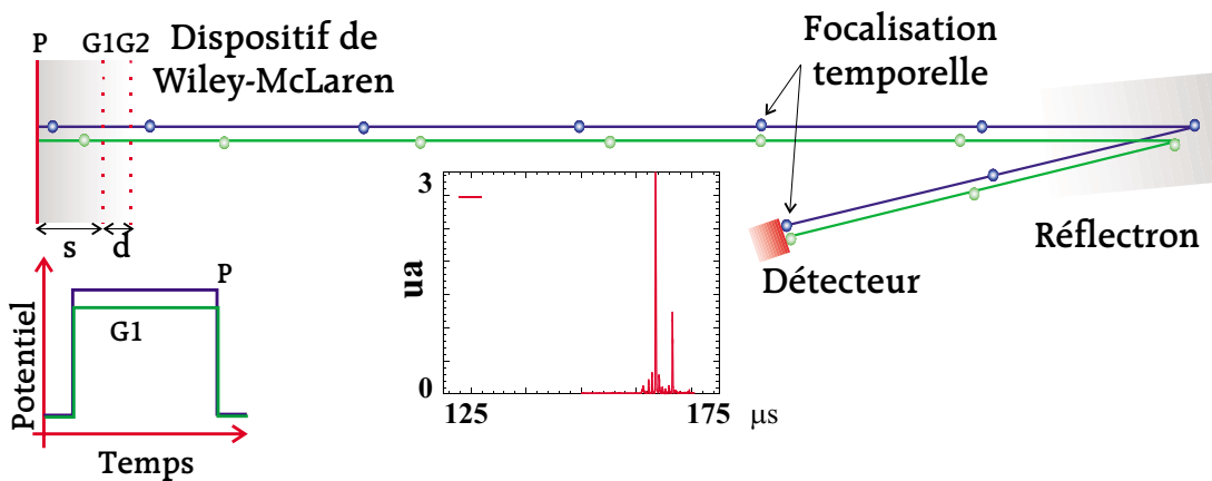
FIGURE 2.1: Description du mode de fonctionnement classique du dispositif de WILEY - MCLAREN. Le potentiel appliqué aux plaques est schématisé. Un exemple de spectre issu d'un tel dispositif est représenté.
