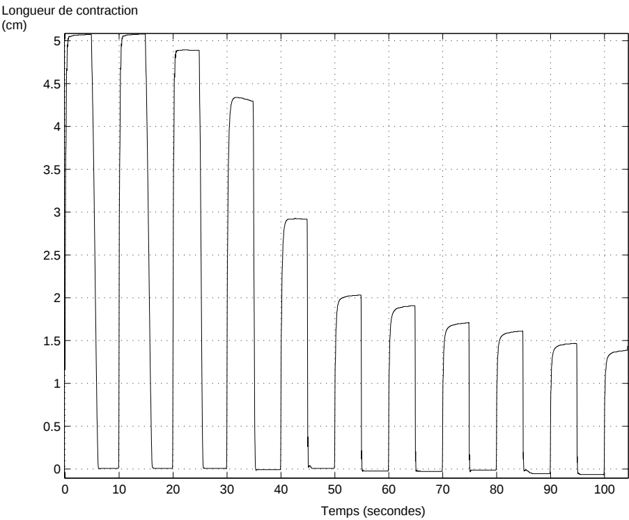
FIG. 2.19 – Réponse en longueur à une crevaision
