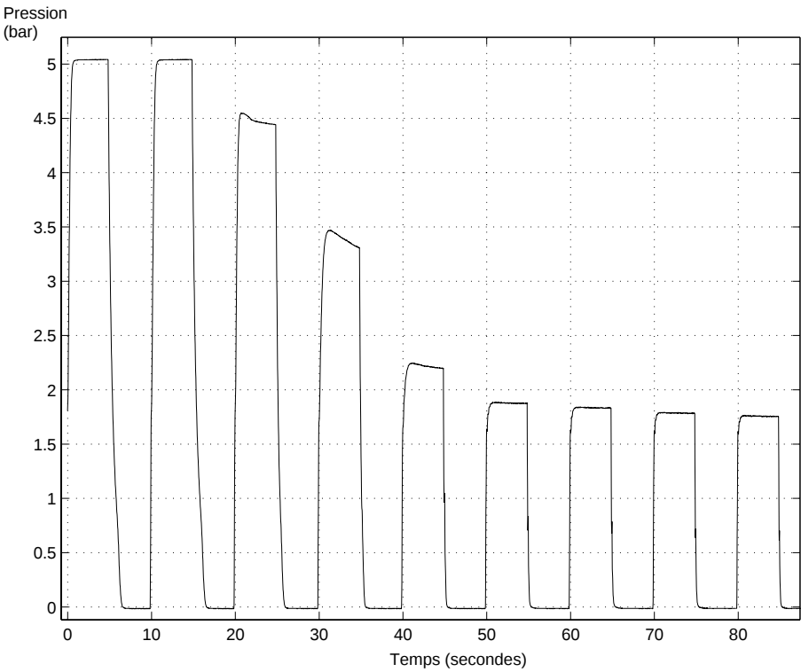
FIG. 2.20 – Réponse en pression à une crevaision
