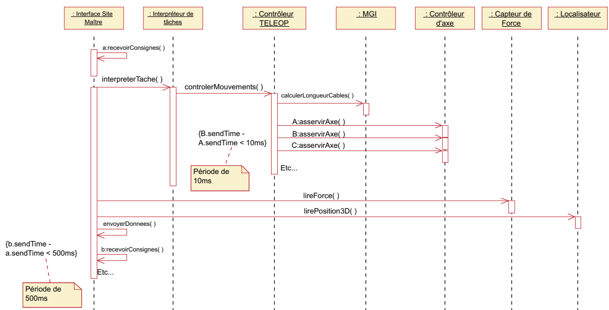
FIG. 5.38 – Diagramme de séquence du logiciel du scénario principal de Réaliser tâche
