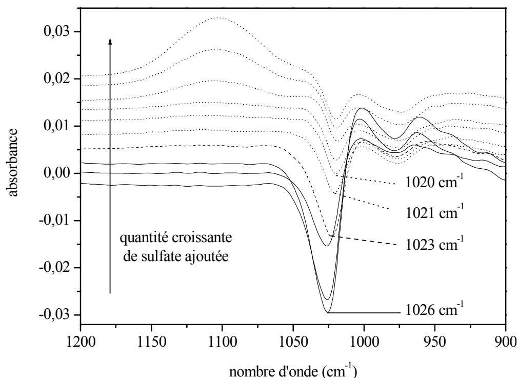
Figure IV. 18 : spectre infrarouge de différence des suspensions de gibbsite par rapport à la suspension initiale, en fonction de la quantité de sulfate ajoutée. Le facteur de soustraction du spectre sans sulfate a été ajusté pour minimiser le "S" et faciliter la mesure de l'aire du pic de sulfate à 1102\text{ cm}^{-1} .
