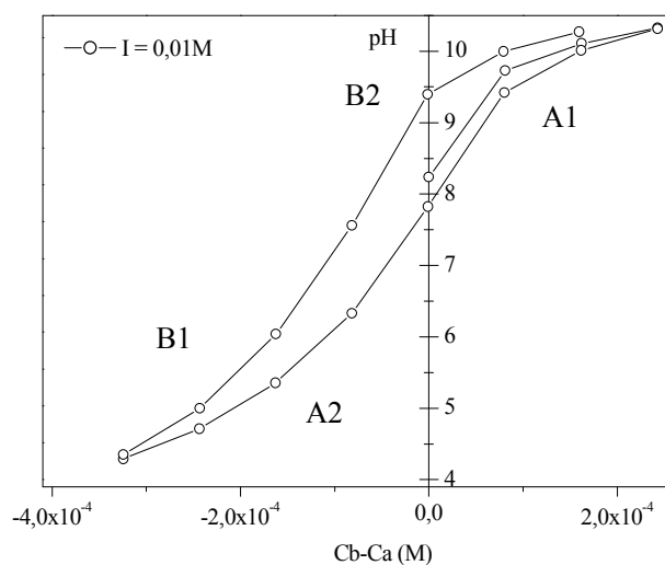
Figure IV. 7 : courbe de titrage originale. Gibbsite type G21, I = 0,01 \text{ M} , 32 \text{ g/L} , dialysée. A1 : ajout d'acide en milieu basique, A2 : ajout d'acide en milieu acide, B1 : ajout de base en milieu acide, B2 : ajout de base en milieu basique.
