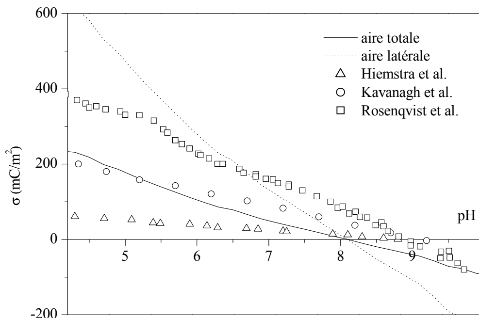
Figure IV. 15 : courbes de charge d'échantillons de gibbsite I = 0,1 M. (—) et (···) : gibbsite G21, 10 min d'équilibre ; (Δ) : (Hiemstra et al. , 1999), 2 min d'équilibre ; (○) : (Kavanagh et al. , 1975), 20-30 min d'équilibre ; (□) : (Rosenqvist et al. , 2002), 8-14h d'équilibre.
