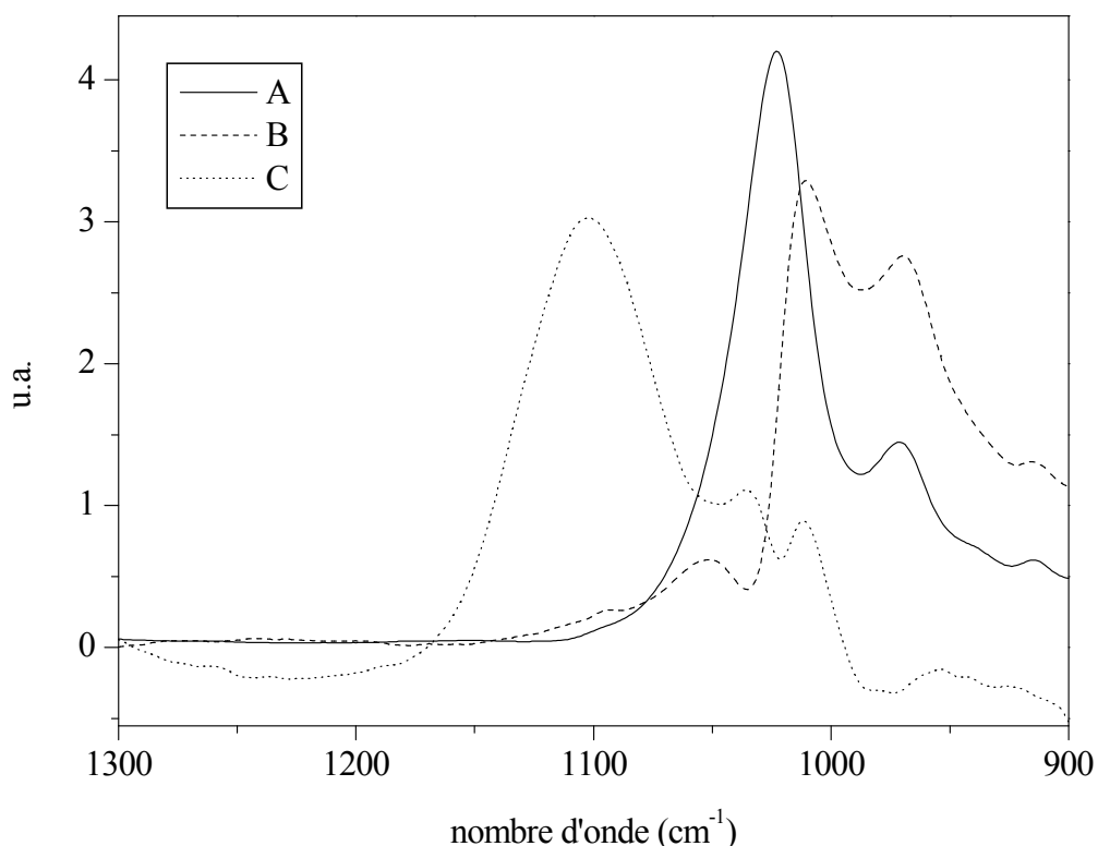
Figure IV. 19 : composantes des spectres de gibbsite en suspension en présence de sulfate, région des vibrations de déformation Al-O-H.
