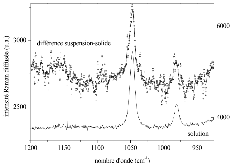
Figure IV. 24 : détail de la Figure IV. 23. Spectres de la solution (échelle de droite) et de la différence suspension-solide séché (échelle de gauche).
