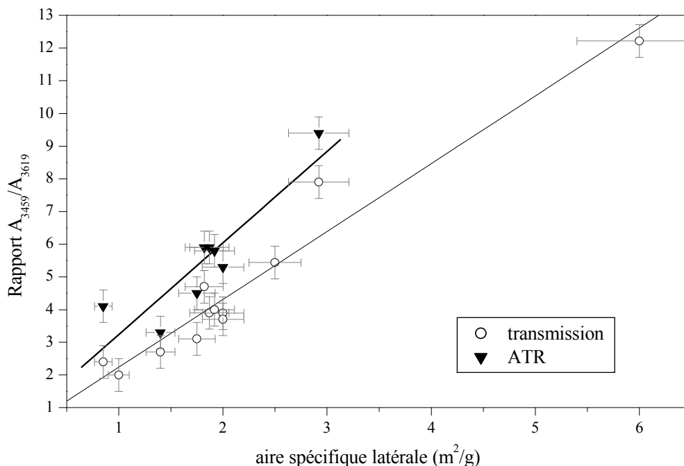
Figure III. 4 : correspondance du rapport des aires intégrées des pics à 3459 et 3619\text{ cm}^{-1} pour des spectres infrarouge en transmission obtenus pour des pastilles à 0,1% en masse dans KBr ou en mode ATR de différents échantillons de gibbsite.
