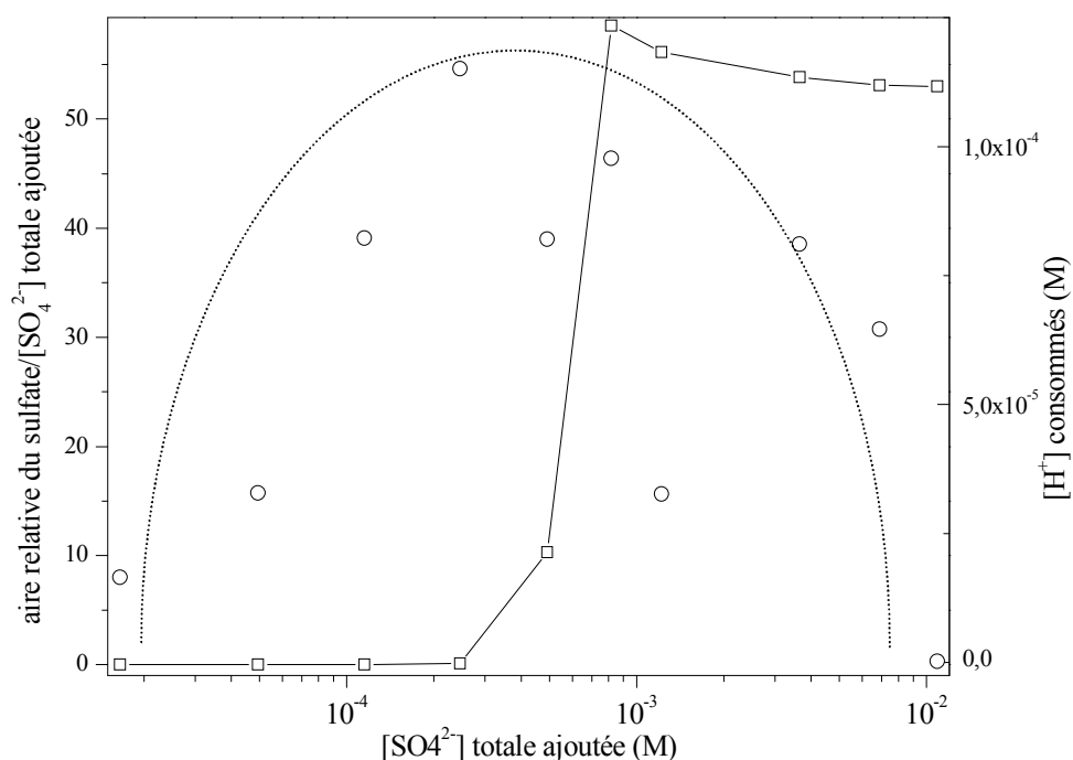
Figure IV. 17 : rapport de l'aire intégrée du pic à 1102 \text{cm}^{-1} et de la concentration initiale en sulfate (échelle de gauche) et consommation de protons ( \circ ) (échelle de droite), en fonction de la concentration totale ajoutée (échelle log). La courbe en pointillés est ajoutée pour faciliter la lecture.
