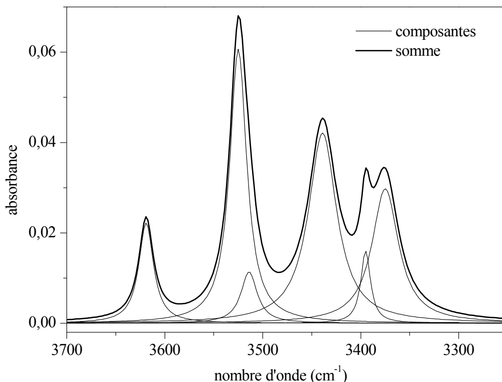
Figure III. 18 : spectre infrarouge des vibrations d'élongation des groupements OH du volume seul de la gibbsite obtenu à partir du spectre de la Figure III. 2 page 82 après élimination des contributions de la phase bayerite, des sites de surface et de l'eau.
