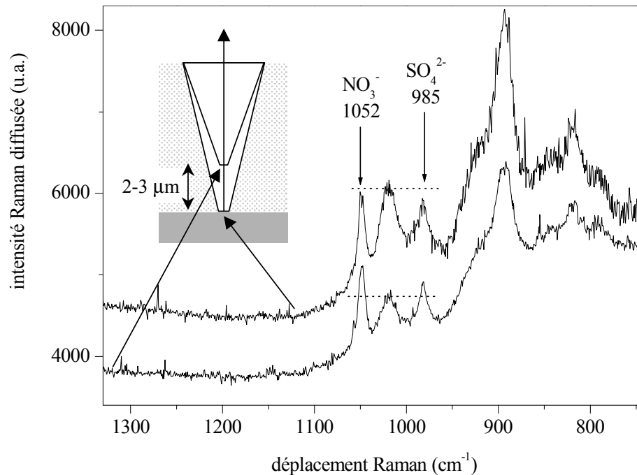
Figure IV. 22 : spectres de la suspension en fonction de la zone de focalisation, dans la solution ou à l'interface.
