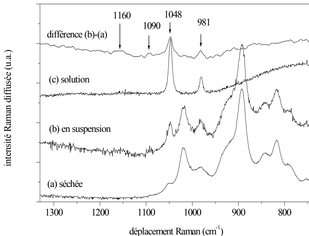
Figure IV. 23 : spectres Raman d'une gibbsite de type G25 : solide séché, gibbsite en suspension dans une solution de nitrate et sulfate, solution seule et différence suspension-solide séché.
