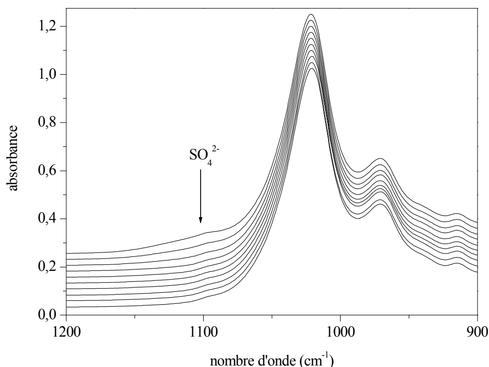
Figure IV. 16 : spectres des suspensions de gibbsite pour les différentes concentrations en sulfate ajouté. Spectres normés à 1020\text{ cm}^{-1} puis décalés. Gibbsite type G21, I = 0,01\text{ M} , 90\text{ g/L} .
