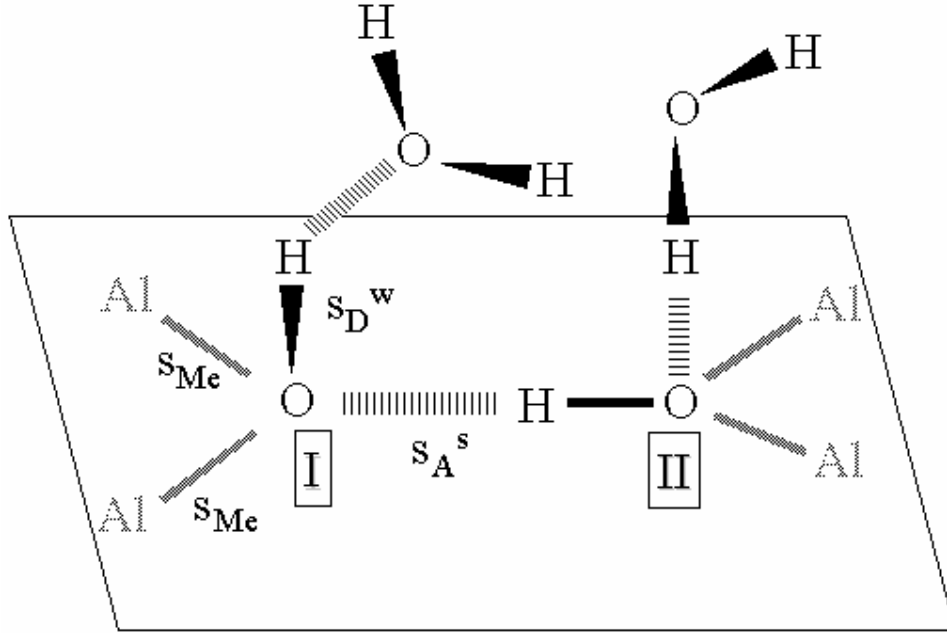
Figure IV. 11 : schématisation d'un site de surface bi-coordonné sur les faces basales de la gibbsite. Les échelles des longueurs de liaison ne sont pas respectées. I : OH 1, 2 ou 4 ; II : OH 3, 5 ou 6.
