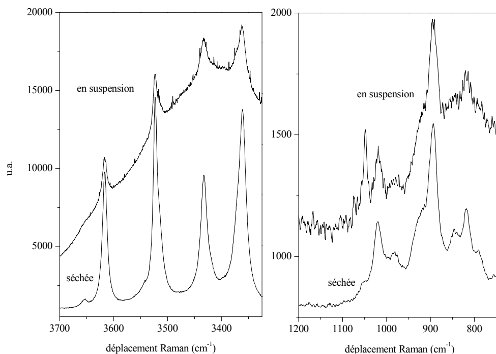
Figure IV. 21 : spectres du solide sec et en suspension dans une solution de nitrate ( [\text{NaNO}_3] = 10^{-2} \text{ M} ). Région des vibrations d'élongation O-H (à gauche) et de déformation Al-O-H (à droite).
