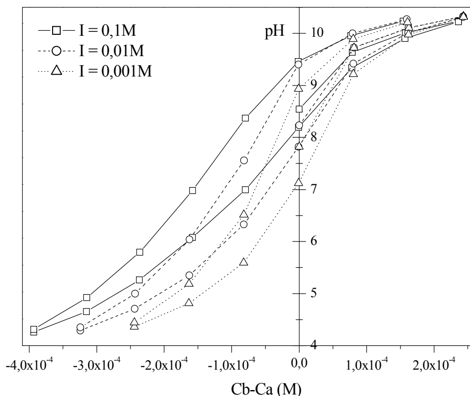
Figure IV. 9 : courbes de titrage d'un même échantillon de gibbsite à trois forces ioniques différentes ( I = 0,1 - 0,01 - 0,001 M). Gibbsite type G21, 32 g/L, intervalle de temps : 600 s, volume ajouté : 50 \mu L.
