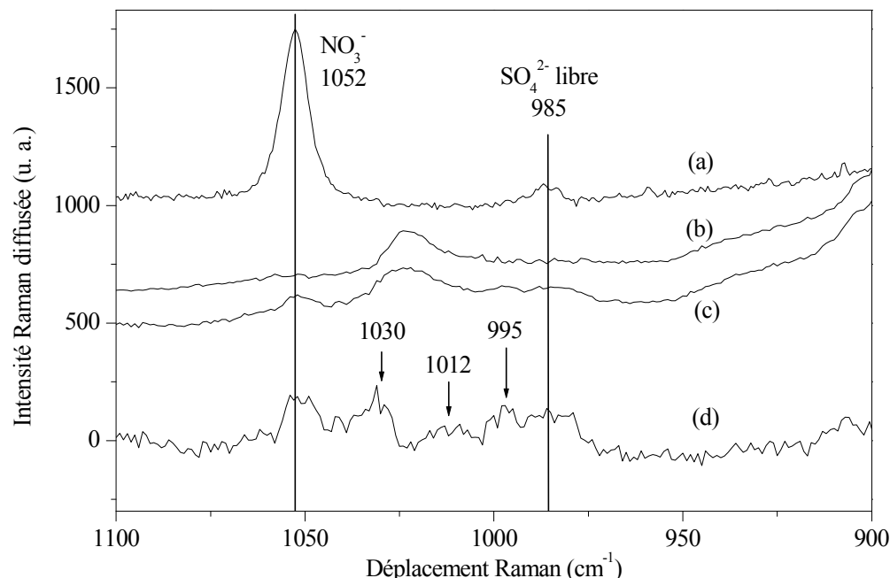
Figure IV. 25 : (a) spectre Raman d'une solution de nitrate et sulfate (respectivement 10^{-2}\text{ M} et 10^{-3}\text{ M} ) ; (b) : gibbsite type G21 in situ ; (c) : gibbsite type G21 en présence de nitrate et sulfate (3 jours) ; (d) : différence [(c)-(b)] x 3. (Rinnert, 2001)
