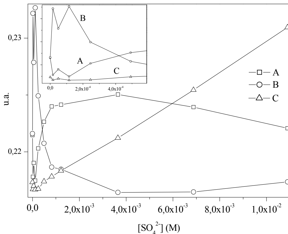
Figure IV. 20 : concentration des composantes en fonction de [\text{SO}_4^{2-}] totale ajoutée.
