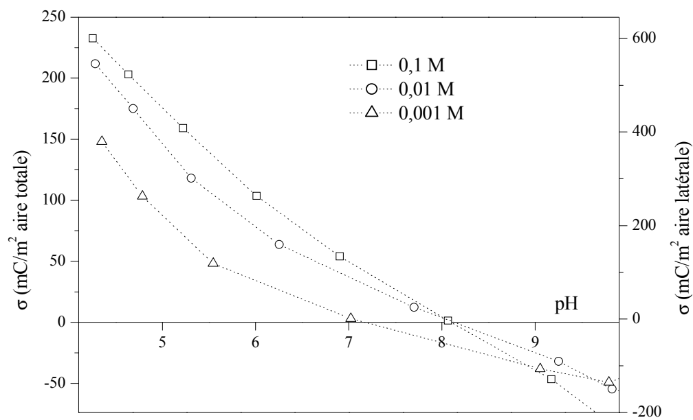
Figure IV. 10 : courbes de charge d'une suspension de gibbsite de type G21, pour trois forces ioniques, en fonction des aires spécifiques totale et latérale.
