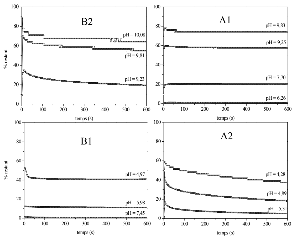
Figure IV. 8 : suivi des concentrations en \text{H}^+ ou \text{OH}^- des suspensions (en % restant par rapport à la quantité ajoutée) au cours du titrage en fonction du temps (Figure IV. ).
