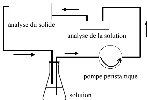
Figure E. 1 : schéma du montage pour les mesures in situ par spectrométrie Raman.
