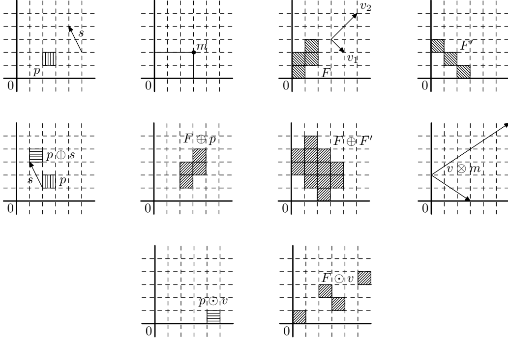
FIG. 2.9 – Opérateurs géométriques
