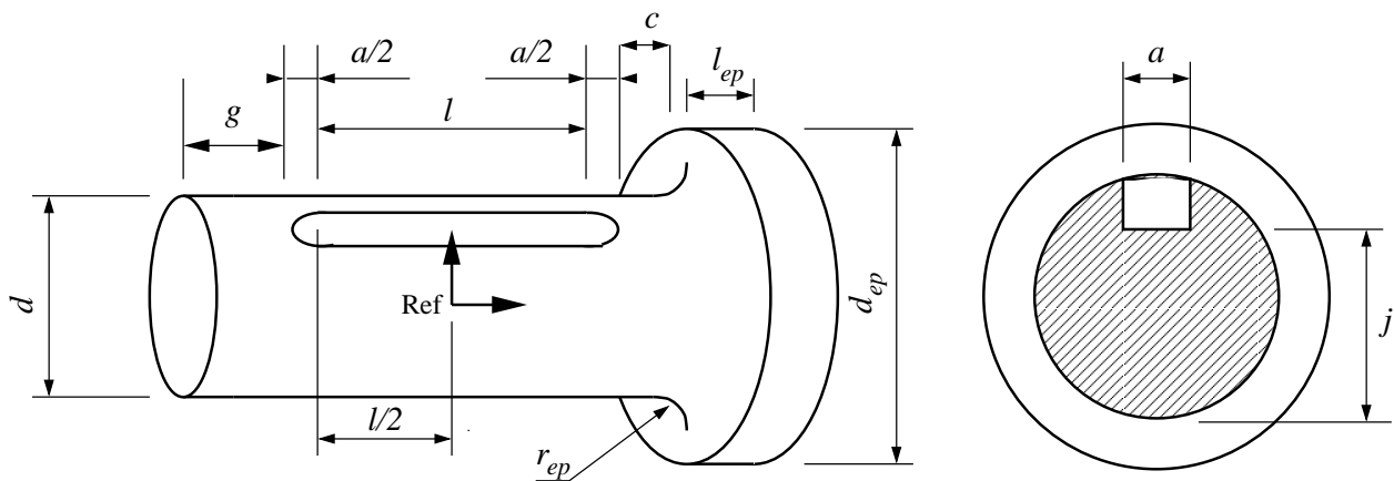
FIG. 2.22 – Exemple de paramétrage de l'arbre du DTLM.
