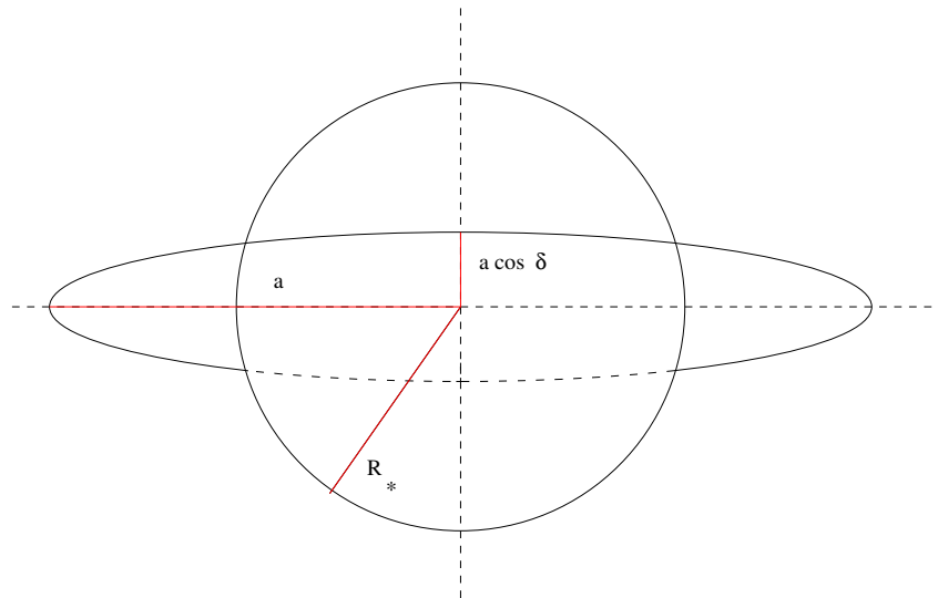
FIG. 1.2: Géométrie du transit vue de côté (a) et du point de vue de l'observateur (b). a est le demi-grand axe de l'orbite de la planète, \delta la colatitude du transit et R_* le rayon de l'étoile.
