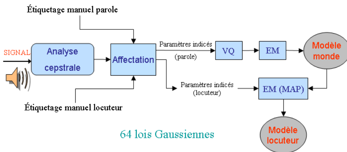
FIG. 5.4 – Procédure d'apprentissage des modèles de mélanges de lois gaussiennes correspondant au locuteur et au monde.
