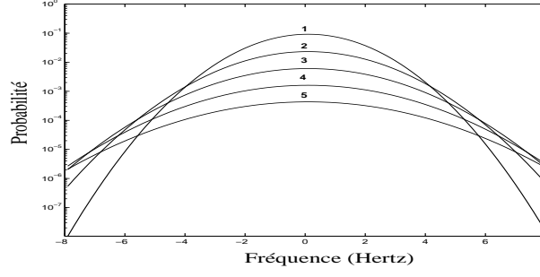
FIG. 3.8 – Représentation de \lambda_n , la probabilité associée à une n -transition entre deux pics distants d'un certain écart de fréquence, pour n \in [1, 5] . À partir d'un certain écart de fréquence (dépendant de \sigma ), il devient plus probable d'effectuer une n -transition qu'une n - 1 -transition.
