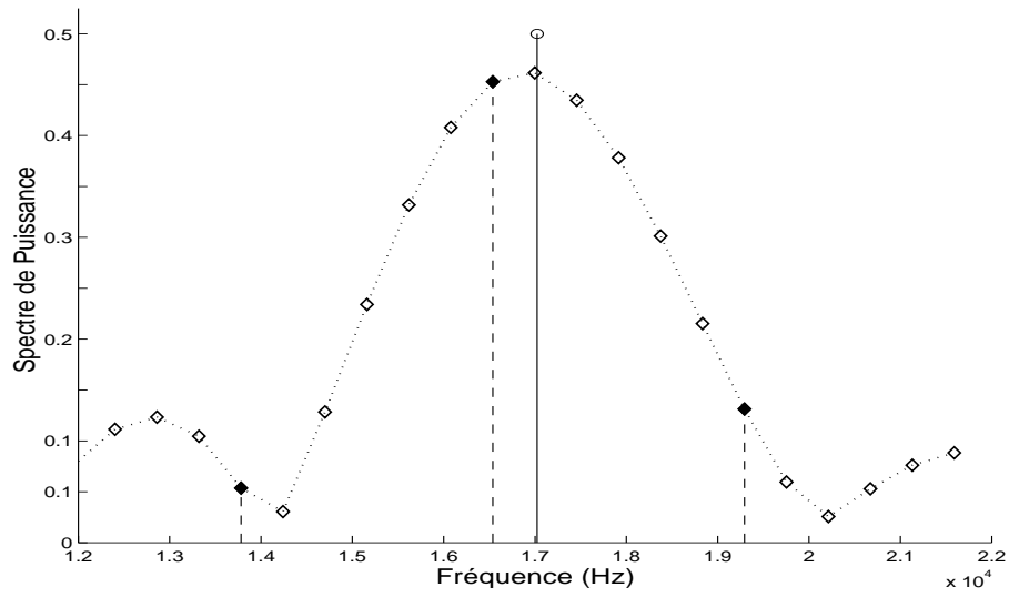
FIG. 2.7 – Sont représentées sur cette figure, la composante sinusoïdale analysée (trait plein), les composantes de la DFT (tirets) et les composantes de la DFT avec un facteur de zero-padding de 6 (diamants évidés).
