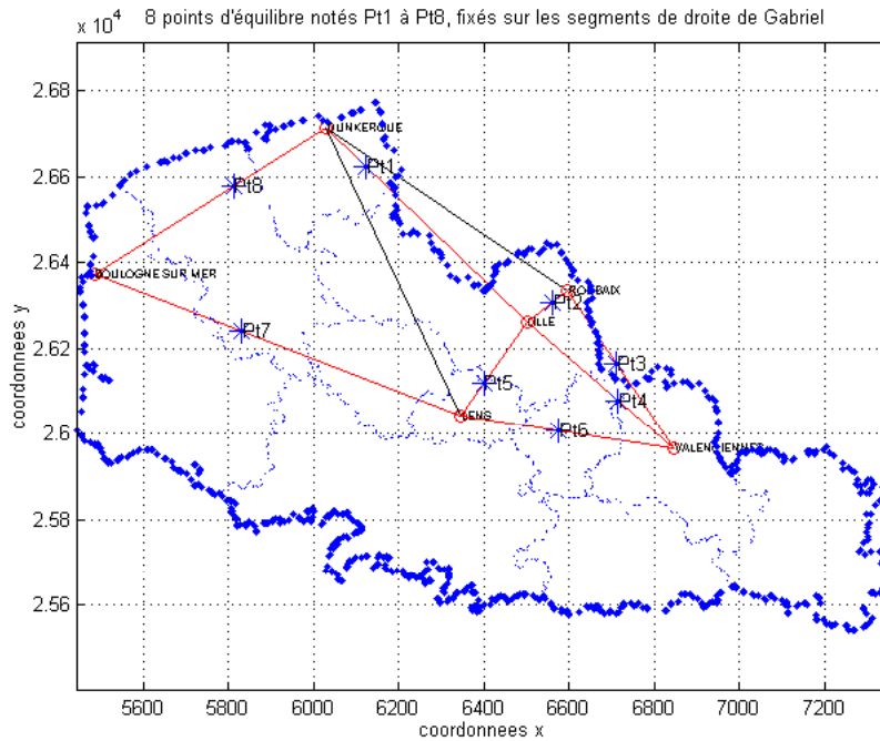
Figure 26 : tracé automatisé depuis le modèle « P » des points d'équilibre aux coordonnées barycentriques des segments de droite, positionnés uniquement sur le tracé de Gabriel.
