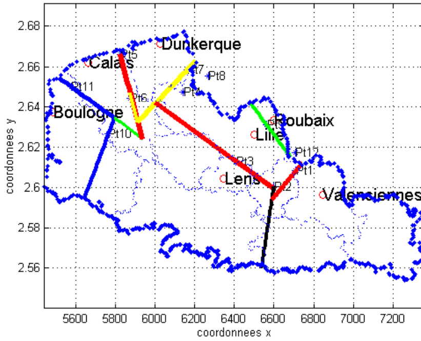
(i1-i2), (i2-i3) 12 PE - non significatifs 6,4,8,- méthode Gabriel
