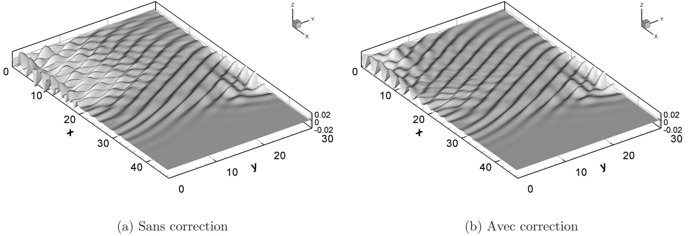
FIG. III.2.6 – Champs de vagues au second ordre après 29 périodes (Dalrymple, f = 0.55 Hz et \theta = 30 degrés)
