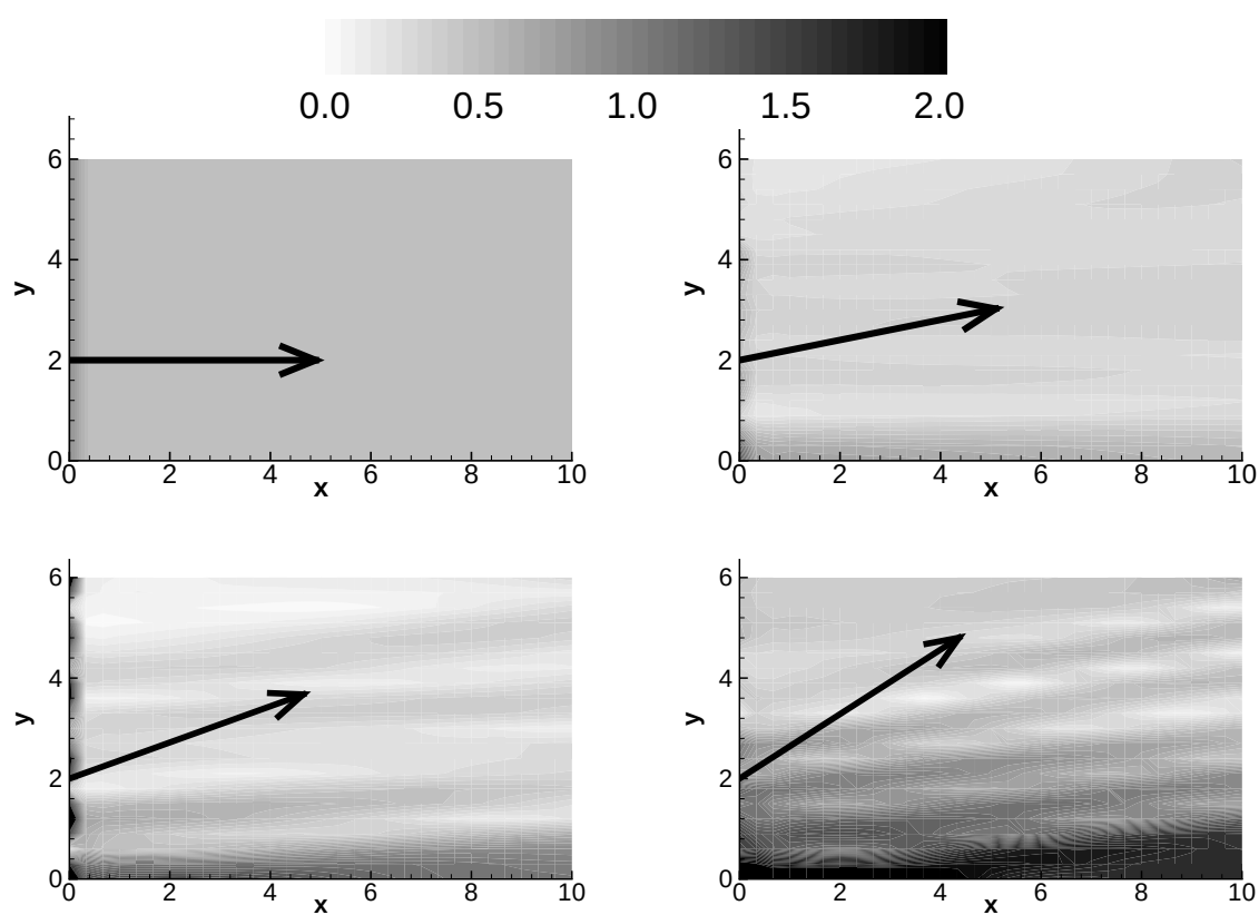
FIG. III.1.6 – Influence de la direction sur l'amplitude des ondes libres (loi de commande D'Alrymple pour f = 0.4 et \theta = 0, 10, 20 et 30 degrés)
