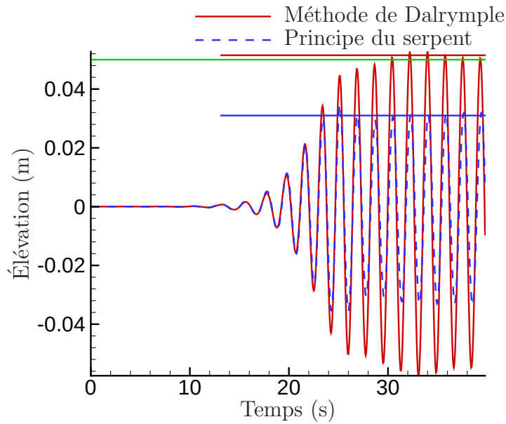
FIG. II.2.5 – Comparaison de l'élévation au point de focalisation géométrique ( \Delta\theta = 45 degrés, N = 5 ).
