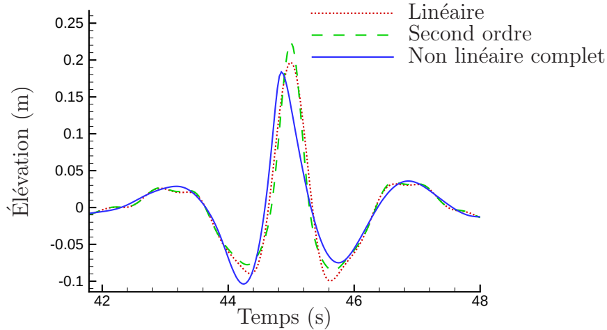
FIG. II.2.7 – Comparaison de l'élévation au point de focalisation.
