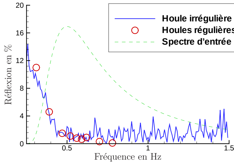
FIG. V.1.31 – Coefficient de réflexion, élévation linéaire ( T_z=1.42\text{ s} et H_s = 32\text{ cm} )
