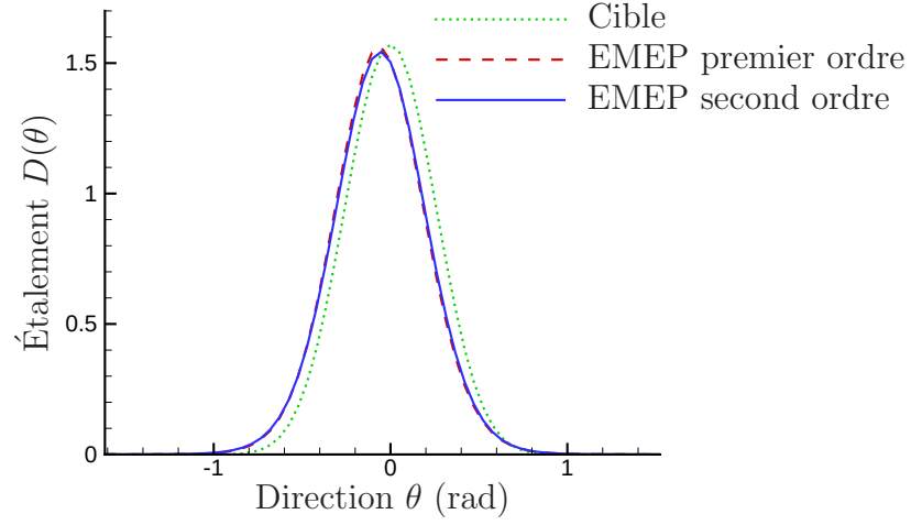
FIG. V.2.8 – Influence des non-linéarité sur l'étalement estimé (Dalrymple, f = f_p )
