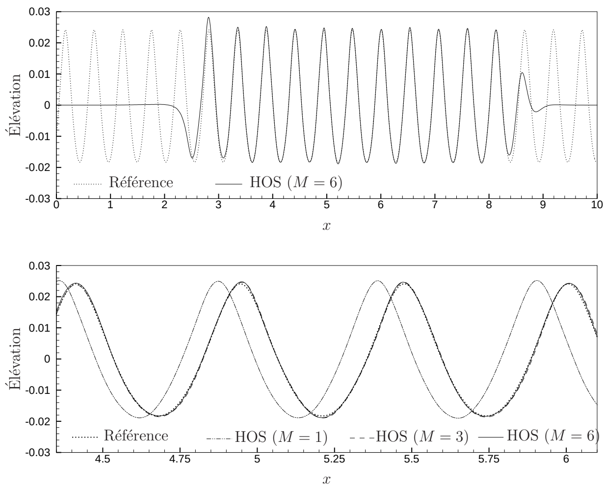
FIG. I.3.4 – Élévation de surface libre ( \varepsilon = 8 \% )
