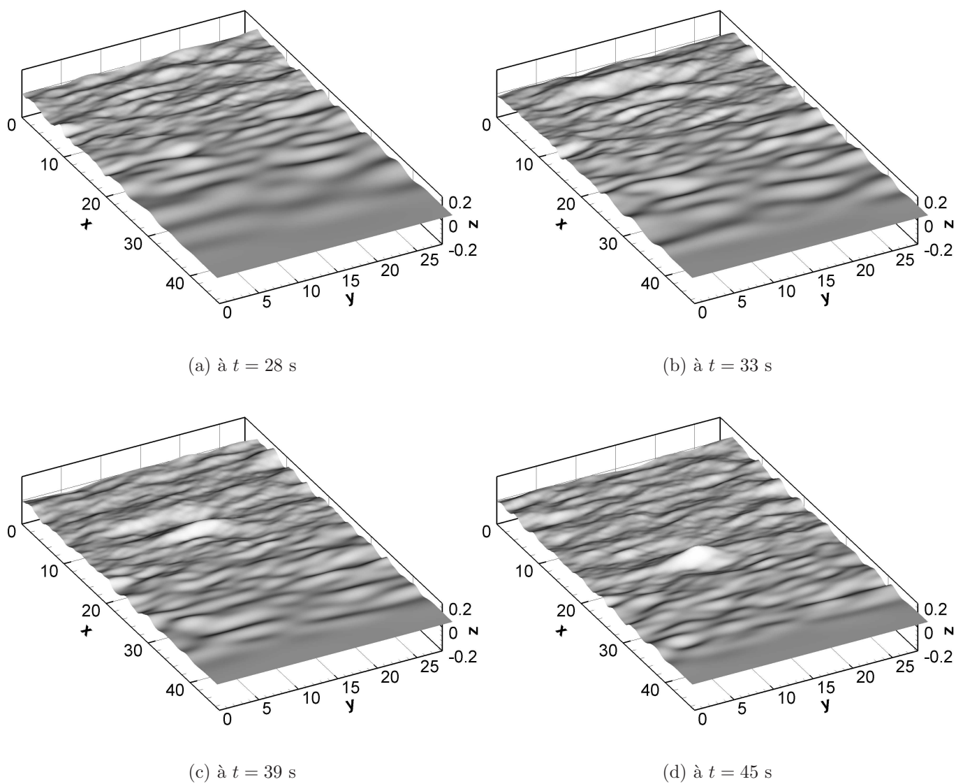
FIG. IV.1.38 – Vues du paquet de vagues reproduit (cas A).
