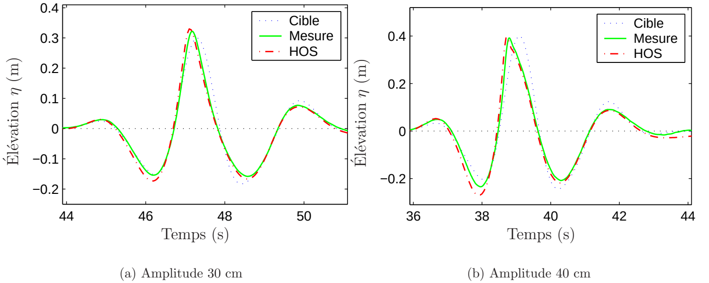
FIG. IV.1.14 – Comparaisons entre expériences et simulations HOS
