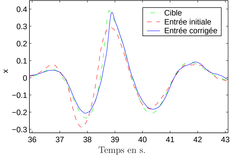
FIG. IV.1.24 – Reproduction déterministe pour un paquet de vagues d’amplitude 40 cm (décomposition initiale linéaire)
