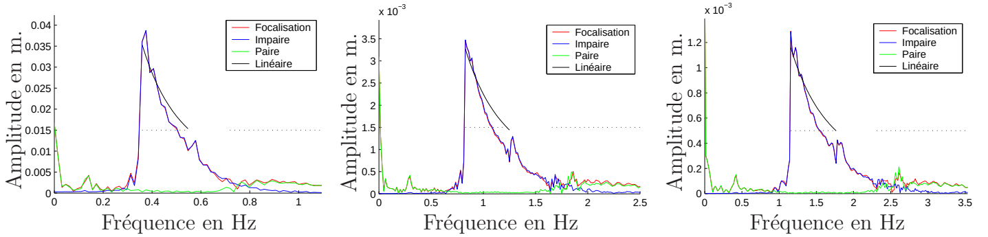
FIG. IV.1.28 – Spectre d’amplitude pour le cas Dud61 et trois facteurs d’échelle différents (de gauche à droite : 5, 1 et 0.5)
