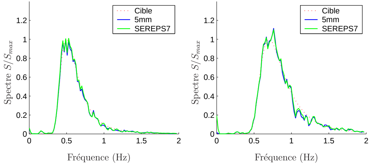
FIG. V.1.8 – Influence de la période de pic pour un état de mer doux \varepsilon_c = 3 \% (gauche : T_p = 1.4 \text{ s} , H_s = 16 \text{ cm} ; droite, T_Z = 1 \text{ s} , H_s = 8 \text{ cm} )
