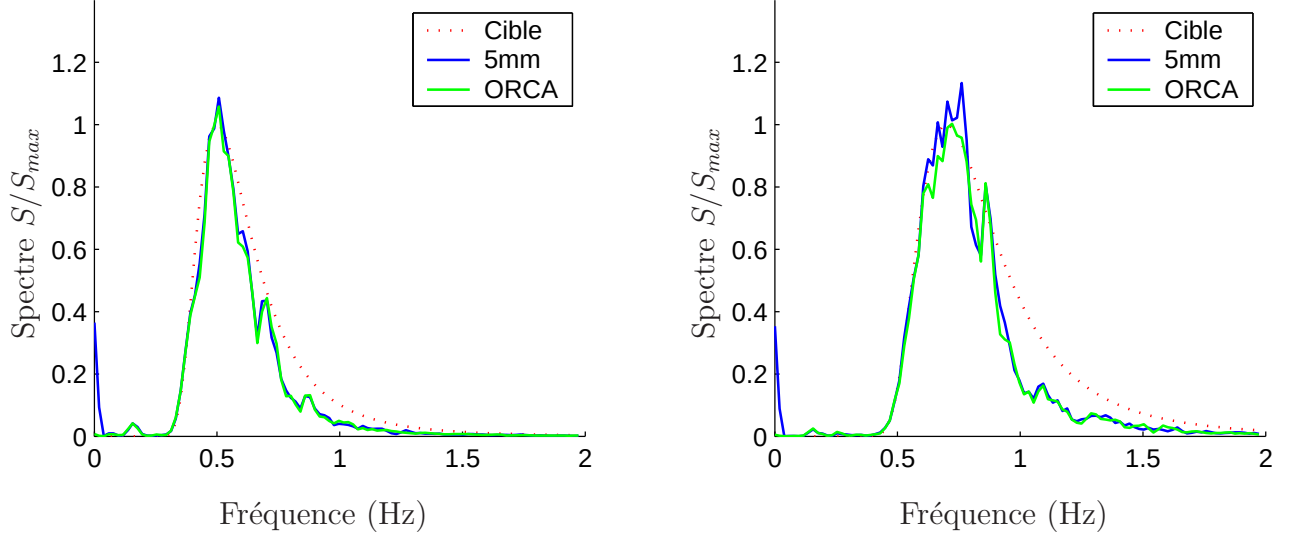
FIG. V.1.7 – Influence de la période de pic pour un état de mer sévère \varepsilon_c = 6 \% (gauche : T_Z = 1.42 \text{ s} , H_s = 32 \text{ cm} ; droite, T_Z = 1 \text{ s} , H_s = 16 \text{ cm} )
