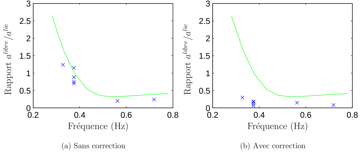
FIG. III.2.8 – Amplitude libre normalisée ( \times : expérimentale et théorique —)
