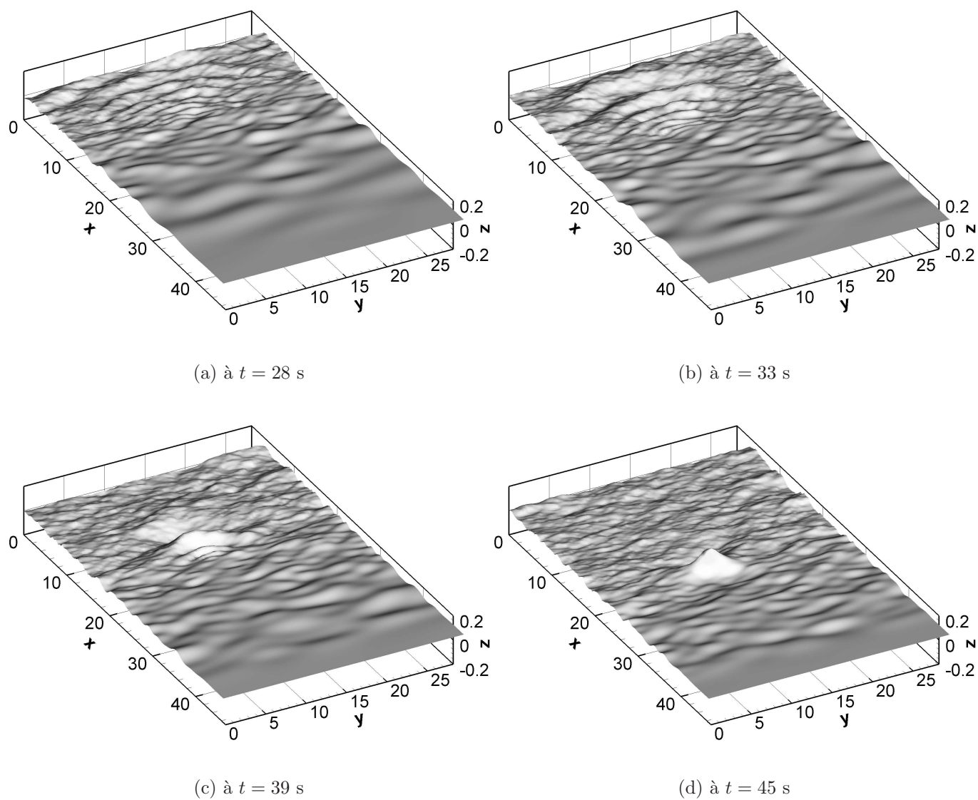
FIG. IV.1.31 – Vues du paquet de vagues cible (cas A).
