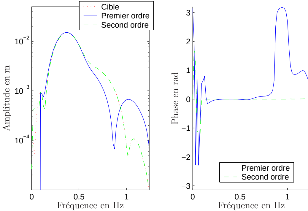
FIG. IV.1.9 – Spectre d'amplitude et de phase du mouvements du batteur (amplitude 30 cm)
