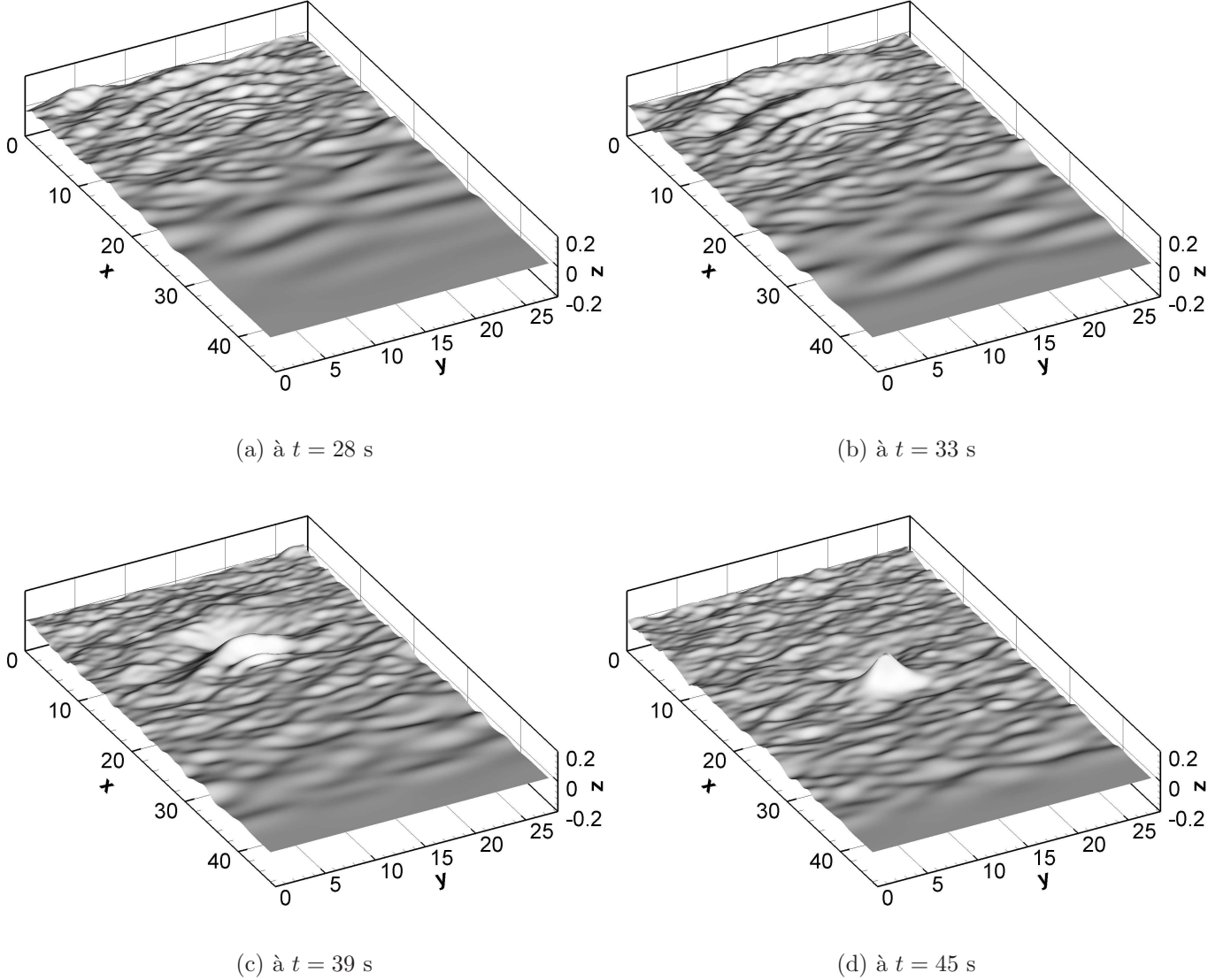
FIG. II.2.6 – Focalisation d'un spectre directionnel
