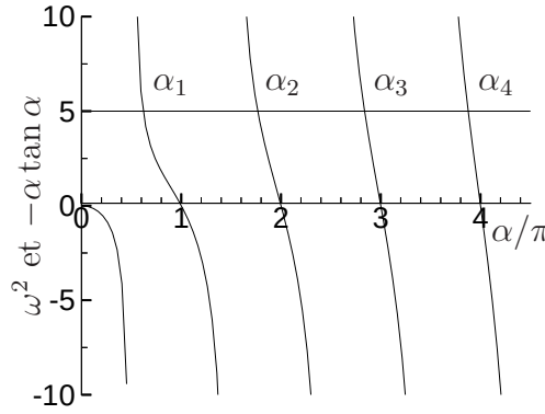
FIG. A.2 – Résolution graphique de \omega^2 = -\alpha_m \tan \alpha_m
