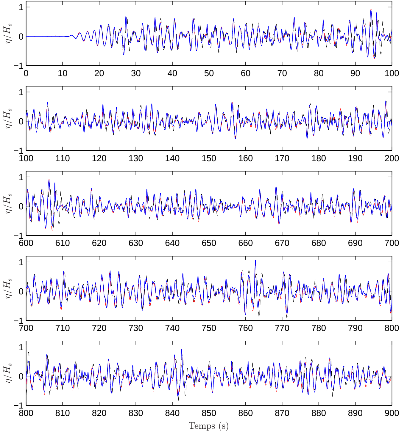
FIG. V.1.11 – Comparaison des signaux expérimental (—) numérique linéaire SWEET (---) et numérique non linéaire HOS (-.-) pour un état de mer \varepsilon_c = 3\%
