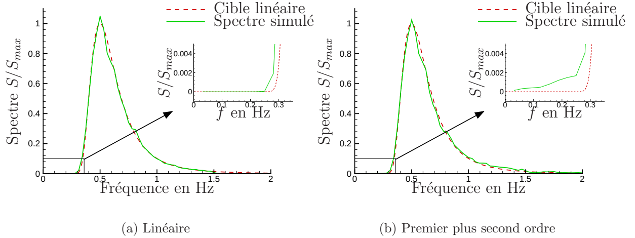
FIG. V.1.20 – Spectres des élévations simulés ( T_Z=1.42 s et H_s = 32 cm)
