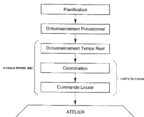
FIG. 1.2 – structure décisionnelle à cinq niveaux pour un atelier flexible
