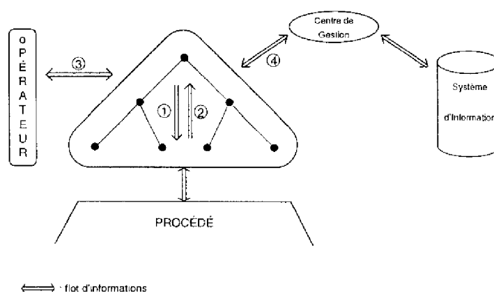
FIG. 1.1 -- les flots d'informations dans le système de surveillance-commande
