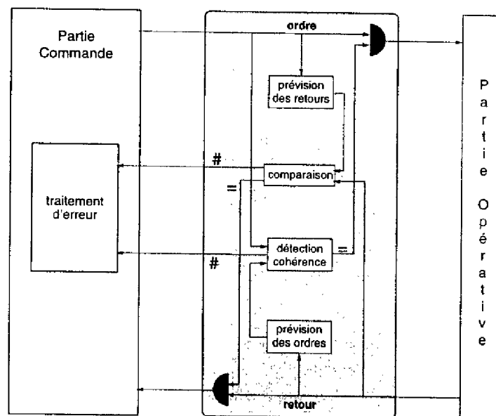
FIG. 2.2 – utilisation du modèle en filtre : émulation du comportement
