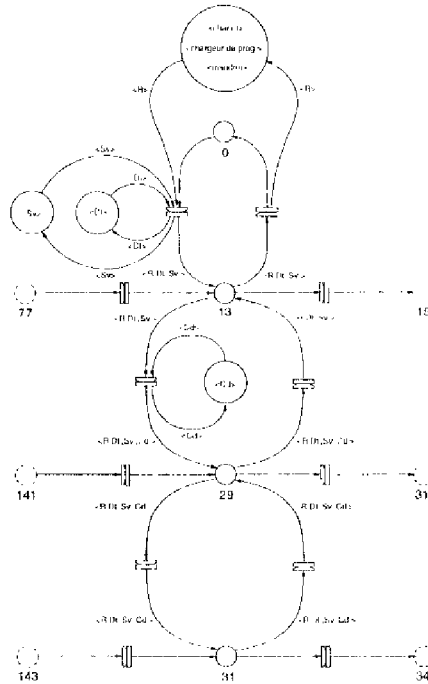
FIG. 1.4 – extrait du réseau de référence du module Tour
