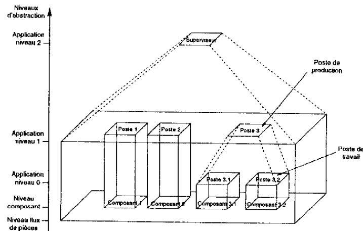
FIG. 2.5 – exemple de modélisation d'une cellule basée sur le MESAP
