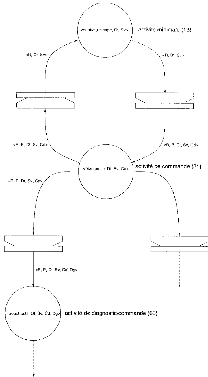
FIG. 3.6 – exemple de réseau de surveillance-commande
