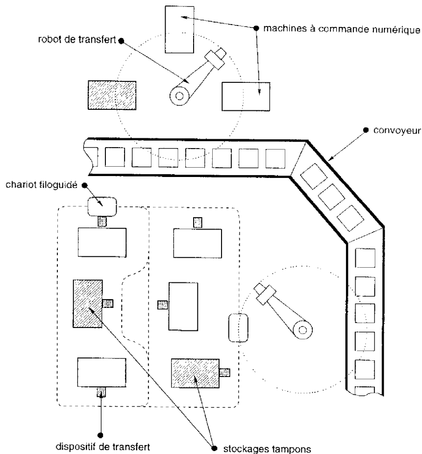
FIG. 1.1 – exemple d'un atelier flexible
