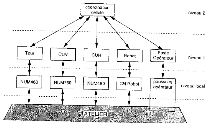
FIG. 1.3 – structure de surveillance-commande
