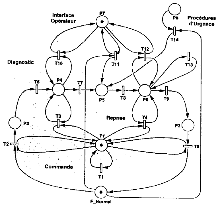
FIG. 3.3 - traitement global de surveillance
