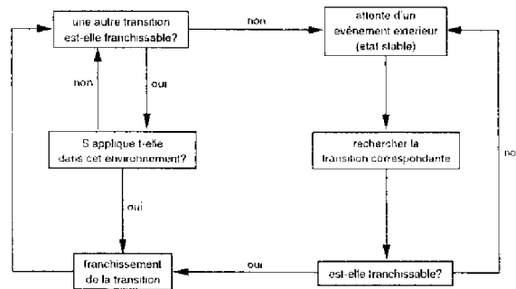
FIG. 3.9 – mécanisme d'un joueur de réseau de Petri
