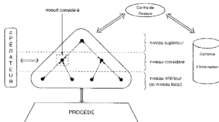
FIG. 2.1 - vue globale de l'architecture de surveillance-commande
