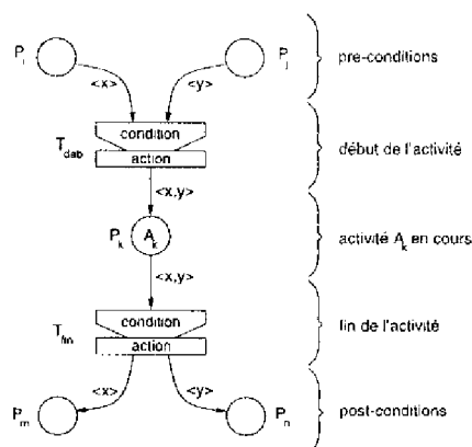
FIG. 3.2 – activité de commande modélisée par RdPO
