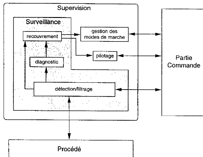
FIG. 2.4 - vue partielle du modèle fonctionnel de la supervision
