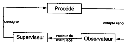
FIG. 2.8 – retour d'état par utilisation d'un observateur
