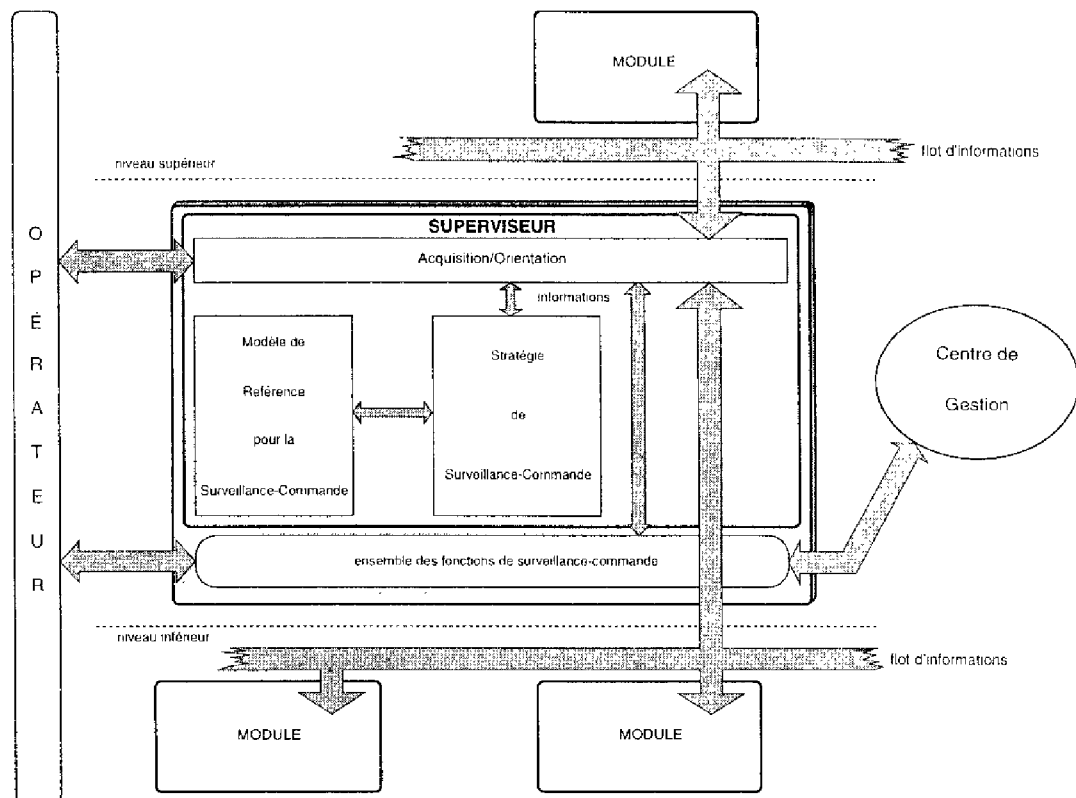
FIG. 3.1 – structure d'un nœud (module) de surveillance-commande
