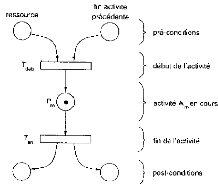
FIG. 1.6 – modélisation par réseaux de Petri d'une activité de commande
