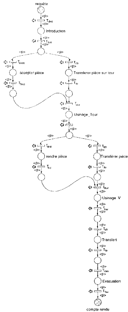
FIG. 2.2 - séquence de commande du module Coordination
