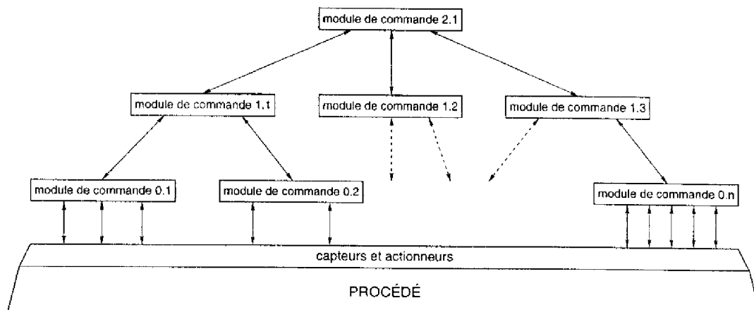
FIG. 1.4 – structure hiérarchique et modulaire de la commande temps réel
