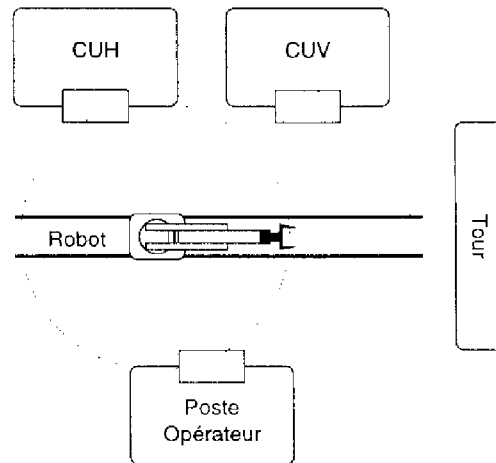
FIG. 1.1 disposition au sol des éléments de la cellule flexible
