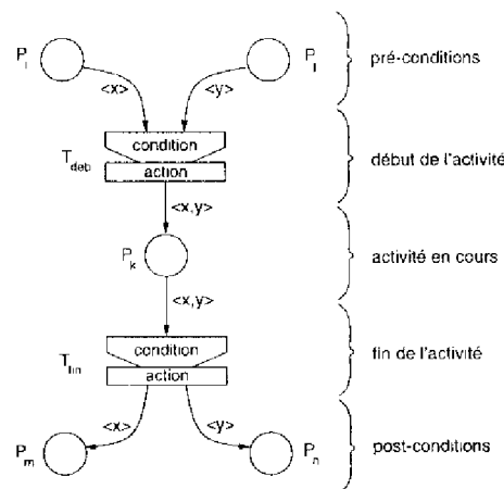
FIG. 3.5 – modélisation par RdPO d'une activité
