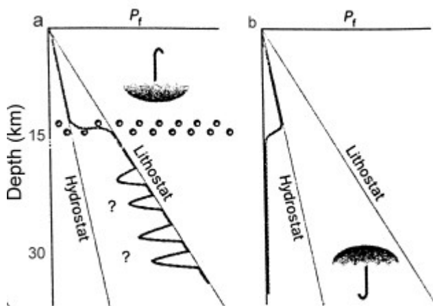
Figure I.10 : Modèles conceptuels d'évolution profondeur-pression des fluides ( P_f ) dans une croûte continentale stable, d'après Yardley & Valley (1994). a) Une phase fluide continue est présente en partie ou en totalité dans la croûte ductile (modèle de Bailey, 1994). b) Les fluides sont présents uniquement dans la croûte cassante, et la croûte ductile est sèche, les fluides étant présent localement sous forme d'inclusions isolées. Les parapluies donnent le sens des transferts des flux prédits par les deux modèles.
