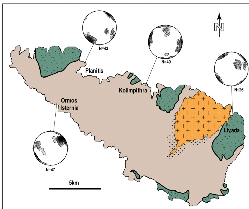
Figure III.17: Stéréogrammes montrant la direction des pôles des veines V3 dans les unités inférieure et supérieure (sans débasculement, Schmidt, hémisphère inférieure). En plus de la direction principale N100 à N135, une direction perpendiculaire N015 à N45 est observable au NE du dôme.
