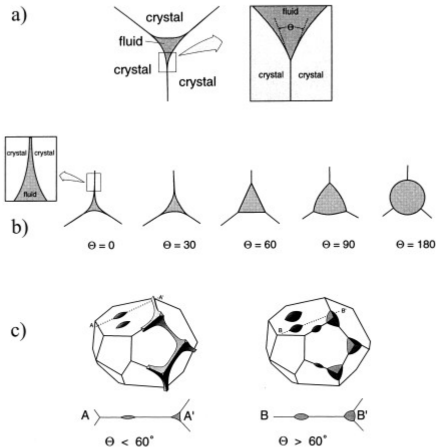
Figure I.9 : Angle diédral des pores dans une texture d'équilibre, d'après Watson & Brenan (1987). a) Section d'un pore saturé ou d'un chenal entre deux pores saturés, en texture d'équilibre, à la jonction de trois grains. L'angle diédral ( \theta ) est représenté dans l'encadré, à droite. b) Section d'un pore ou d'un chenal à différentes valeurs de \theta . c) Perspective illustrant la distribution des fluides (grisé) autour d'un grain unique pour des valeurs de \theta inférieures à 60^\circ (à gauche) et supérieures à 60^\circ (à droite). A gauche, les pores sont interconnectés par un réseau de chenaux. A droite, les pores sont isolés aux sommets du grain. Les coupes A-A' et B-B', localisées par des lignes pointillées, sont perpendiculaires à la surface du grain.
