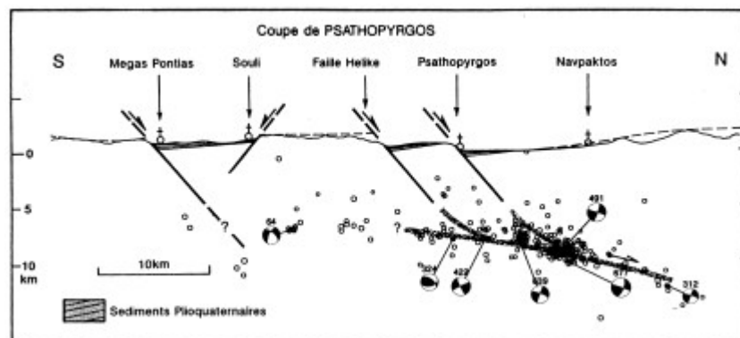
Figure II.5 : Micro-sismicité dans le golfe de Corinthe entre Juillet et Août 1991, d'après Rigo (1994). Sur une coupe Nord-Sud, les microséismes sont répartis le long d'un plan à faible pendage vers le Nord, entre 10 et 12 km de profondeur. Les essaims sont dans le prolongement des grandes failles normales à fort pendage de la région.
