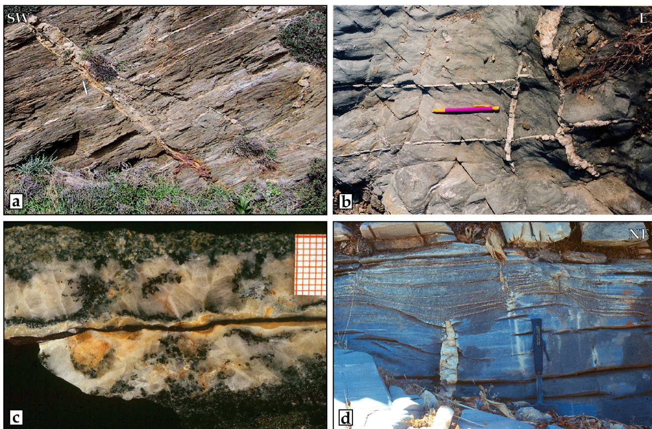
Figure III.16: a) Veines V3 à oxydes orientées N135 sur le flanc SW du dôme. b) Deux directions perpendiculaires de veines V3 N100 et N015 sur le flanc NE. Les V3 N100 intersectent les V3 N15 avec une composante décrochante sénestre. c) Zonation syntaxiale des V3. Des épontes vers le centre: Albite-chlorite; calcite; chlorite; calcite micritique; oxydes de fer. d) V3 dans les marbres du toit de la dolomie. La veine recoupe les plans de cisaillement ductile à vergence NE. Localisation Fig. III.10.
