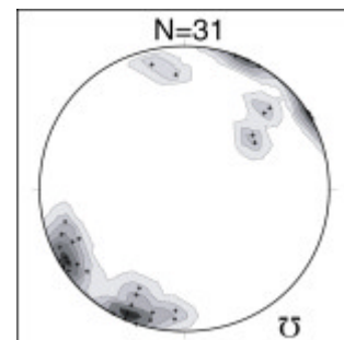
Figure VII.4 : Pôles des V2b tardifs (Planitis, plans débaisculés de la foliation).
