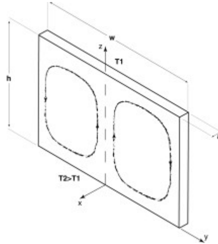
Figure I.18 : Géométrie des cellules de convections dans une fracture verticale d'après Murphy (1979).
