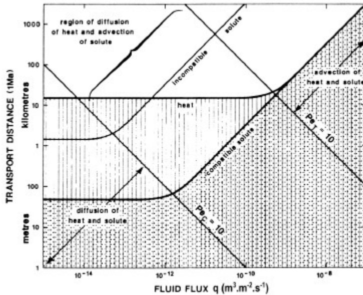
Figure 1.3 : Distance de transport en 1 Ma de la chaleur, d'un élément "compatible" (c'est-à-dire présent dans les phases fluide (fl) et solide (r) tel que C_r.r_r/C_\beta.r_\beta = 1 , C étant la concentration de l'élément et r la densité de la phase), et d'un élément "incompatible" (absent dans la roche), en fonction du flux de matière q calculé avec une porosité de 0.1 %. La courbe de l'élément compatible est celle de l'oxygène, avec une diffusivité efficace D = 10^{-11} \text{ m}^2/\text{s} . Conductivité thermique K_m = 10^{-6} \text{ m}^2/\text{s} . La surface délimitée par des points noirs est la région de transport de l'élément compatible (ici l'oxygène). Les traits verticaux donnent la région de transport de chaleur (d'après Bickle & McKenzie, 1987).
