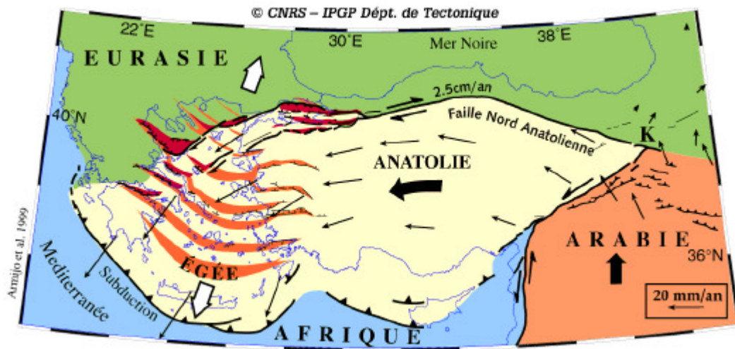
Figure III. 3 : Cadre géodynamique actuel de l'Anatolie d'après Armijo et al. (1999). L'étalement de la région égéenne vers le front de subduction hellénique (au Sud) se traduit par une rotation anti-horaire à l'Ouest de l'Egée, et une rotation horaire à l'est, conformément au modèle de Taymaz et al. (1991).
