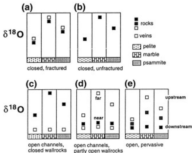
Figure I.4 : Schémas d'altération isotopique ou chimique d'une roche sujette aux différents types d'interaction fluide/roche d'après Oliver (1996). L'élément pris comme exemple est l'oxygène. Les compositions isotopiques de la roche et des veines métamorphiques sont représentées. De a) à e) les signatures isotopiques reflètent un degré et une distance d'équilibration croissant entre la roche et le fluide. Les Figures a) b) et c) sont théoriquement indépendantes de l'échelle, mais l'observation de ces phénomènes est généralement faite à l'échelle mésoscopique. d) est surtout observée aux échelles méso- et macroscopiques. e) est surtout vrai à l'échelle macroscopique.
