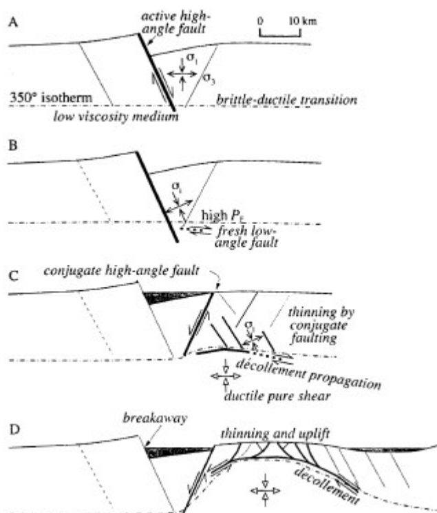
Figure II.6 : Modèle de formation d'un détachement par rotation des contraintes le long d'une faille à faible coefficient de friction, d'après Chéry (2001). L'évolution d'un dôme métamorphique se résume en quatre stades. A) Stade demi-graben, l'orientation des contraintes n'est pas perturbée car le coefficient de la friction de la faille est élevé. B) Stade "golfe de Corinthe" : la pression de pore P_f élevée diminue le coefficient de friction, ce qui induit une rotation de la contrainte principale majeure s_1 parallèlement au plan de rupture. Une faille à faible pendage se forme. C) Propagation du détachement : la croûte supérieure est amincie par le jeu de faille normale dans le compartiment supérieur. D) Stade "Snake Range" : dans le cadre d'une extension rapide, le mur du détachement développe une structure anticlinale par isostasie. Le détachement joue à faible profondeur (0-4 km). La température n'est rééquilibrée qu'après la fin de l'extension.
