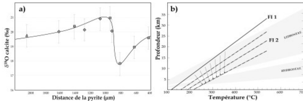
Figure VII.6 : a) \delta^{18}\text{O} des grains de calcite dans l'ombre de pression en fonction de la distance du porphyroblaste de pyrite. b) Fluctuation des isochores de stabilité dans l'ombre de pression. Les isochores les plus basses correspondent aux inclusions les plus tardives.
