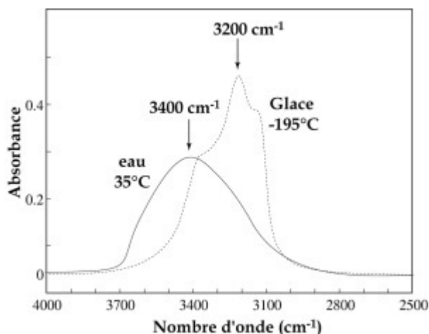
Figure VI.2 : (à droite) Variation de la position du spectre IR de l'eau pure en fonction de la température (figure de Aines & Rossman, 1984 , d'après les données de Eisenberg & Kauzmann, 1962). Le pic apparent de la glace à -195 °C est à 3200 \text{cm}^{-1} . Le pic apparent de l'eau liquide à 35 °C est à 3400 \text{cm}^{-1} .
