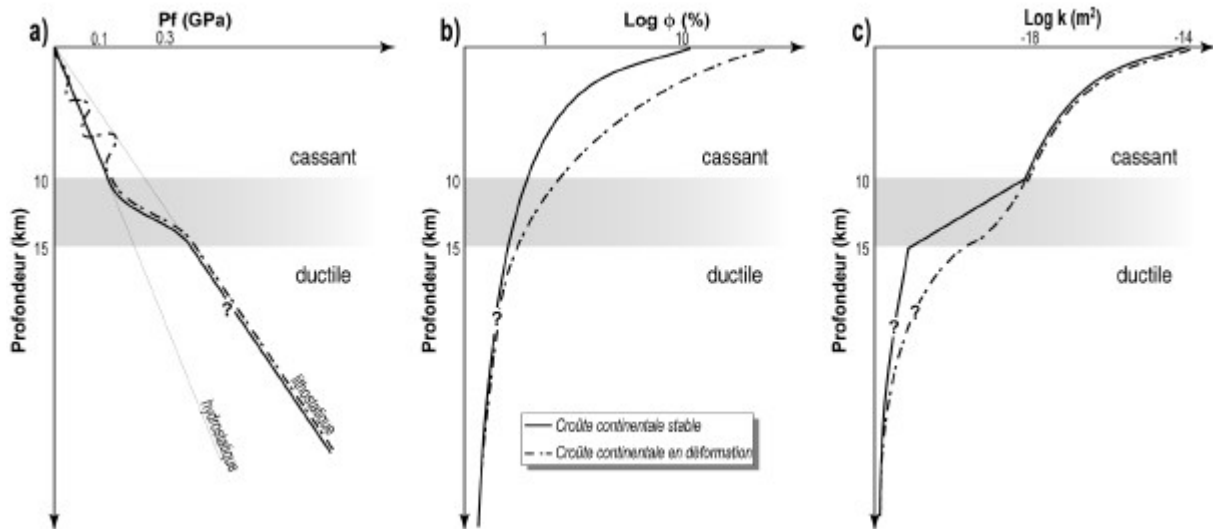
: a), b) et c) Profils synthétiques de pression des fluides ( P_f ), de porosité ( \phi ) et de perméabilité ( k ), respectivement, de la croûte continentale en fonction de la profondeur. Traits pleins : croûte stable. Tirets : croûte déformée. Les points d'interrogation soulignent les zones où aucune donnée n'est disponible. Voir texte pour justification.
