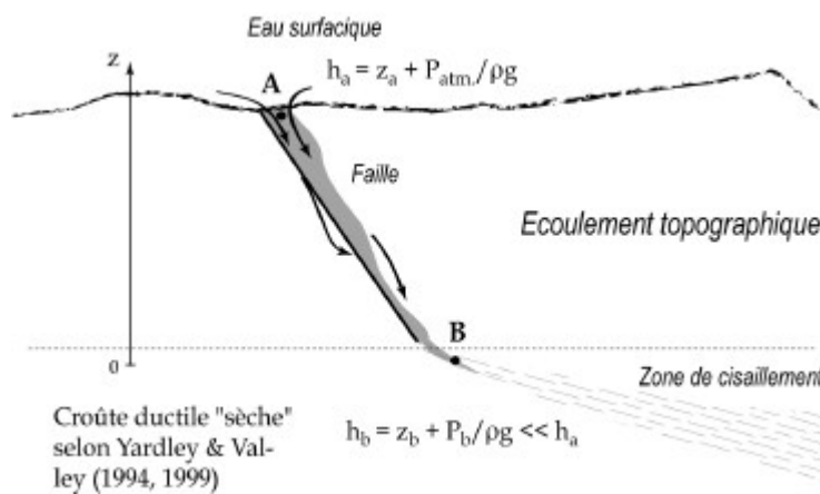
Figure I. 15 : Ecoulement topographique le long d'une faille vers une zone de cisaillement. L'eau se dirige vers la charge hydraulique la plus faible. C'est B qui a la charge la plus faible, selon l'hypothèse d'une croûte inférieure sèche de Yardley & Valley (1994,1999).
