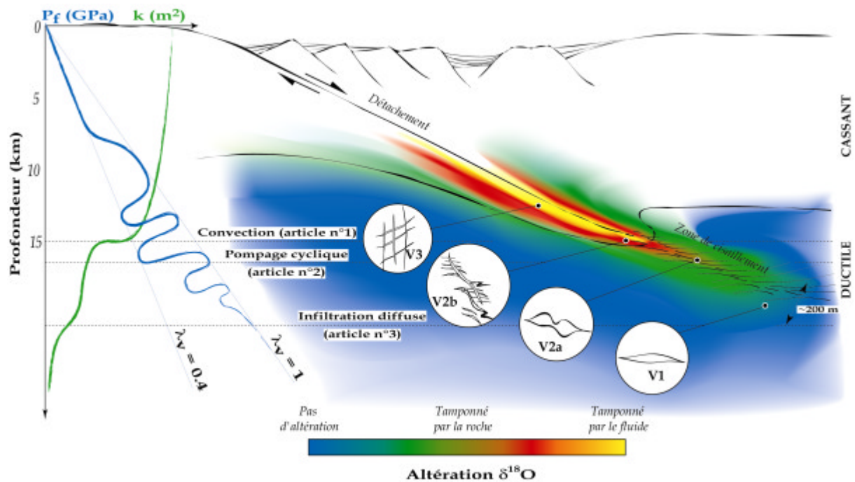
Figure VII.7 : Synthèse des interprétations montrant l'étagement des mécanismes de circulation, ainsi que les profils de pression et de perméabilité en fonction de la profondeur. L'épaisseur de la frange d'altération isotopique ne respecte pas l'échelle horizontale.
