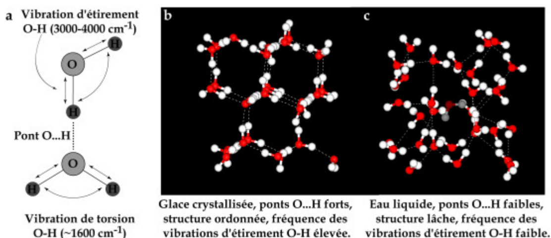
Figure VI.3 : (ci-dessous) Structures des molécules d'eau. a) Vibrations de la molécule d'eau dans l'infrarouge. La vibration d'étirement est celle qui produit un spectre dans la gamme 3000-4000 \text{cm}^{-1} . Le pont O...H est engendré par les forces d'attraction \text{O} \cdots \text{H}^+ . La distance des ponts O...H influe sur la fréquence de vibration d'étirement O-H. b) et c) modèles structuraux de l'agencement des molécules d'eau à l'état liquide et à l'état cristallisé (image obtenue sur le site http://www.sbu.ac.uk/water/index.html ).
