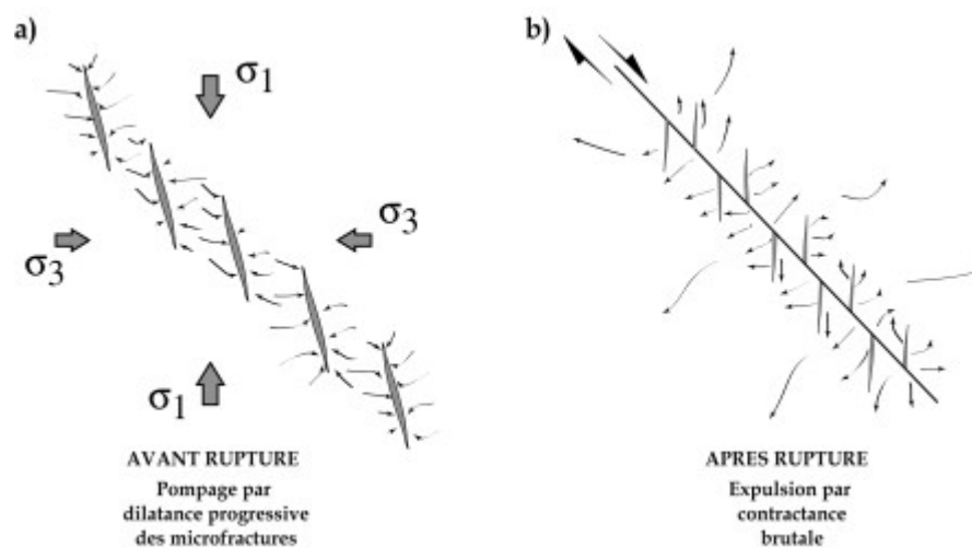
Figure 1.16 : Mouvement de fluides par dilatance-contractance au cours des cycles sismiques. a) Avant fracturation lors de l'accumulation progressive des contraintes. b) Après rupture, lors du relâchement brutal des contraintes.
