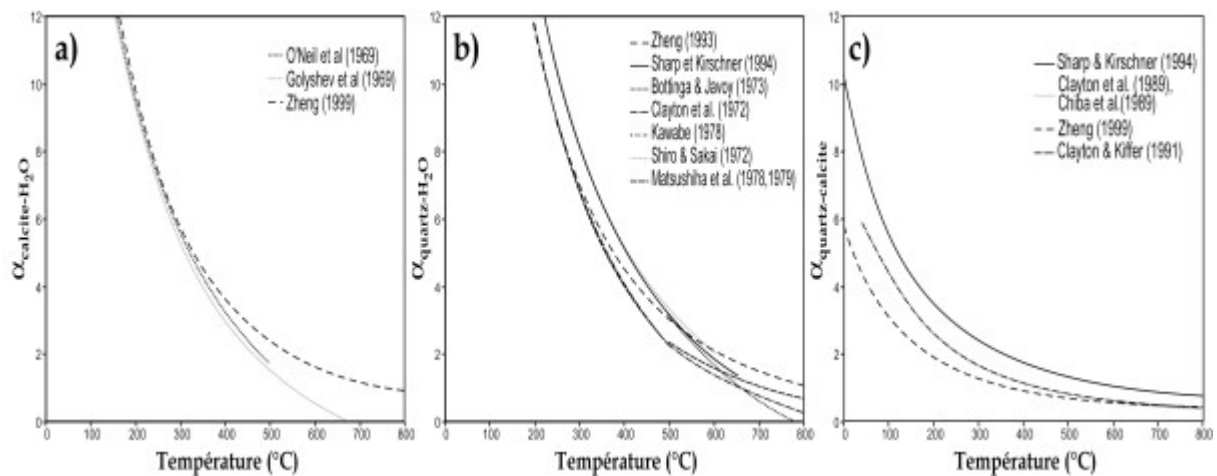
Figure IV.1 : Calibration des équations de fractionnement en fonction de la température. a) Couple calcite-H 2 O. b) Couple quartz-H 2 O. c) Couple quartz-calcite.
