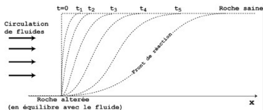
Figure I.1 : Schéma d'évolution chromatographique d'une réaction chimique ou isotopique entre le fluide en circulation et la roche encaissante. La forme du front de réaction est liée à la quantité de fluides ayant circulé.
