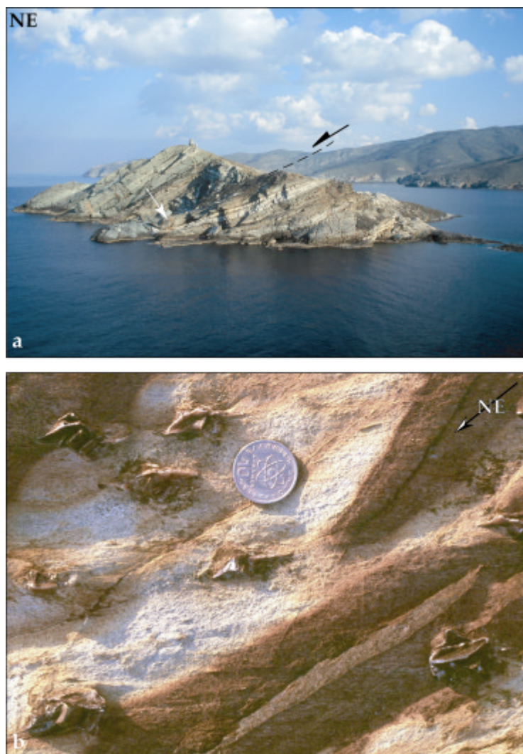
Figure V.2 : a) Détachement de Planitis, entre les alternances volcano-sédimentaires de l'unité inférieure et les metabasites de l'unité supérieure. La flèche blanche marque le lieu d'échantillonnage. b) Porphyro-blastes de pyrite avec ombres de pression à quartz-calcite dans les ultramylonites qui bordent le contact.
