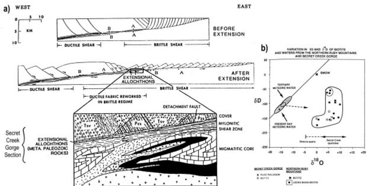
Figure II.9 : a) Coupe schématique du dôme métamorphique de la East Humbolt Range (Ruby Mountains), illustrant l'évolution tectonique du mur du détachement au cours de l'extension Tertiaire, depuis la déformation ductile vers la déformation cassante. La coupe de la gorge de Secret Creek est agrandie. b) Valeurs du \delta^{18}O et du \delta D de biotites échantillonnées dans des quartzites, sur une coupe Est-Ouest allant vers le détachement, du Lizzies Basin à Secret Creek. Les données définissent une trajectoire d'échange isotopique croissant avec une eau surfacique, depuis les roches magmatiques vierges (biotites du Lizzies Basin) jusqu'aux mylonites, puis aux brèches à quartz ( \delta^{18}O \sim 0 ‰, \delta D \sim -160 ‰). A 500 °C, les échantillons les biotites les plus altérées seraient en équilibre avec une eau à \delta^{18}O \sim 5 ‰ et \delta D \sim -120 ‰ (d'après Fricke et al. 1992).
