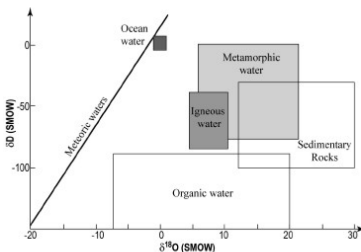
Figure II.8 : Classification des eaux en fonction de leur composition en isotopes de l'oxygène ( \delta^{18}\text{O} ) et de l'hydrogène ( \delta\text{D} ), par rapport aux eaux océaniques (SMOW), modifiée d'après Sheppard (1986).
