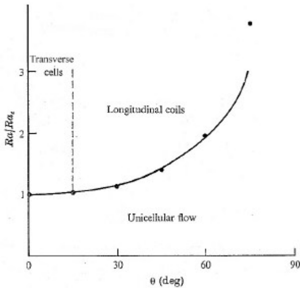
Figure A5.1 : Géométrie des cellules de convection en fonction du rapport Ra/Ra_{\text{critique}} et de l'inclinaison de l'horizon perméable, d'après Bories & Combarnous (1973). Trait noir : relation théorique. Points noirs : données expérimentales.
