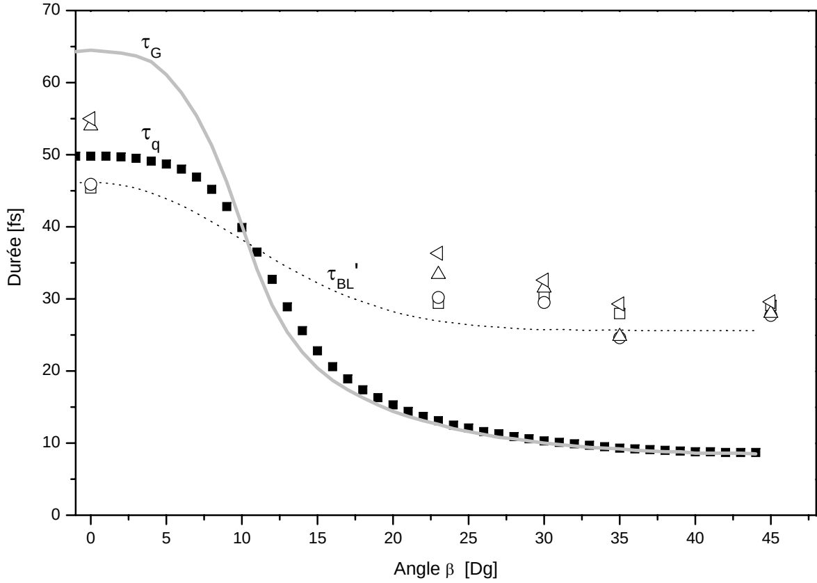
Fig. II.37 : Largeur à mi-hauteur des bandes latérales expérimentales de 14 à 20 en fonction de l'angle \beta (respectivement \square , \circ , \triangle , \diamond ). La largeur de la porte d'ellipticité \tau_G est représentée (trait gris) ainsi que la largeur à mi-hauteur de l'émission harmonique ( \blacksquare ) et enfin la largeur de la fonction d'inter-corrélation attendue (trait noir pointillé).
