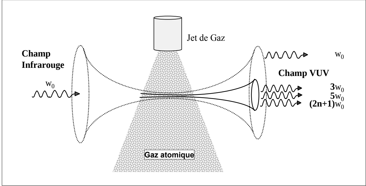
Fig. I.2 : Principe schématique de la génération d'harmoniques d'ordres élevés.
