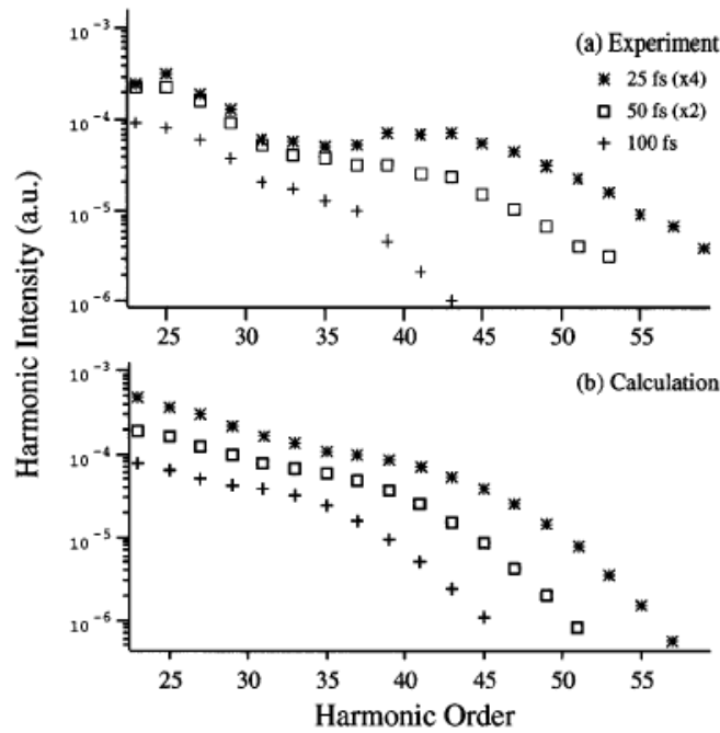
Fig. I.21 : (a) Harmoniques générées dans l'argon par une impulsion de durée proche de la limite de fourier de 25 fs (*), 50 fs (□) et 100 fs (+) avec une intensité de 4 \times 10^{14} \text{ W/cm}^2 . La cellule de gaz de longueur 1 mm est placée 2,5 cm après le foyer. D'après [Christov et al. 96].
