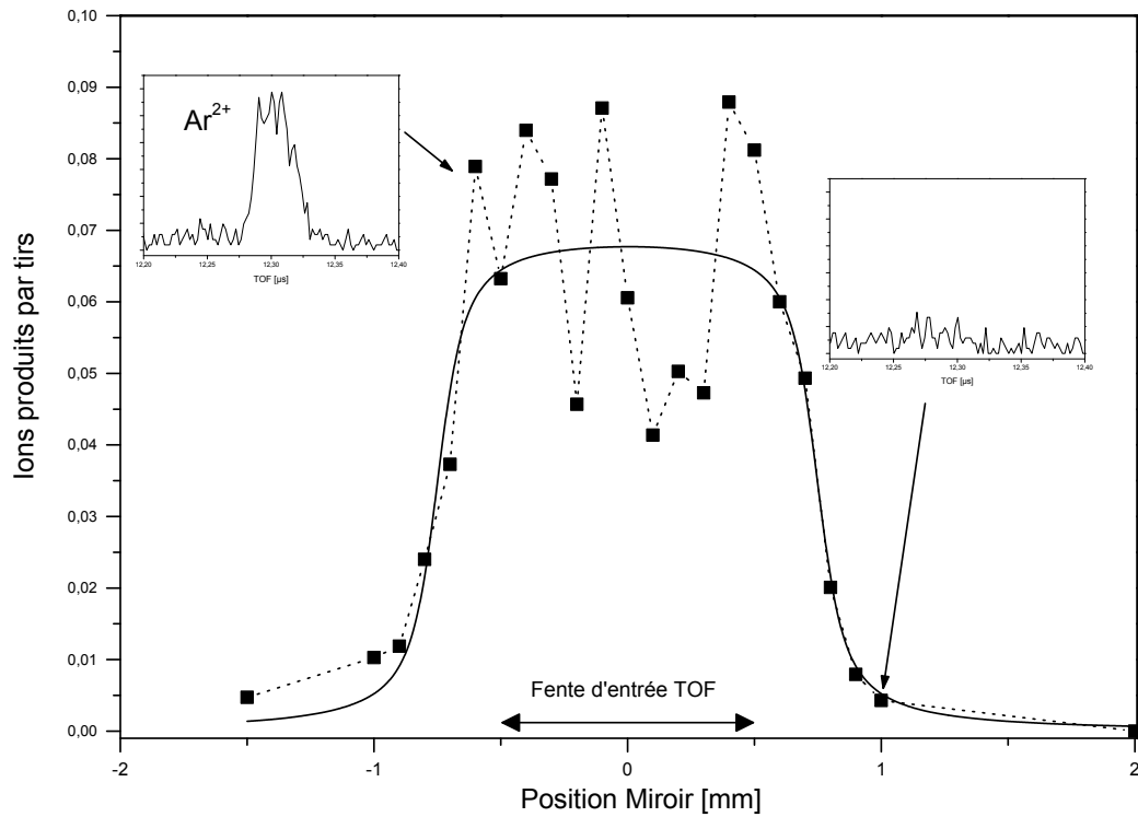
Fig. III.24 : Nombre d'ions \text{Ar}^{2+} détectés en fonction du déplacement longitudinal du miroir en platine. Les points expérimentaux (en pointillé) sont mesurés sous les conditions suivantes : La pression dans la zone sensible est P(\text{Ar})=8.10^{-5} mbar. La pression dans la cellule remplie de xénon est P(\text{Xe})=9 mbar. Énergie incidente dans la cellule E=2,6 mJ. La courbe théorique définie par la formule III.21 et donnant le meilleur ajustement est en trait plein.
