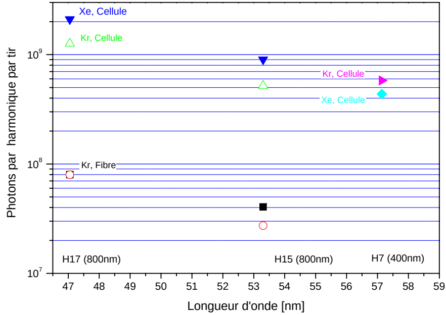
Fig. I.34 : Nombre de photons par harmonique en fonction de la longueur d'onde des harmoniques pour différents dispositifs expérimentaux:
