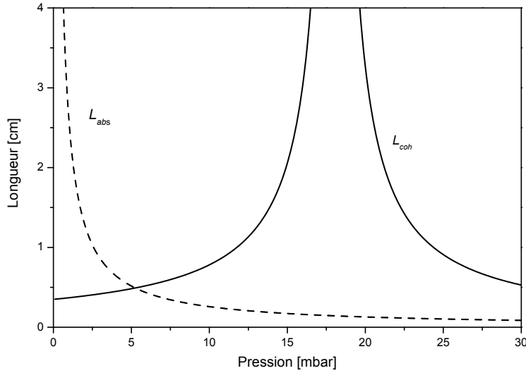
Fig. I.13 : Évolution des longueurs de cohérence (trait plein) et d'absorption (trait pointillé) en présence d'ionisation pour l'harmonique 23 dans l'argon dans le cas ①
