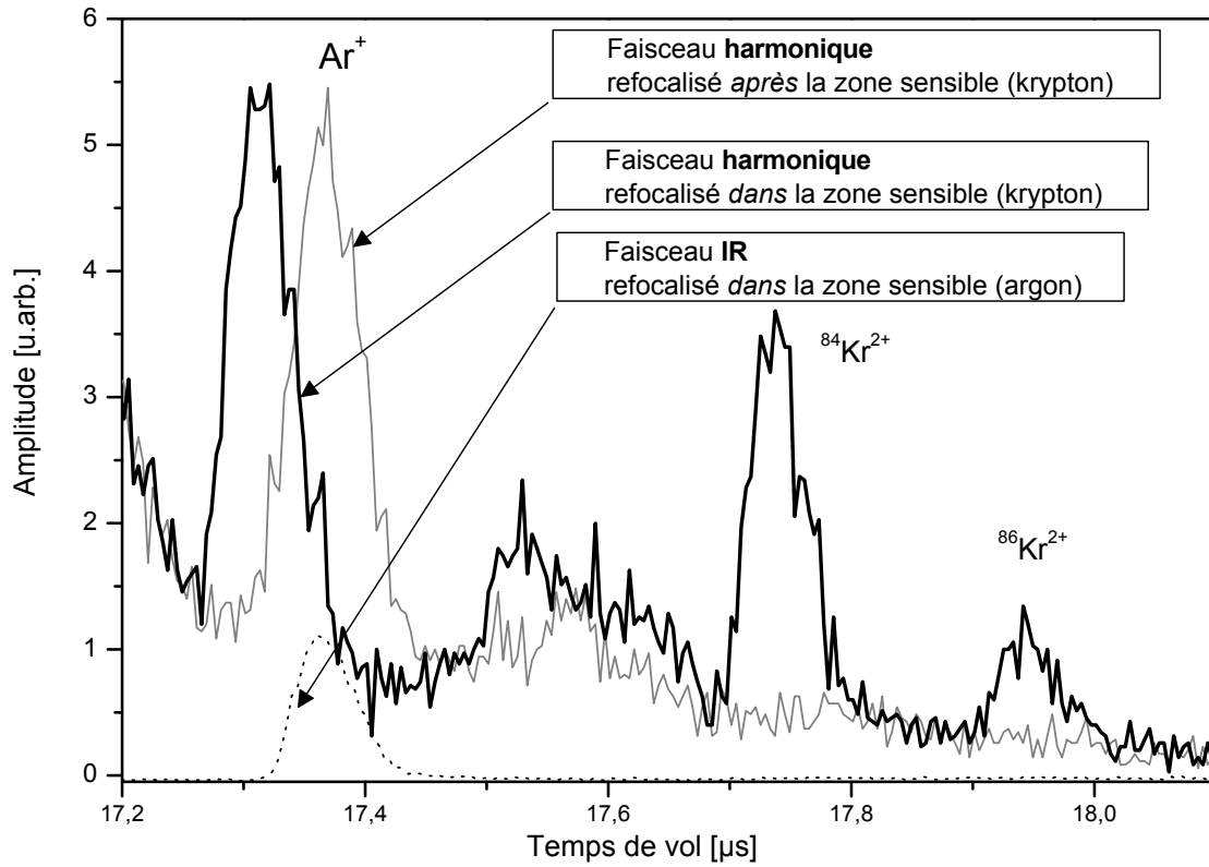
Fig. III.26 : Temps de vol des ions \text{Kr}^{2+} et \text{Ar}^+ . Signal d'ions (trait plein) dû au faisceau harmonique refocalisé dans la zone sensible ( z=0 mm). Signal d'ions (trait gris) dû au faisceau harmonique refocalisé hors la zone sensible ( z=6 mm). La pression dans la zone sensible est de P(\text{Kr})=2.10^{-4} mbar. La pression dans la cellule de génération d'harmoniques remplie de xénon est P(\text{Xe})=14 mbar. Énergie incidente sur la cellule E=2.5 mJ. Le signal d'ions dû au faisceau IR refocalisé dans la zone de détection ( z=0 mm) avec de l'argon comme gaz de détection P(\text{Ar})=3.10^{-7} mbar.
