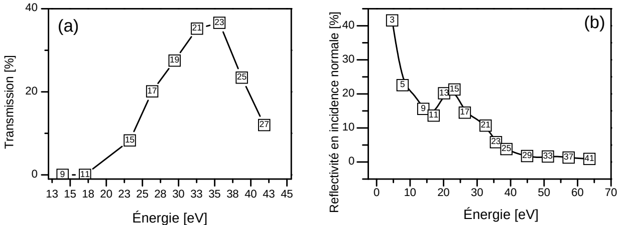
Fig. III.18 : (a) Transmission expérimentale d'un filtre en aluminium d'épaisseur 1500 Å en fonction de l'énergie des photons incidents. (b) Réflectivité théorique du miroir en platine pour une incidence normale en fonction de l'énergie des photons incidents d'après [Palik 85]. Les ordres des harmoniques sont indiqués sur la courbe.
