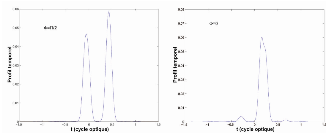
Fig. II.3 : Profils temporels des harmoniques de la coupure sélectionnées par un filtre Gaussien de largeur 9\omega_0 pour \Phi = \pi/2 (à gauche) et \Phi = 0 (à droite) [de Bohan et al. 98].
