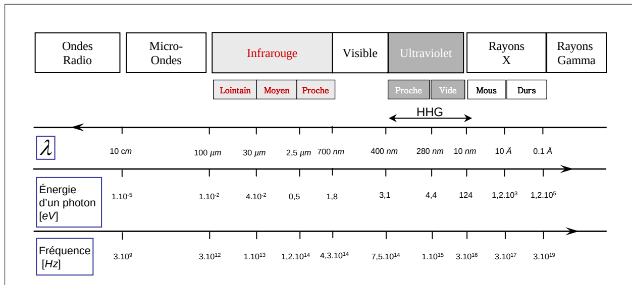
Fig. 2 : Spectre électromagnétique.
