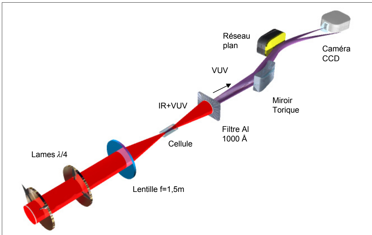
Fig. II.19 : Dispositif expérimental.
