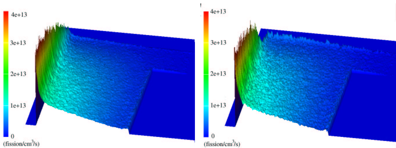
FIG. 5.3 – Répartitions des fissions dans le quart de coeur supérieur droit pour deux configurations : réflecteur axial mince en graphite (à gauche) et réflecteur axial en ZrO_2 (à droite).
