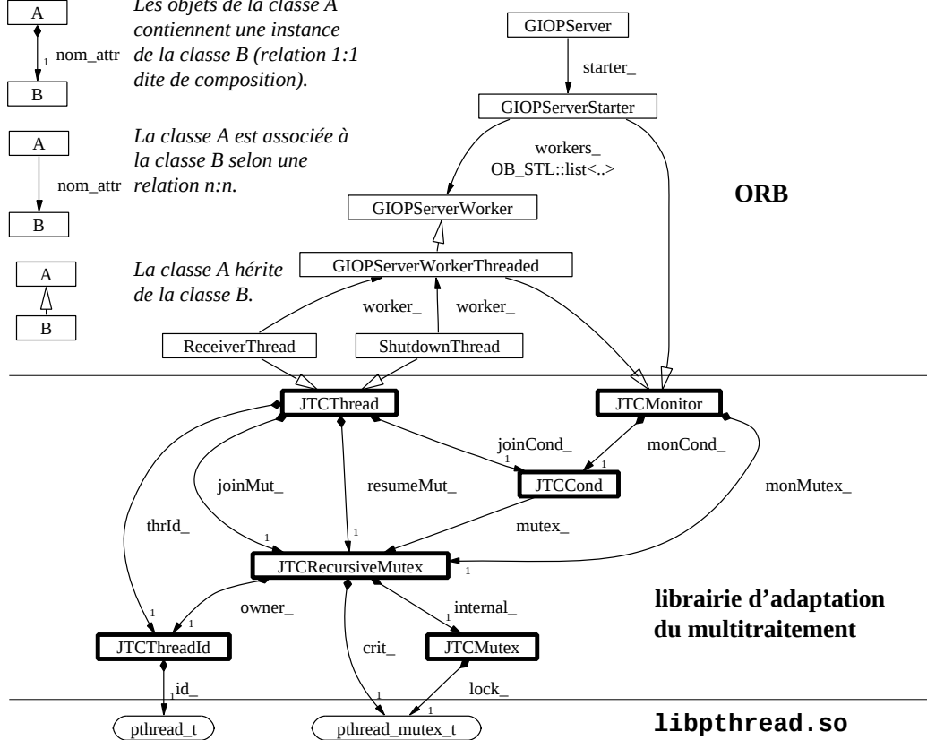
FIG. 5.18 : Ramifications structurelles de la bibliothèque libpthread.so dans ORBACUS
