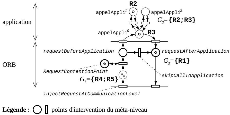
FIG. 5.10 : L'état à restaurer
