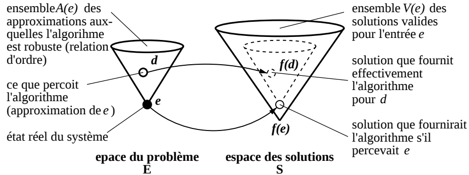
FIG. 4.7 : « Robustesse » d'un algorithme à l'approximation
