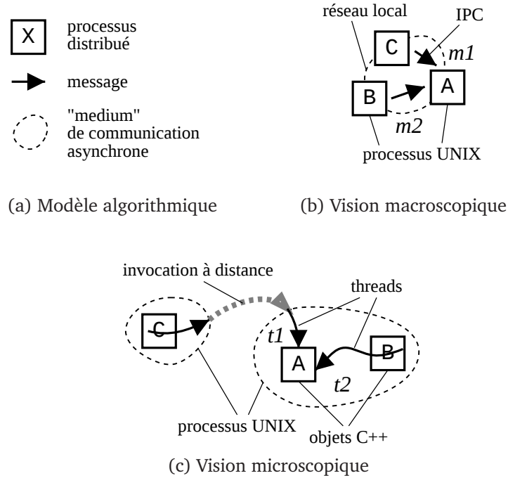
FIG. 4.6 : Diversité des correspondances entre algorithme et implémentation
