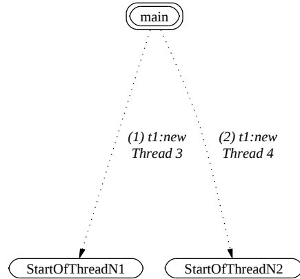
FIG. B.8 : Après abstraction des méthodes POSIX pthread_... du graphe B.7
