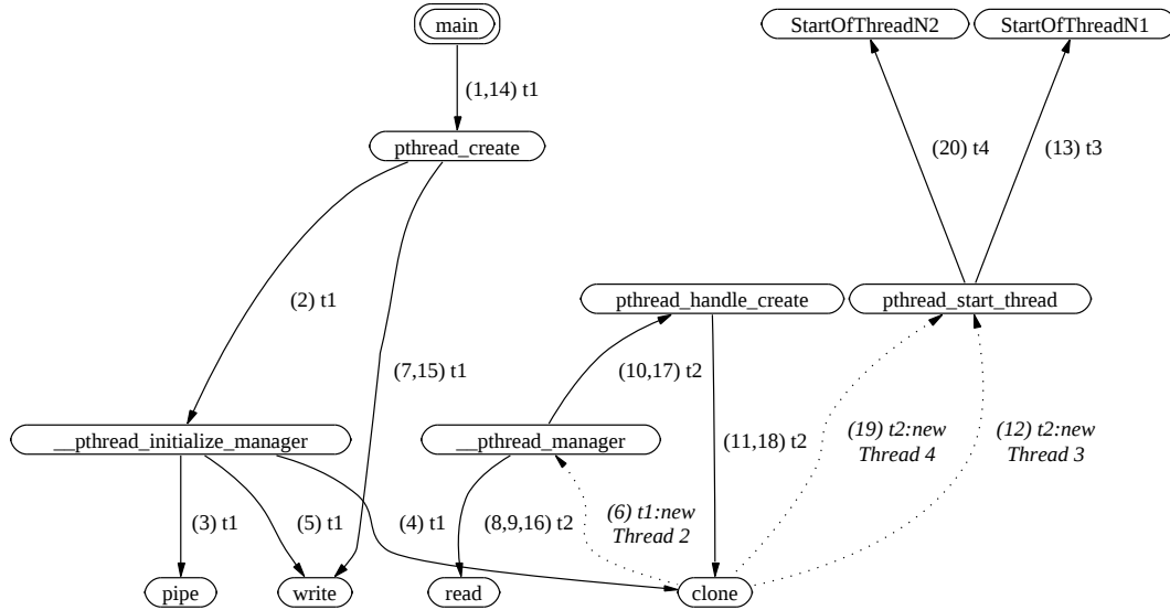
FIG. B.4 : Création de deux brins par la bibliothèque de multitraitement de LINUX 2.4
