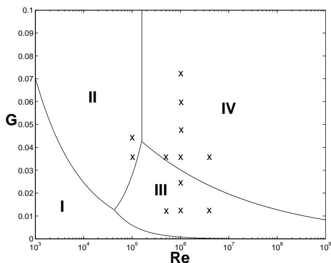
FIG. B.1 – Les 4 régimes d'écoulement rencontrés dans une cavité de type rotor-stator fermée, selon Owen et Rogers [170], avec (x) les cas traités. Le régime I correspond à un écoulement laminaire à couches limites jointes, le régime III à un écoulement turbulent à couches limites jointes. Dans les régimes II et IV , les couches limites sont séparées, et l'écoulement est respectivement laminaire et turbulent
