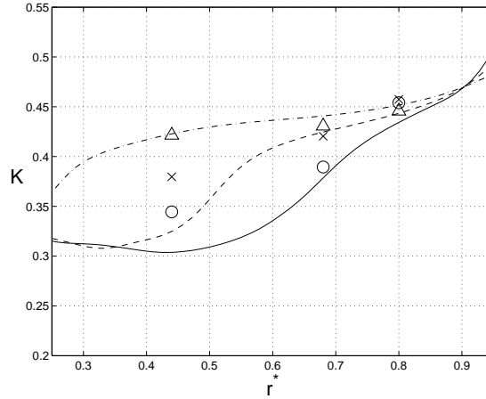
FIG. 4.6 – Évolutions radiales du coefficient d'entraînement K pour G = 0.036 et trois nombres de Reynolds : (-, o) Re = 5.19 \times 10^5 , (-., \times) Re = 1.04 \times 10^6 , (-, \triangle) Re = 4.15 \times 10^6 ; (lignes) modèle RSM, (symboles) mesures par LDA.
