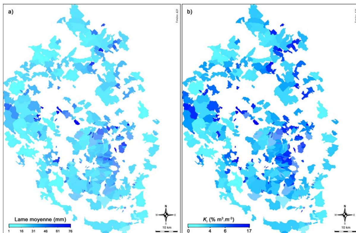
Fig.IV-19 : représentation par bassin des sorties du modèle Zarbhy pour les 377 bassins élémentaires sur la période 1992-2003; a) moyennes des lames annuelles; b) coefficients d'écoulement interannuels.
