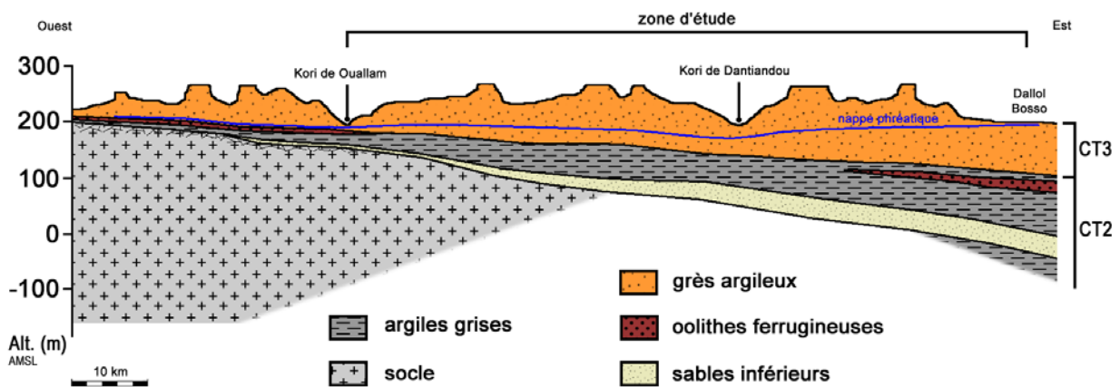
Fig.II-18 : coupe géologique schématisée à 13°40'N à travers le degré carré de Niamey (d'après Monfort, inédit, modifié).
