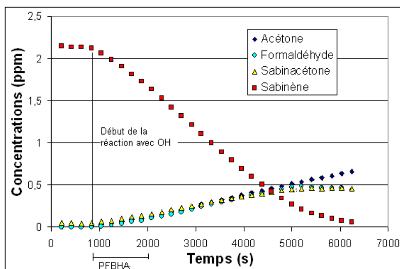
Figure 81 : Courbe cinétique de la réaction entre le sabinène et OH du 19/11/03 (CRAC, absence de NO_x ).
