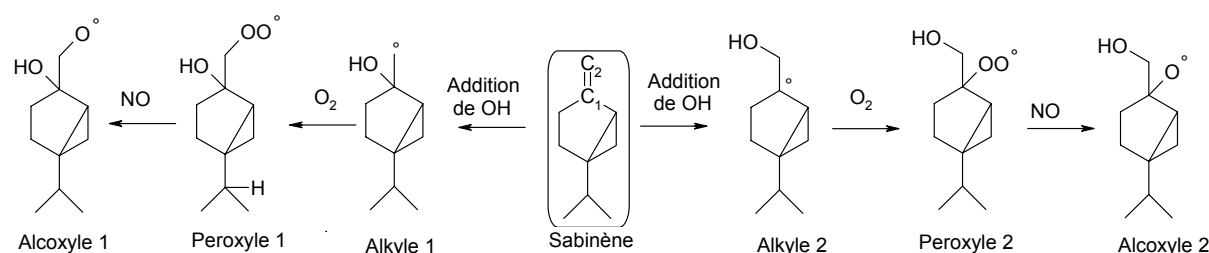
Figure 84 : Première étape de la réaction entre le sabinène et OH : production des radicaux alcoxy 1 et 2.
