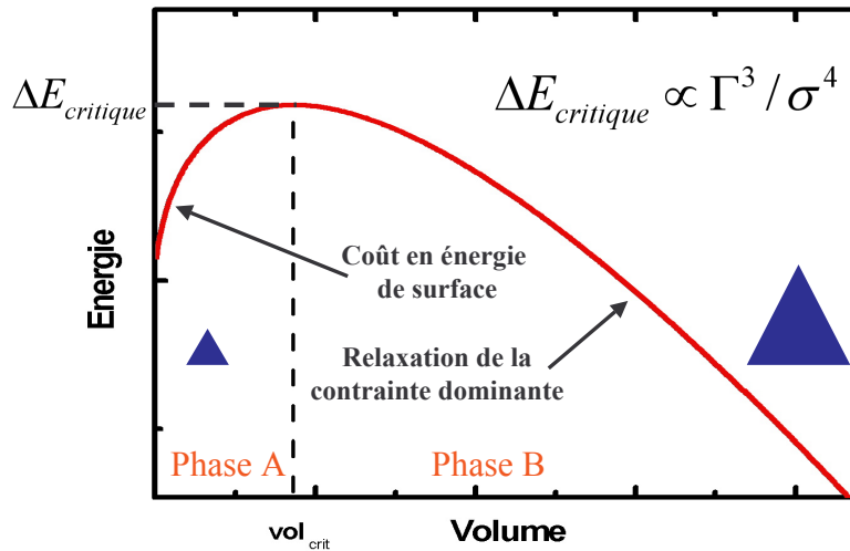
FIG. 1.10 – Variation d'énergie d'une BQ isolée en fonction de son volume. La barrière énergétique de nucléation est proportionnelle à \Gamma^3/\Phi^4 , \Gamma l'excès d'énergie de surface et \Phi la contrainte, d'après [107].
