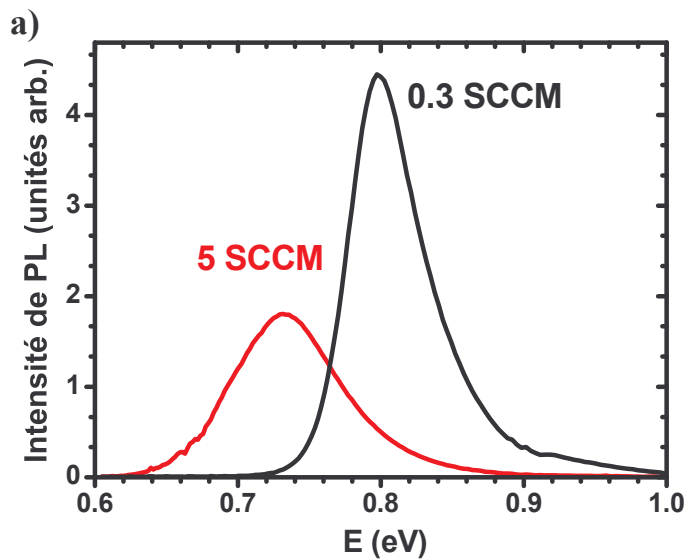
FIG. 3.13 – Spectres de PL à température ambiante d'échantillons InAs/Q1,18 encapsulés par du Q1,18, pour deux débits d'AsH 3 : 0,3 SCCM et 5 SCCM (a).
