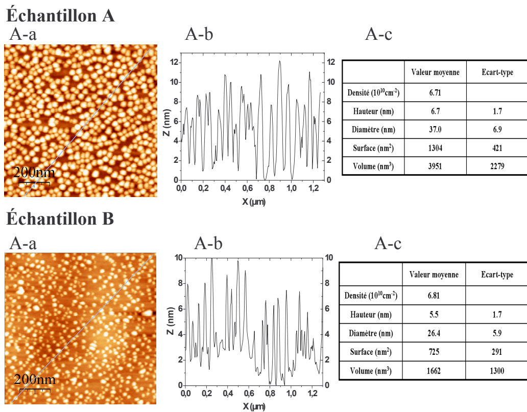
FIG. 4.7 – Images AFM (a), profils de la surface (b) et données statistiques (c) pour l'échantillon de référence sans premier cap de Q1,18 (A) et pour l'échantillon avec premier cap Q1,18.
