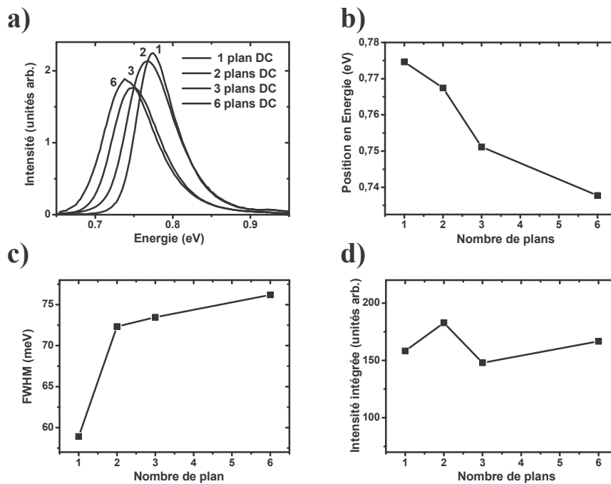
FIG. 5.8 – Spectres de PL à température ambiante pour des empilements de BQs d'InAs DC Q1,18/Q1,18 avec un espaceur de 20 nm et un premier cap de 2,2 nm (a). Evolution de l'énergie d'émission en fonction du nombre de plans (b). Evolution de la largeur totale à mi-hauteur (FWHM) en fonction du nombre de plans (c). Evolution de l'intensité intégrée en fonction du nombre de plans (d).
