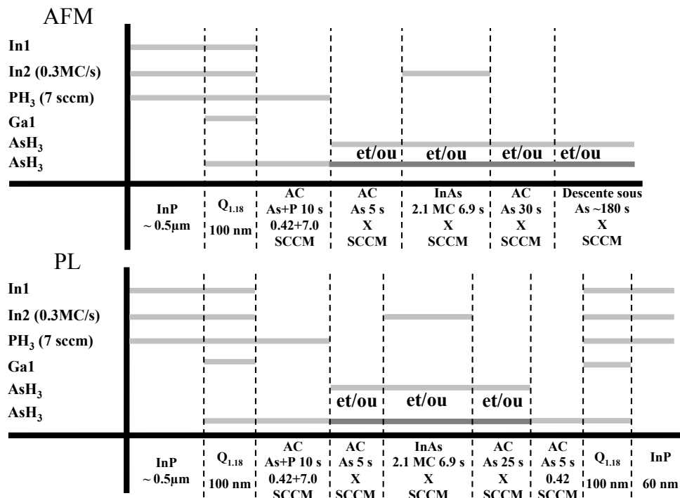
FIG. 3.6 – Séquences de croissance des échantillons de l'étude du flux d'As 2 pour l'AFM et la PL. Les teintes pour la voie d'arsine correspondent à des débits différents
