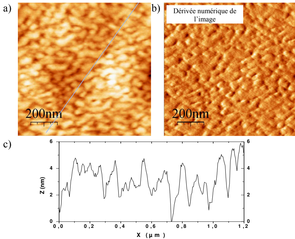
FIG. 4.13 – Images AFM (a), vue en coupe (b) et profil de l'image AFM (c) pour un échantillon de BQs partiellement recouvertes par un premier cap de Q1,18 de 3 nm et un AC sous P_2 de 120 s.
