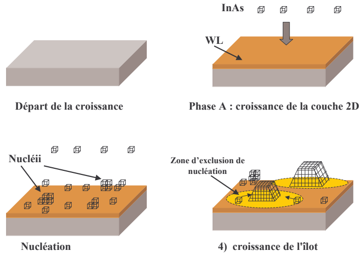
FIG. 1.14 – Départ de la croissance, puis croissance de la WL jusqu'à son épaisseur sur-critique où ont lieu l'étape de nucléation, puis celle de croissance des BQs avec extension de la zone d'exclusion autour des BQs formées.
