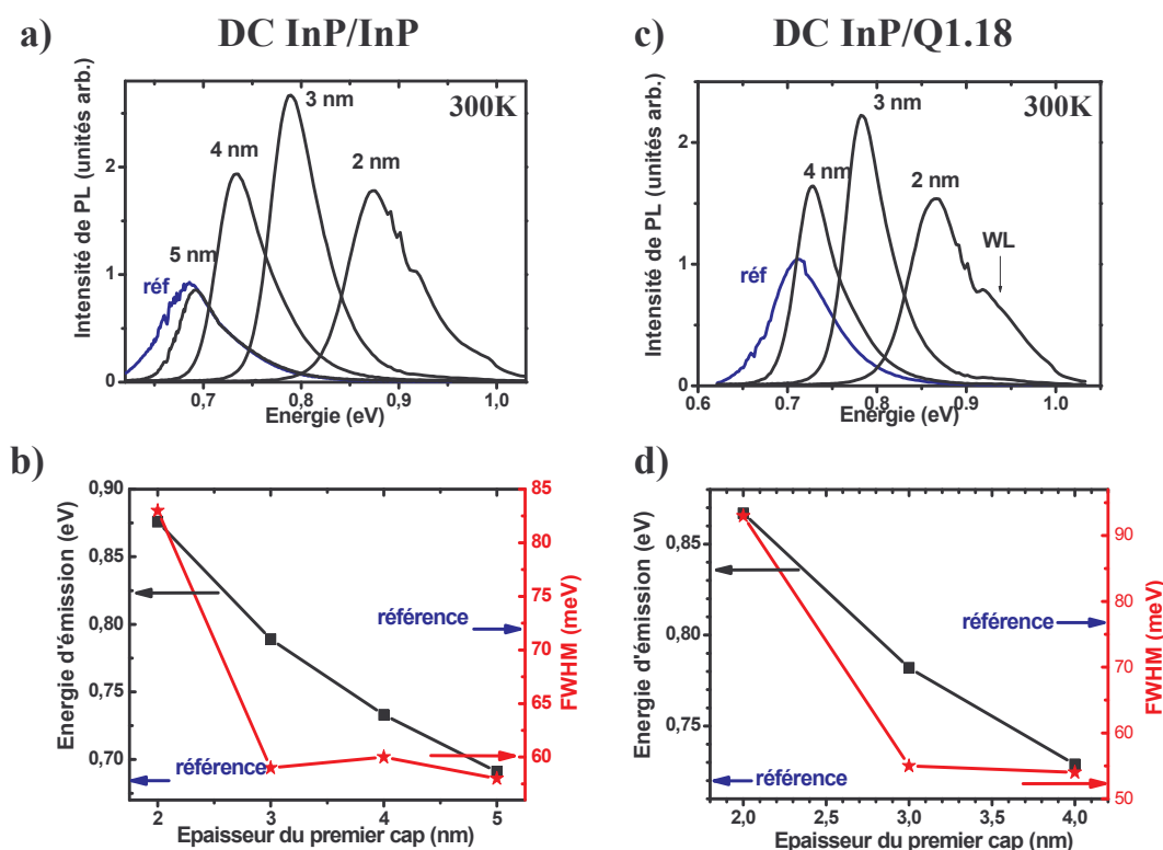
FIG. 4.4 – Spectres de luminescence à température ambiante de BQs DC InP/InP (a) et DC InP/Q1,18 (c) en fonction de l'épaisseur du premier cap d'InP et variation de l'énergie de luminescence et de la largeur totale à mi-hauteur en fonction de l'épaisseur du premier cap pour le DC InP/InP (b) et In/Q1,18 (d).
