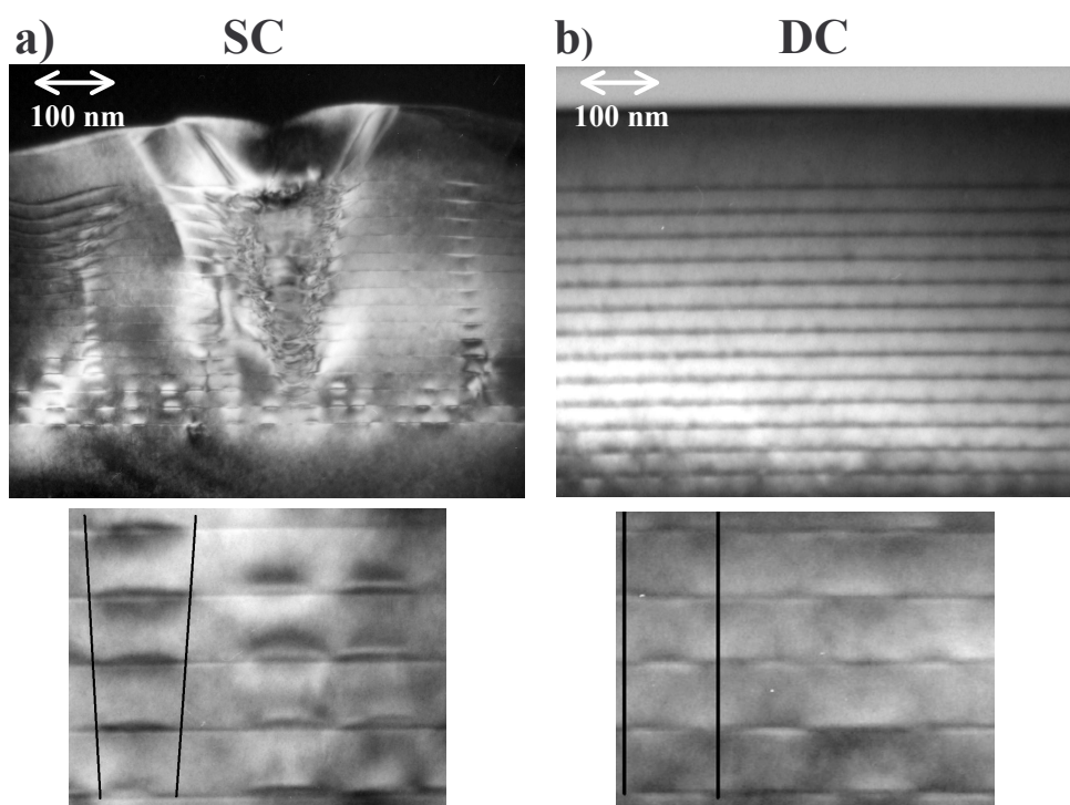
FIG. 5.3 – Clichés MET en coupe selon [33-2] à 200 kV sur Philips CM20 en champ sombre (113). Vue d'ensemble (images du haut) et des premiers plans (images du bas) d'un empilement de quinze plans de BQs réalisés en utilisant une procédure d'encapsulation SC (a) et DC InP (b). Les traits sur les images du bas permettent de suivre l'évolution de la taille latérale. Clichés réalisés par A. Ponchet.
