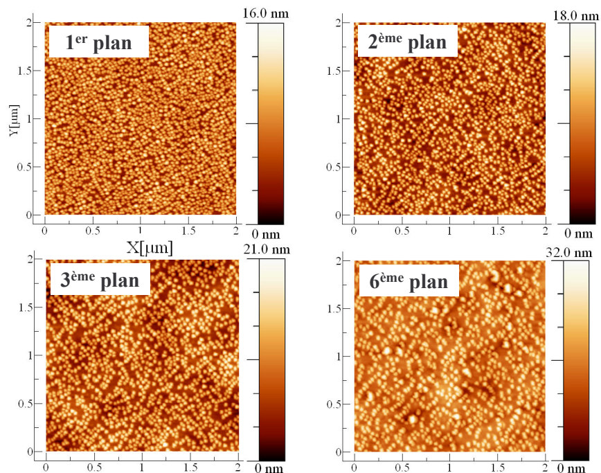
FIG. 5.10 – Images AFM de 2 \times 2 \mu\text{m}^2 pour le premier plan (a), le second (b), le troisième (c) et le sixième plan non recouvert (d).
