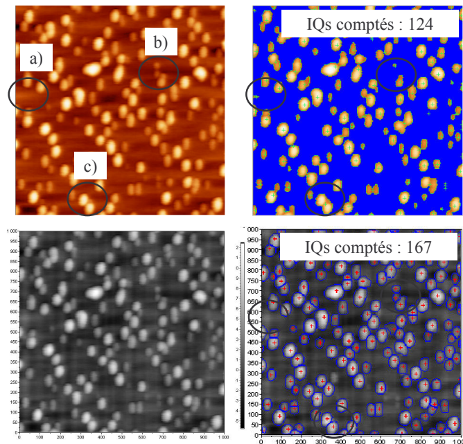
FIG. 2.11 – Comparatif de l’analyse d’une image AFM par une méthode classique (haut) et par le logiciel spécialement dédié (bas)
