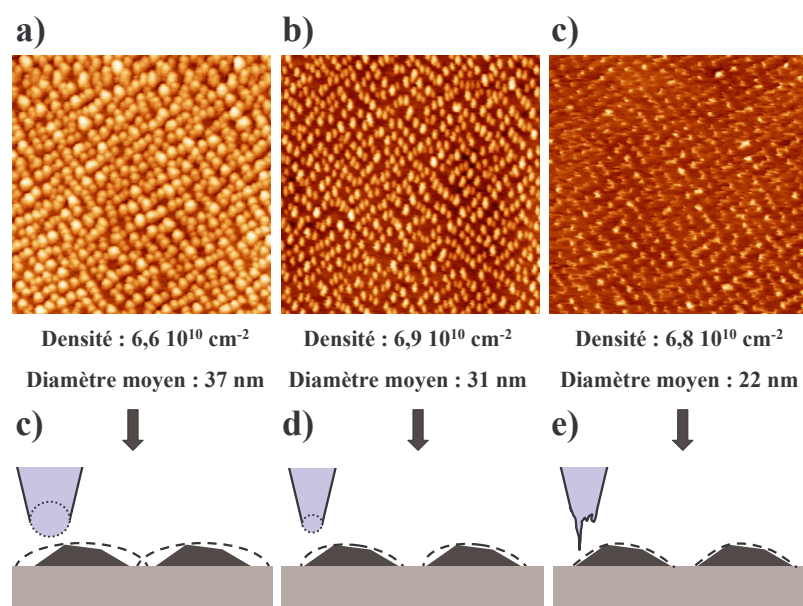
FIG. 2.9 – Trois images AFM d'un même plan de BQs en utilisant par trois pointes UL06A par ordre décroissant de rayon de courbure (a, b, c) et schéma de la convolution avec la pointe dans chaque cas (d, e, f). Les traits en pointillés représentent l'image obtenue après passage de la pointe sur l'échantillon.
