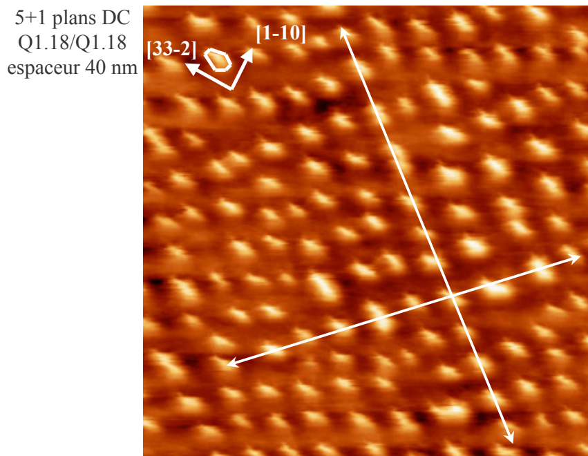
FIG. 5.25 – Image AFM de 0,5 \times 0,5 \mu\text{m}^2 d'un empilement de 5+1 plans de BQs DC Q1,18/Q1,18 avec un espaceur de 40 nm et un faible flux d'As 2 .
