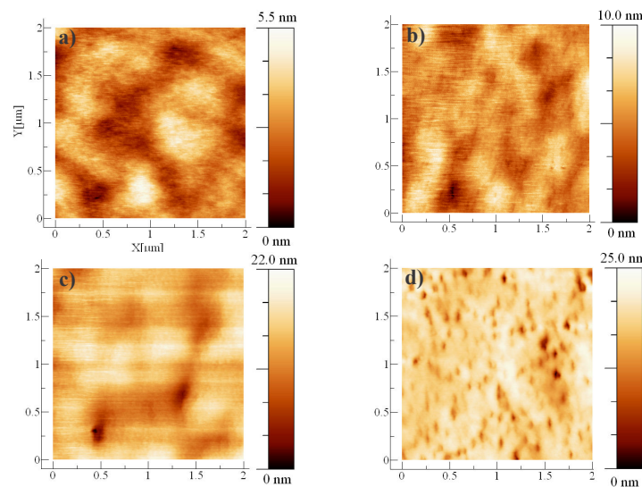
FIG. 5.12 – Vue en coupe des surfaces à partir des images AFM de la surface de Q1,18 avant épitaxie du second plan (a), troisième plan (b), sixième plan (d) de BQs.
