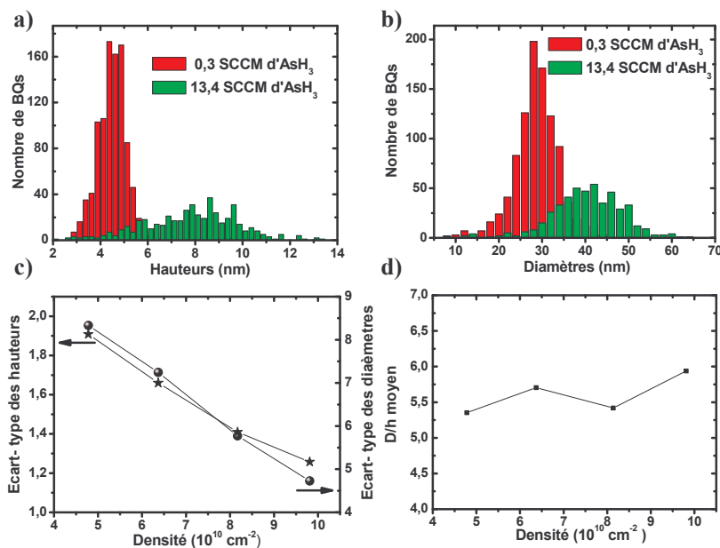
FIG. 3.9 – Distribution des hauteurs (a) et des diamètres (b) pour deux débits d'AsH 3 , 13,4 SCCM et 0,3 SCCM. Ecart-type de la distribution de hauteurs et de diamètres en fonction de la densité (c). Rapport d'aspect Diamètre sur hauteur ( D/h ) en fonction de la densité surfacique d'BQs. (d)
