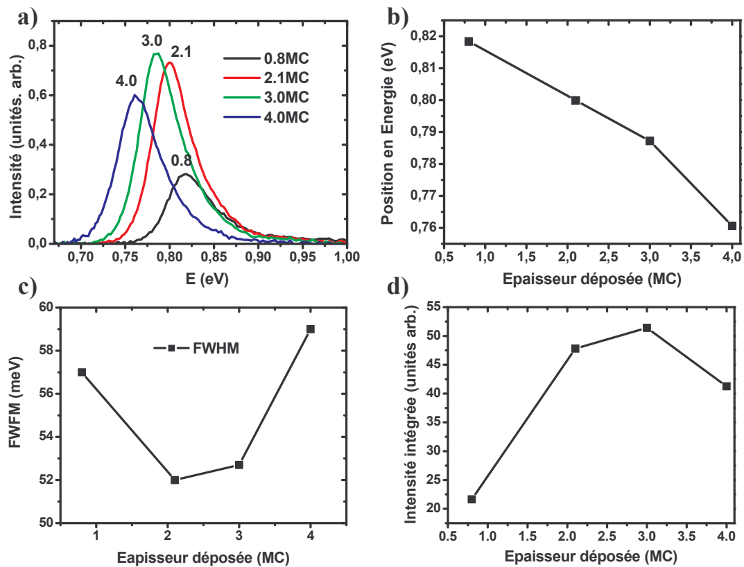
FIG. 3.21 – Spectres de PL à température ambiante pour des épaisseurs déposées de 0,5 MC à 4 MC (a). Evolution de la position en énergie du maximum des spectres de PL pour ces échantillons (b). Evolution de la largeur totale à mi-hauteur (FWHM) des spectres de PL (c) et de leurs intensités intégrées (d) en fonction de l'épaisseur d'InAs déposée.
