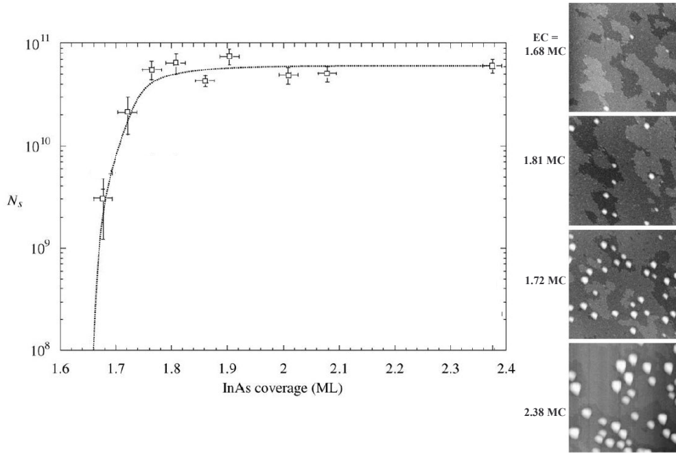
FIG. 1.6 – Evolution de la densité de BQs en fonction de l'épaisseur déposée (à gauche). Images STM (états pleins) de BQs d'InAs/GaAs en fonction de l'épaisseur déposée (à droite). D'après [23].
