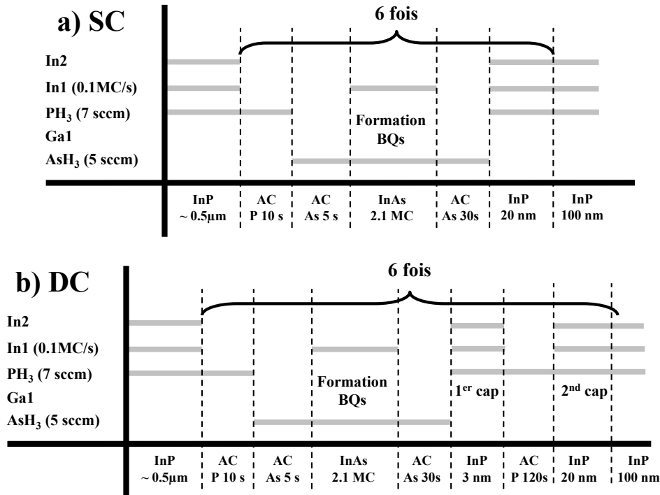
FIG. 5.1 – Séquences de caches pour les échantillons des séries d'empilements SC (a) et DC (b).
