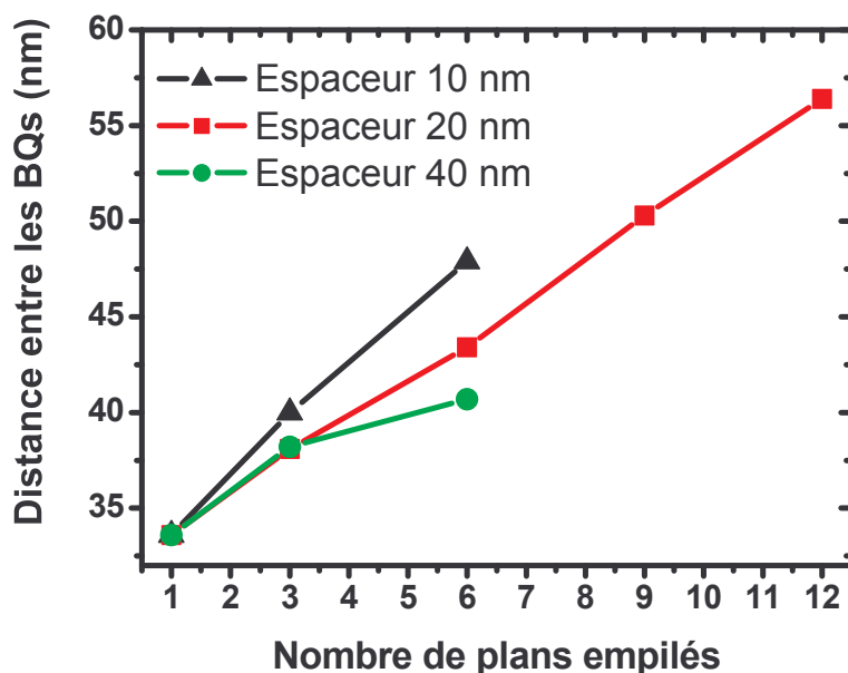
FIG. 5.24 – Distance moyenne entre les BQs en fonction du nombre de plans de BQs DC Q1,18/Q1,18 avec un espaceur de 10, 20 et 40 nm et un faible flux d'As 2 .
