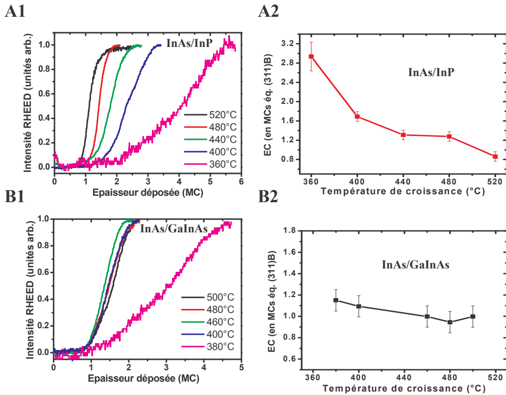
FIG. 3.4 – Evolution de l'intensité RHEED d'une tache de diffraction 3D en fonction de l'épaisseur déposée sur InP et GaInAs (A1 et B1) et évolution de l'EC en fonction de la température de croissance pour ces deux couches tampon (A2 et B2). L'incertitude sur la détermination de l'EC est indiquée par des segments.
