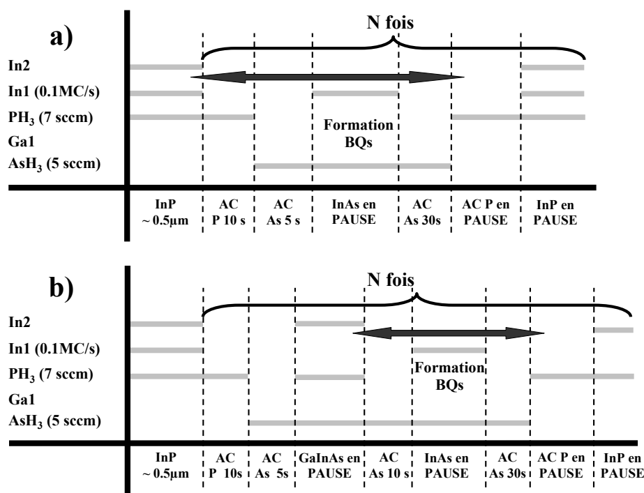
FIG. 3.1 – Séquences de caches pour les échantillons des séries EC en fonction de la température pour la croissance sur couche tampon InP (a) et GaInAs (b).
