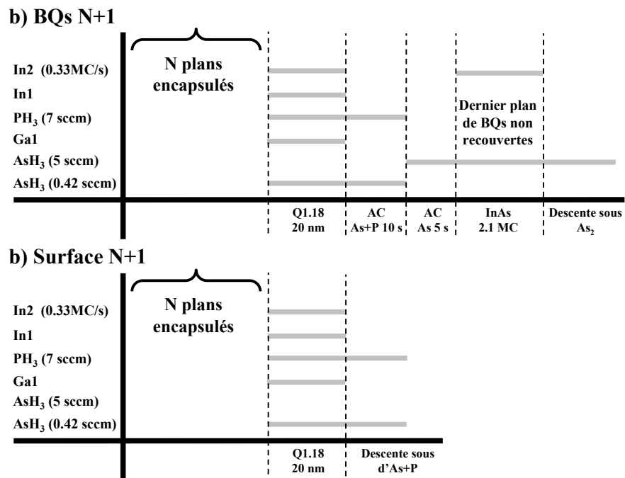
FIG. 5.9 – Séquences de croissance d'empilements de BQs DC Q1,18/Q1,18 avec un espaceur de 20 nm et un flux d'As 2 de 5 SCCM, pour des échantillons dont le dernier plan est non recouvert (a) ou le dernier espaceur est non recouvert (b).
