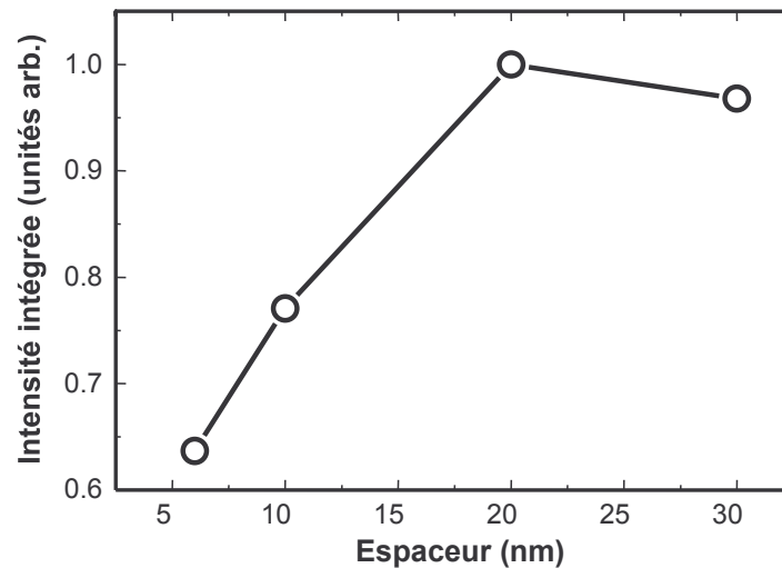
FIG. 5.6 – Evolution de l'intensité intégrée à température ambiante d'une structure à 3 plans de BQs DC InP/InP en fonction de l'épaisseur de l'espaceur entre les plans.
