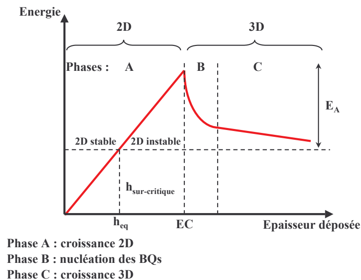
FIG. 1.13 – Evolution de l'énergie totale du système lors des 3 phases (A,B,C) de la croissance des BQs). h_{eq} est l'épaisseur de la WL d'équilibre, et h_{sur-crit} l'épaisseur de la couche 2D métastable.
