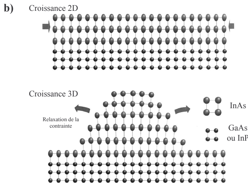
FIG. 1.5 – Transformation 2D/3D de la croissance : mode SK.
