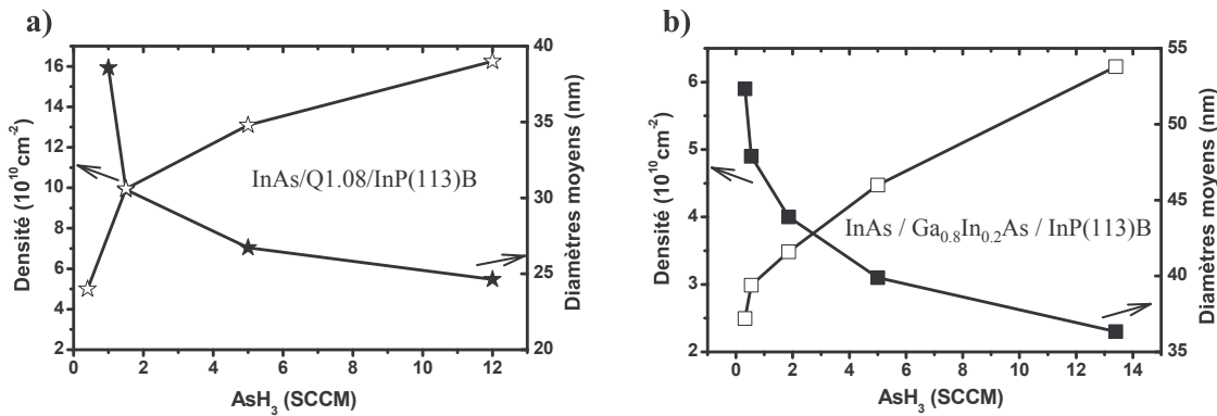
FIG. 3.11 – Evolution de la densité (symboles pleins) et du diamètre moyen (symboles vides) en fonction du débit d' \text{AsH}_3 , pour la croissance de BQs sur une couche tampon de Q1,08 (a) et GaInAs (b). Les échelles en Y sont adaptées aux valeurs différentes pour les graphes (a) et (b).
