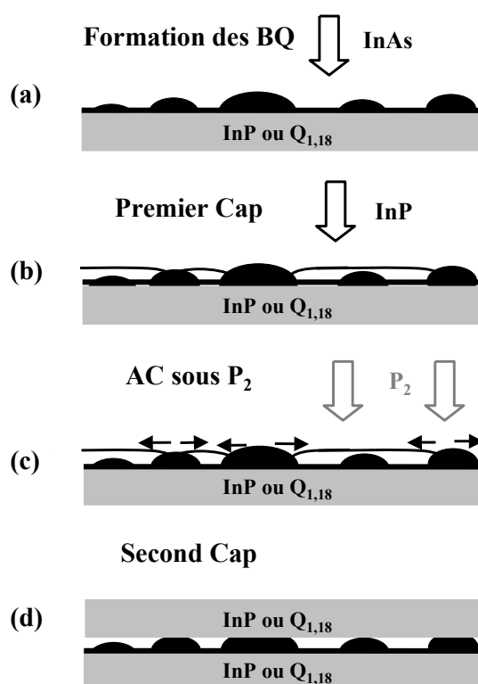
FIG. 4.2 – Schéma de principe du DC InP/InP et InP/Q1,18. Les 4 étapes sont : la formation de BQs d'InAs (a), le premier cap d'InP (b), l'AC sous P_2 (c) et le second cap d'InP ou Q1,18 (d).
