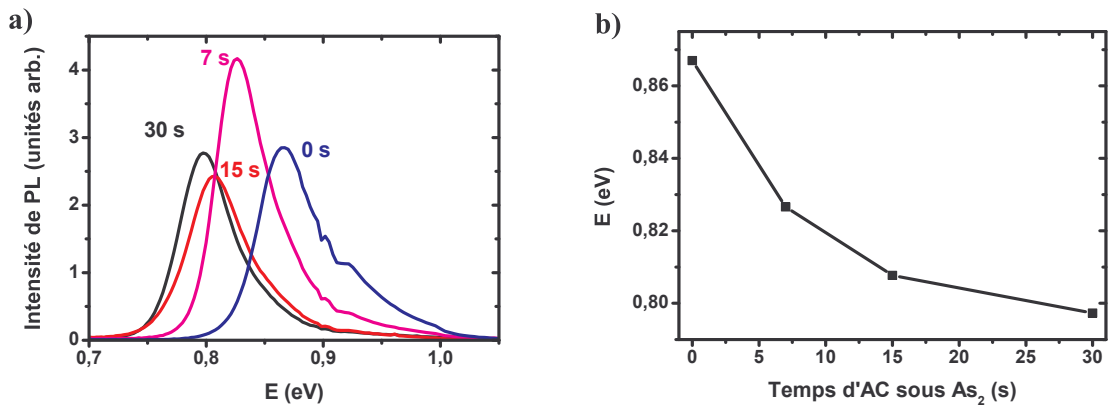
FIG. 3.14 – Spectres de PL à température ambiante pour des BQs d'InAs/Q1,08 en fonction de la durée de l'AC sous As 2 avant encapsulation (a) et évolution de la position en énergie des pics de PL en fonction de la durée de l'AC (b).
