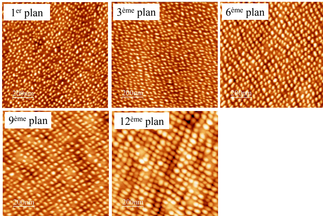
FIG. 5.18 – Images AFM des derniers plans d'un empilement de 0+1 , 2+1 , 5+1 , 8+1 et 11+1 plans de BQs d'InAs DC Q1,18/Q1,18 avec un espaceur de 20 nm à faible flux d'arsenic.
