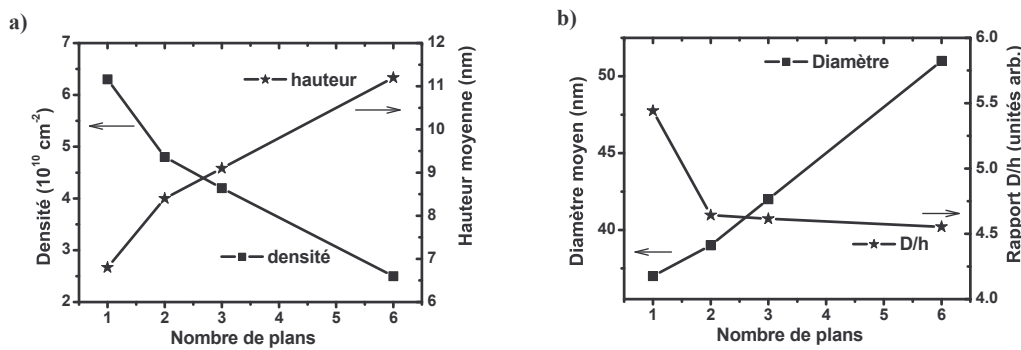
FIG. 5.11 – Evolution de la densité et de la hauteur moyenne en fonction du nombre de plans (a). Evolution du diamètre moyen et du rapport de forme moyen en fonction du nombre de plans.
