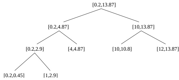
FIG. V.4 – Approche descendante.
