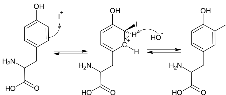
Figure 24 : Mécanisme réactionnel de l'iodation de la tyrosine
