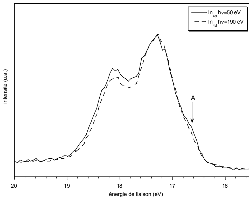
Fig. 9 : niveau de cœur \text{In}_{4d} d'un substrat d' \text{InP}(100) nettoyé ioniquement à deux énergies de faisceaux primaires différentes
