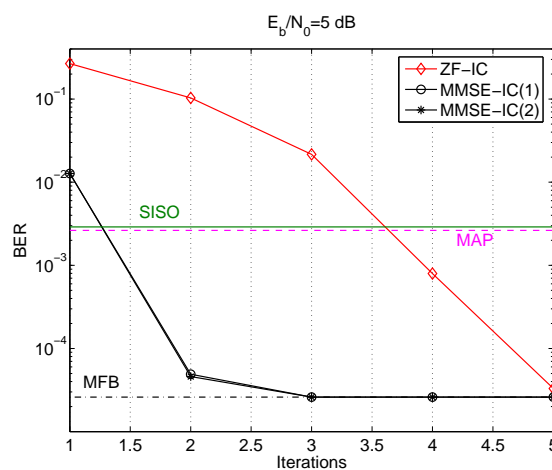
(c) QPSK, \eta = 4 bps/Hz, performances suivant les itérations
