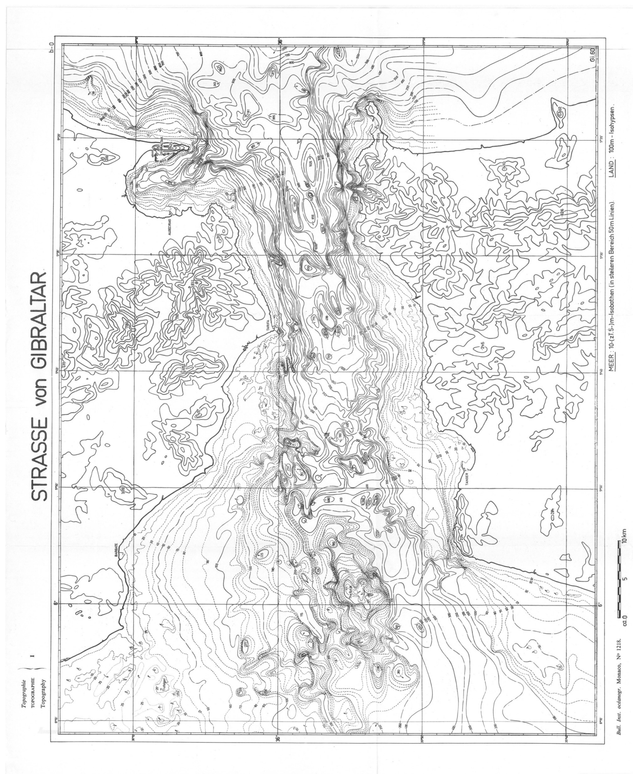
Figure a1 : Carte bathymétrique du détroit de Gibraltar (d'après Giemann, 1961).
