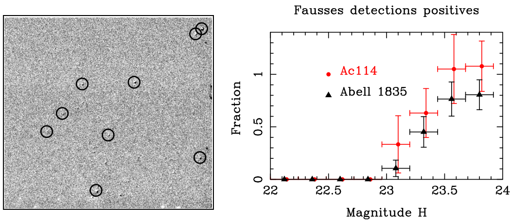
Fig. 4.16: A gauche : image artificielle en bande H utilisée pour mesurer le taux de fausses détections positives. Des résidus sont encadrés à la position des objets brillants. A droite : résultats obtenus pour chaque amas, en terme de fraction d'objets faussement détectés dans l'image de bruit avec les mêmes critères de détection que pour les données de science.
