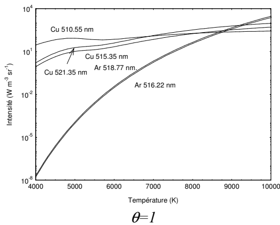
Fig. 3. : Intensités des raies spectrales de cuivre et d'argon en fonction de la température des espèces lourdes à l'équilibre thermique et hors d'équilibre thermique.
