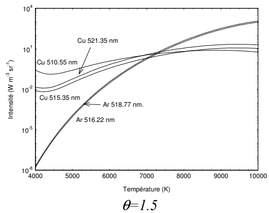
Fig. 3. : Intensités des raies spectrales de cuivre et d'argon en fonction de la température des espèces lourdes à l'équilibre thermique et hors d'équilibre thermique.
