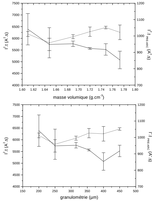
FIGURE 5.38 – Evolution de la contrainte thermique en fonction de la masse volumique du sable compacté et de la granulométrie. — : grandeur exprimée pour le régime de préarc ; — : grandeur exprimée pour le phénomène total. Tension de charge : 460 V ; courant présumé : 3,2 kA.
