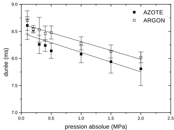
FIGURE 4.17 – Durée du phénomène dans le cas des décharges entre les contacts \text{AgSiO}_2 pour les deux natures de gaz. Tension de charge : U_{CH} = 300 \text{ V} .
