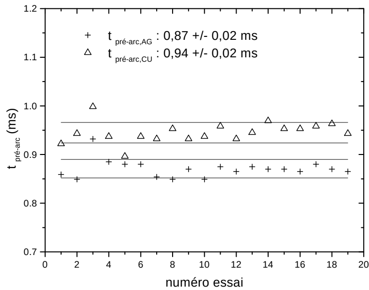
FIGURE 5.23 – Valeurs des temps de préarc pour des éléments fusibles en argent et en cuivre, de dimensions : 70 \text{ mm} \times 5 \text{ mm} \times 0,105 \text{ mm} . Tension de charge : 460 \text{ V} ; courant présumé : 3,2 \text{ kA} .
