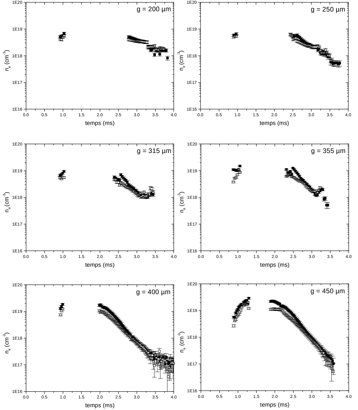
FIGURE 5.44 – Evolution de la densité électronique au cours du phénomène de coupure en fonction de la masse volumique du sable compacté et de la granulométrie. ■ : densité électronique déduite de la transition Si II (2) centrée à 634,71 nm ; □ : densité électronique déduite de la transition Si II (2) centrée à 637,14 nm. Tension de charge : 460 V ; courant présumé : 3,2 kA.
