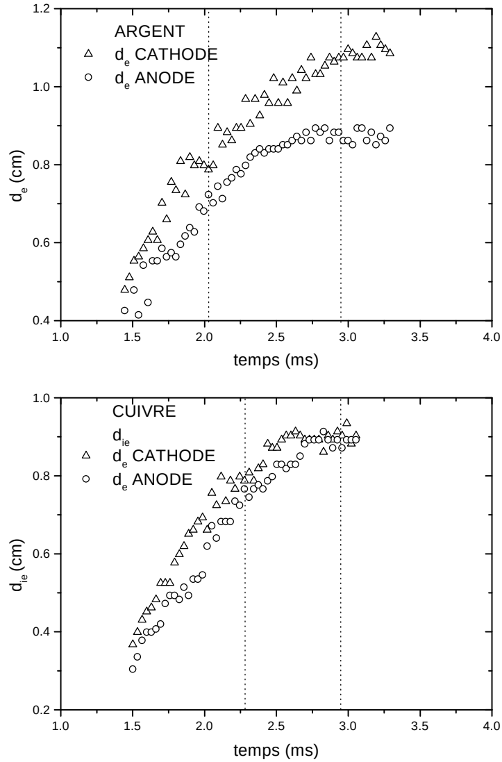
FIGURE 5.8 – Evolution de la dissymétrie de la vitesse de "burn-back" liée à la polarité en fonction du temps ; d_e représente la distance entre la zone centale (sections réduites) et l'électrode.
