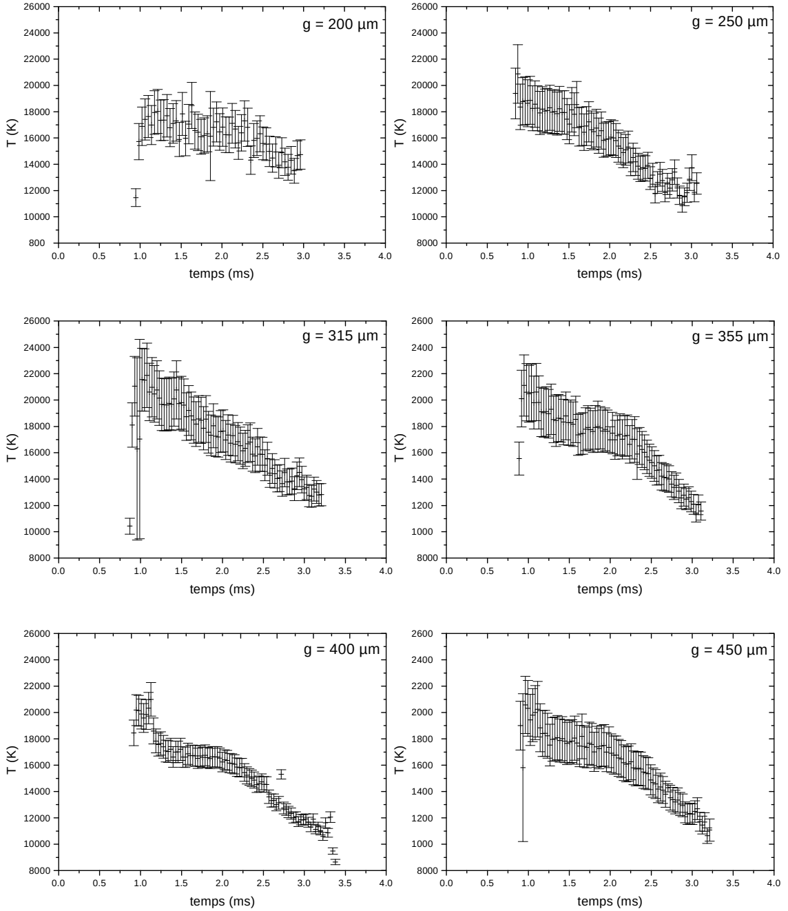
FIGURE 5.42 – Evolution de la température au cours du phénomène de coupure en fonction de la masse volumique du sable compacté et de la granulométrie. Tension de charge : 460 V ; courant présumé : 3,2 kA.
