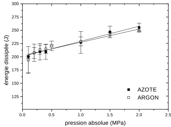
FIGURE 4.18 – Energie dissipée pendant la décharge entre les contacts \text{AgSiO}_2 pour les deux natures de gaz. Tension de charge : U_{CH} = 300\text{ V} .
