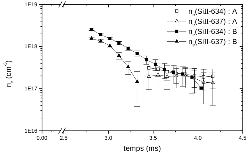
FIGURE 5.29 – Evaluation de la densité électronique à partir des décalages en longueur d'onde du doublet Si II centré à 634,71 nm et 637,14 nm. Etude de l'influence de la position de l'élément fusible par rapport au hublot de visée : configuration A = élément fusible plaqué sur le hublot ; configuration B = élément fusible placé sur le chant. Tension de charge : 460V ; courant présumé : 3,2 kA.
