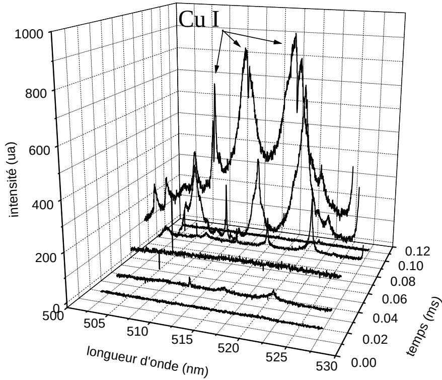
FIGURE 4.12 – Evolution au cours de la décharge du rayonnement issu du capillaire. Tension de charge : U_{CH} = 120\text{ V} . Fil métallique en cuivre.
