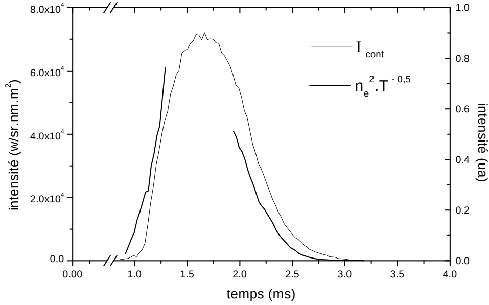
FIGURE 5.21 – Evolution du rayonnement discret et continu pour le domaine centré sur 635 nm. Comparaison entre l'émission continue déduite du spectre expérimental I_{cont} ( W/sr.nm.m^2 ), et la courbe de tendance (chapitre 2) : n_e^2/T^{0,5} (Unité Arbitraire).
