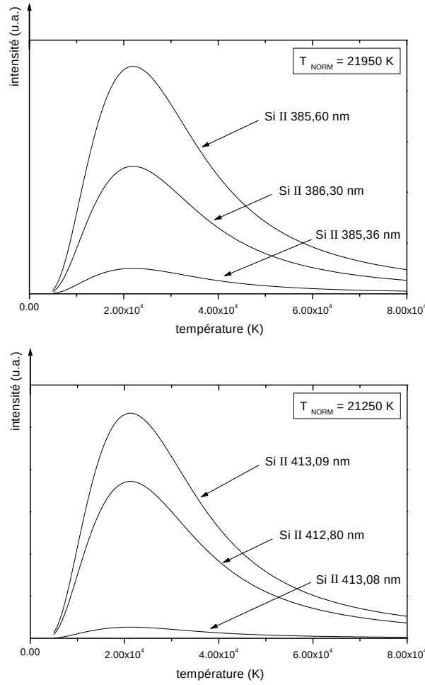
FIGURE 2.2 – Température normale évaluée pour les triplets (1) et (3) du silicium ionisé une fois.
