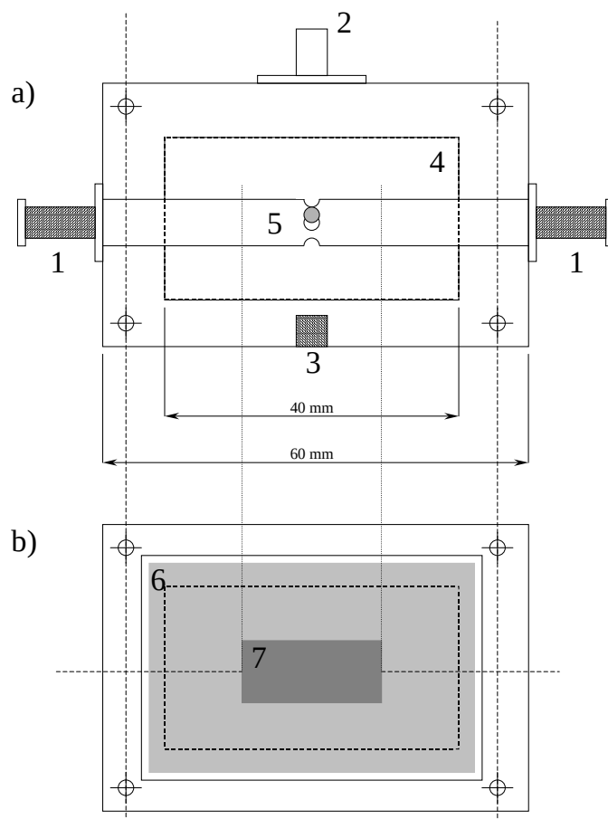
FIGURE 3.3 – Boîtier fusible expérimental de type A : la cavité de remplissage est parallélépipédique, et l'élément fusible est plaqué sur le hublot de visée. L'illustration a) est une vue de dessus du boîtier fusible. L'illustration b) montre la constitution du couvercle et la position des deux hublots de visée. 1 : électrodes ; 2 : obturateur de la cavité de remplissage ; 3 : orifice de fixation du support du boîtier ; 4 : cavité de remplissage ; 5 : élément fusible - le cercle grisé représente la zone à partir de laquelle le rayonnement est intégré ; 6 : hublot principal de visée (verre) ; 7 : hublot supplémentaire (quartz).
