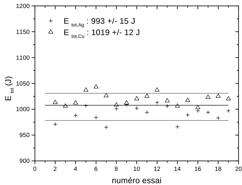
FIGURE 5.25 – Energie totale dissipée pendant la coupure pour des éléments fusibles en argent et en cuivre de dimensions : 70\text{ mm} \times 5\text{ mm} \times 0,105\text{ mm} . Tension de charge : 460\text{ V} ; courant présumé : 3,2\text{ kA} .
