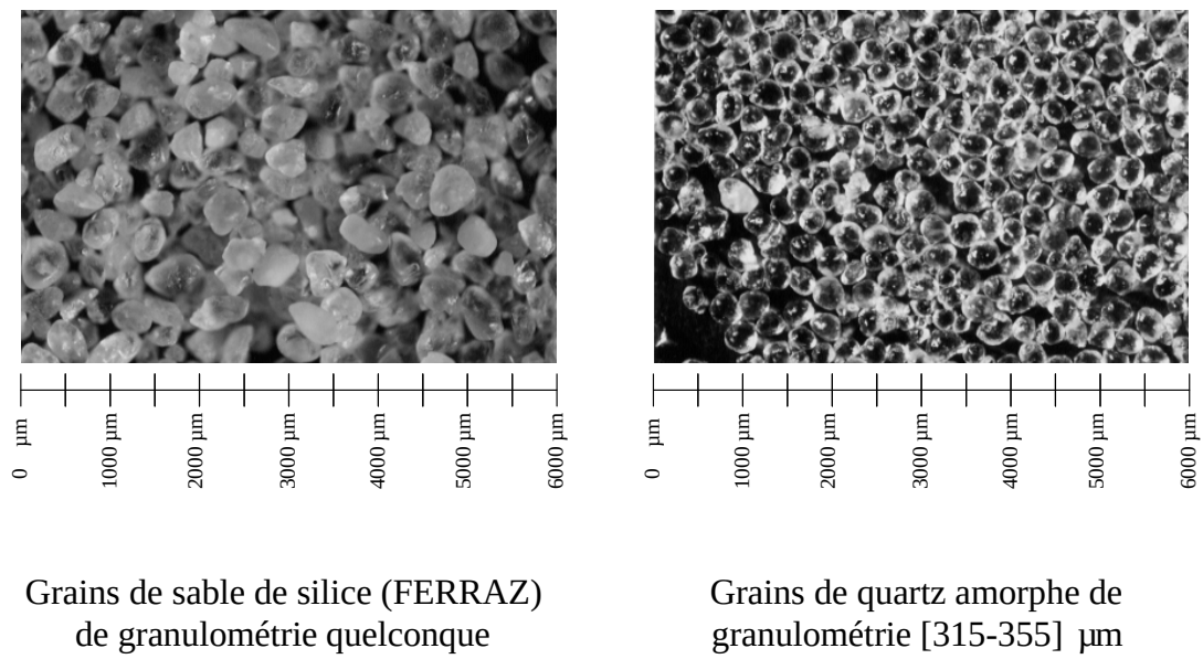
FIGURE 3.7 – Visualisation des grains de sable de silice et des grains de quartz amorphe.
