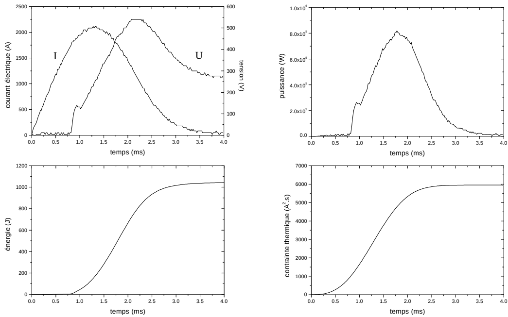
FIGURE 5.24 – Evolution des grandeurs électriques aux bornes du fusible au cours de la coupure. Tension de charge : 460 \text{ V} ; courant présumé : 3,2 \text{ kA} .
