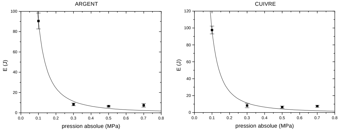
FIGURE 4.9 – Variation de l'énergie dissipée dans le cas des décharges sur les fils métalliques en fonction de la pression au sein du milieu gazeux (air comprimé). Tension de charge : U_{CH} = 120 \text{ V} .
