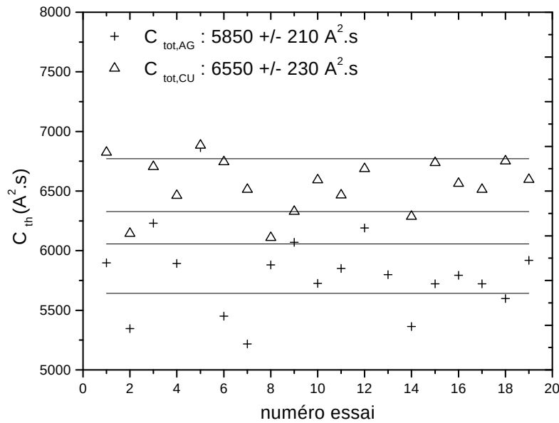
FIGURE 5.26 – Contrainte thermique totale pour des éléments fusibles en argent et en cuivre de dimensions : 70\text{ mm} \times 5\text{ mm} \times 0,105\text{ mm} . Tension de charge : 460\text{ V} ; courant présumé : 3,2\text{ kA} .
