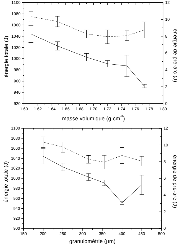
FIGURE 5.39 – Evolution de l'énergie en fonction de la masse volumique du sable compacté et de la granulométrie. — : grandeur exprimée pour le régime de préarc; — : grandeur exprimée pour le phénomène total. Tension de charge : 460 V ; courant présumé : 3,2 kA.
