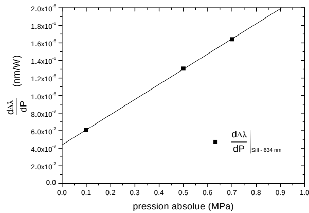
FIGURE 4.7 – Evolution du coefficient d'élargissement par unité de puissance électrique en fonction de la pression dans l'enceinte, pour la transition Si II centrée à 634,71 \text{ nm} .
