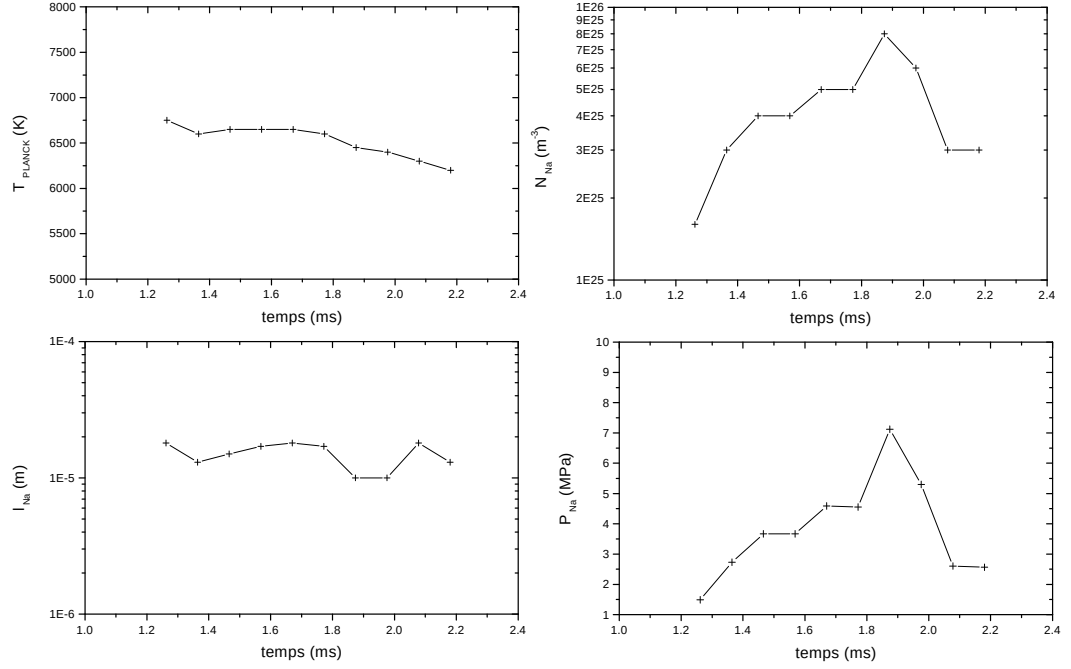
FIGURE 5.33 – Paramètres de caractérisation de la couche limite sodium. T_{\text{PLANK}} : température obtenue par superposition d'un spectre de corps noir ; N_{\text{Na}} : densité en atomes Na I ; l_{\text{Na}} : épaisseur de la couche limite ; P_{\text{Na}} : pression déduite de la densité en atomes Na I. Tension de charge : 460\text{ V} ; courant présumé : 3,2\text{ kA} .
