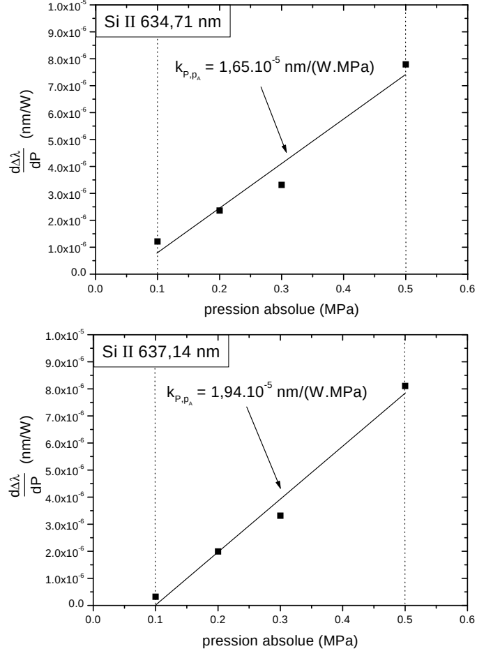
FIGURE 4.25 – Evolution des coefficients d'élargissement par unité de puissance pour les deux composantes du multiplet Si II (2) sur le domaine de pression [0, 1 - 0, 5] \text{ MPa} .
