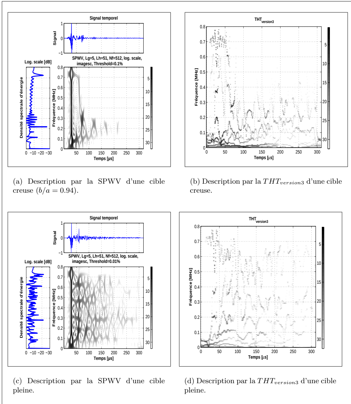
Figure VI.11 — Descriptions temps-fréquence d'une cible cylindrique en Nickel-Molybdène ( a = 15mm , c_l = 5554m/s , c_t = 3021m/s , \rho = 9217kg/m^3 ), l'axe d'observation étant perpendiculaire à la direction principale du cylindre.
