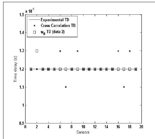
(d) Estimation des retards sur la ligne de capteurs par T_{B_\Psi} et T_{B_{MF}} .
