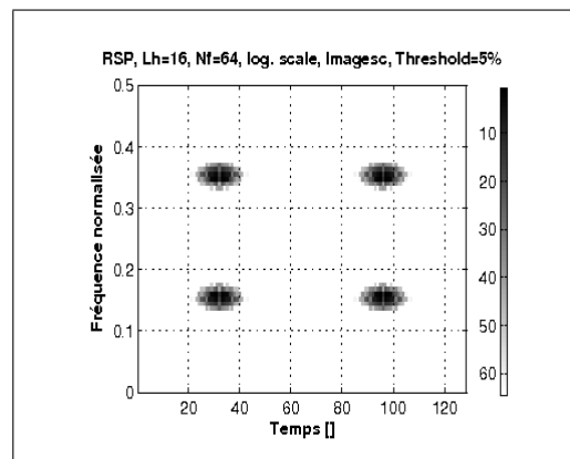
(b) Réallocation du spectrogramme.
