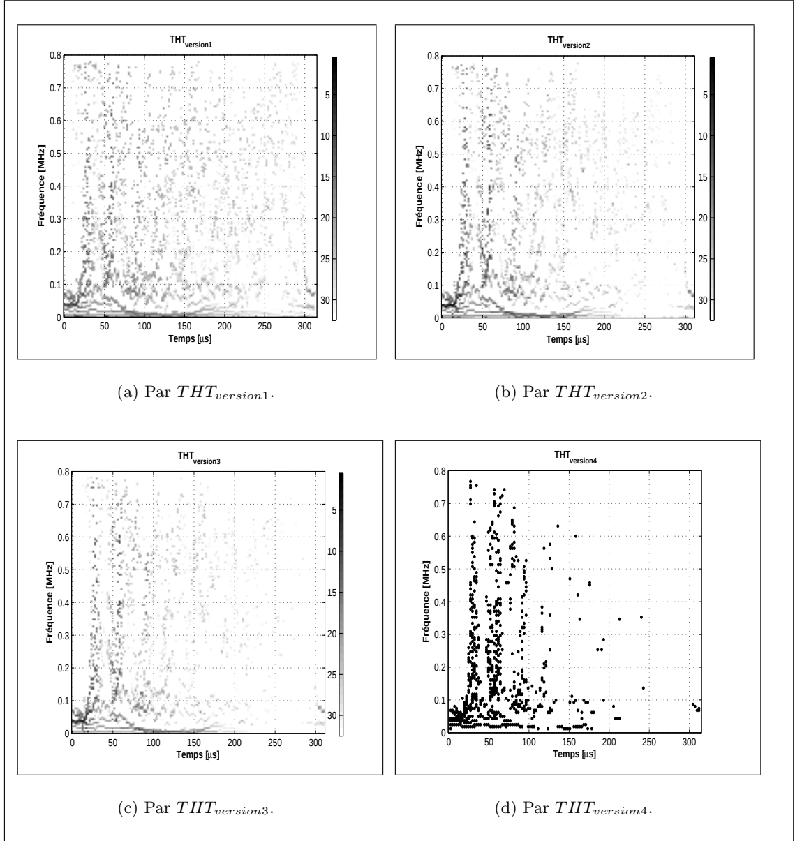
Figure VI.9 — Descriptions temps-fréquence pour les différentes versions de la THT d'un écho d'une sphère pleine en Nickel-Molybdène ( a = 15mm , c_l = 5554m/s , c_t = 3021m/s , \rho = 9217kg/m^3 ) (signal décrit par la RTF de la figure VI.2(b)).
