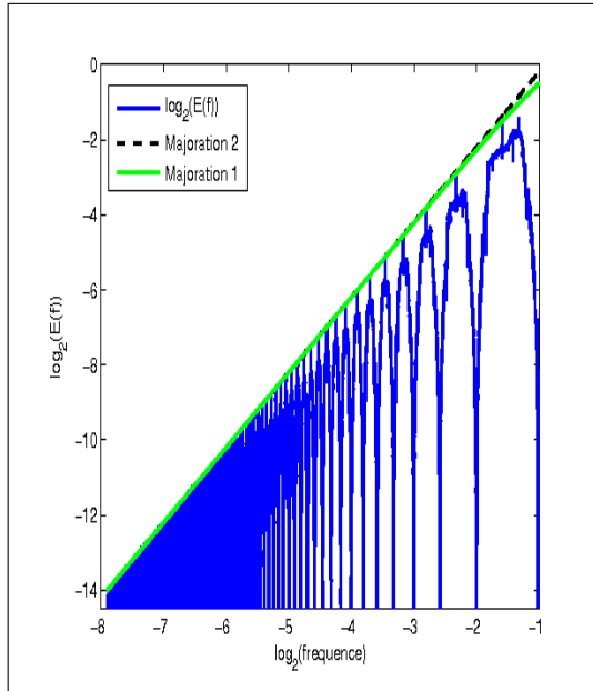
(c) Modélisation de : \text{Max}(\log_2(E(\nu))) .
