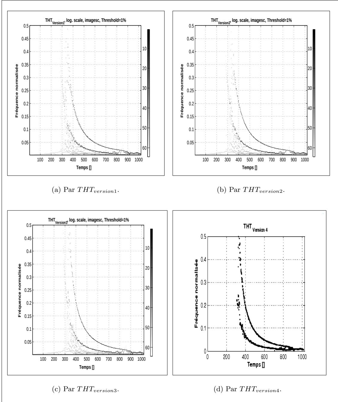
Figure V.8 — Description temps-fréquence d'un signal composé de deux « chirps hyperboliques » par les quatre versions de la THT.
