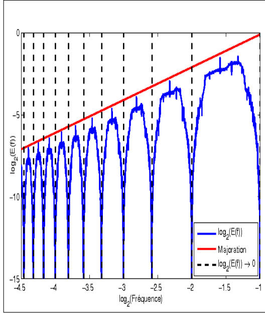
(a) Estimation de E(\nu) dans le plan (\log_2 - \log_2) .
