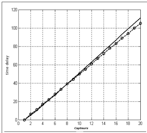
(c) Estimation des retards sur la ligne de capteurs par T_{B_\Psi} et T_{B_{theo}} .
