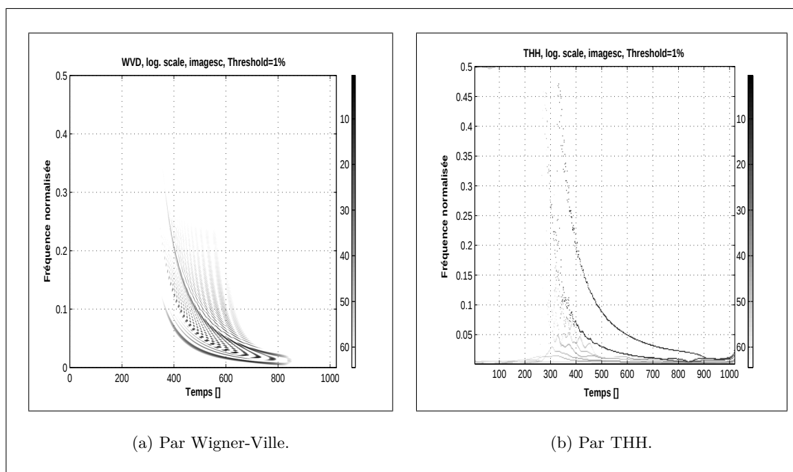
Figure II.19 — Comparaison des représentations temps-fréquence d'un signal constitué de deux chirps hyperboliques obtenues par WVD et par THH.
