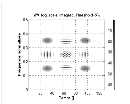
(c) Wigner-Ville.
