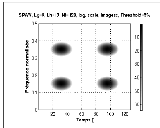
(d) Pseudo Wigner-Ville lissée.
