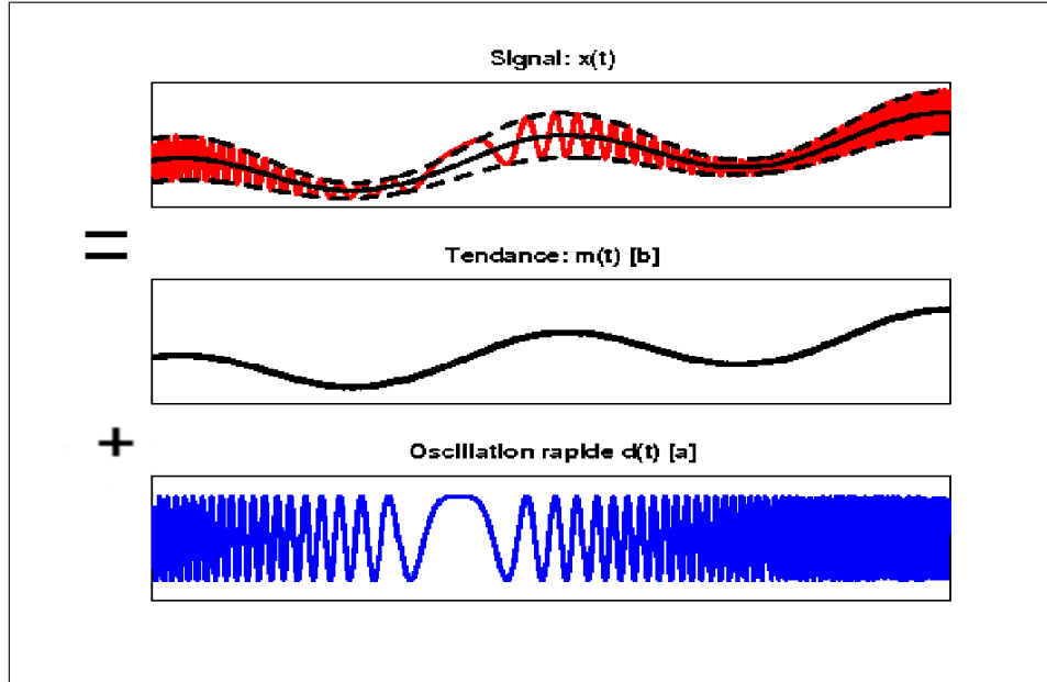
Figure II.1 — Principe de l'EMD : « oscillation rapide » (a) + « oscillation lente » (tendance) (b).
