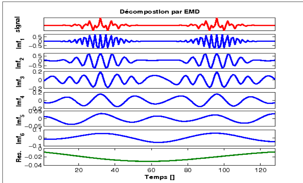
(a) Décomposition par EMD.
