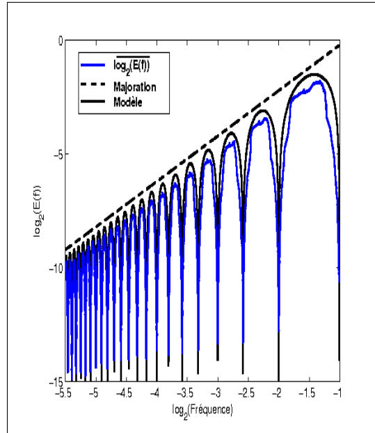
(d) Modélisation parabolique de \log_2(E(\nu)) .
