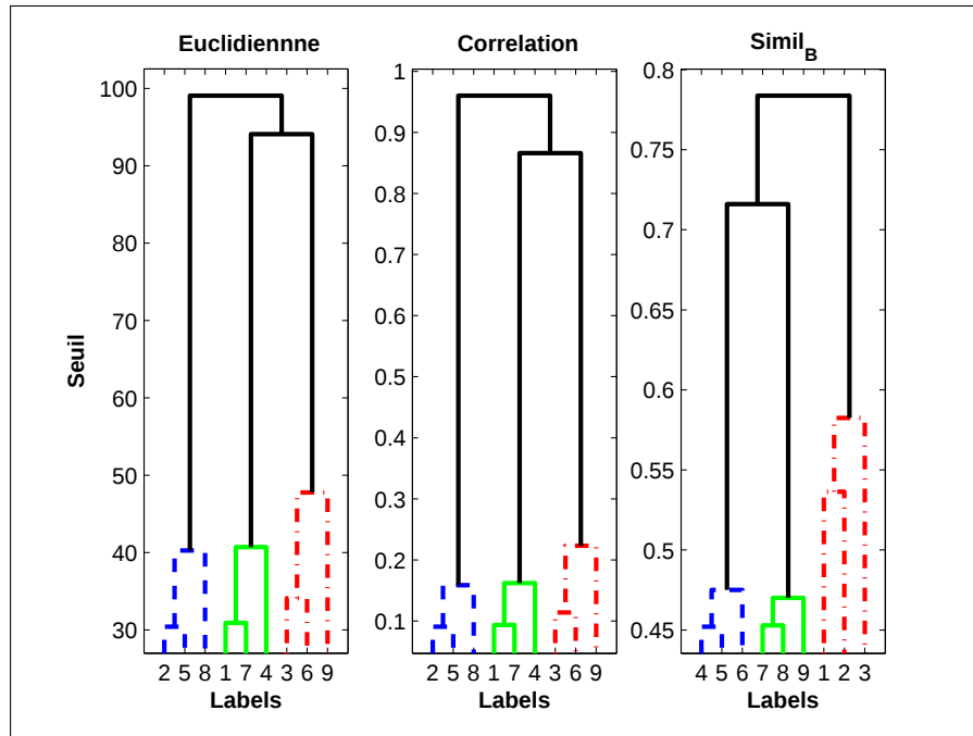
Figure IV.7 — Comparaison de la coalescence par Simil_B , DE et CC. Les labels (1, 2, 3), (4, 5, 6) et (7, 8, 9) correspondent respectivement aux classes Cylinder, Bell et Funnel.
