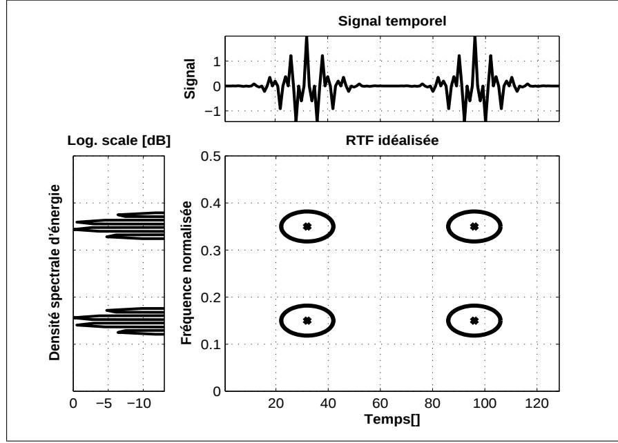
Figure I.5 — Représentations (temps, fréquence, RTF idéalisée) du signal avec quatre atomes gaussiens élémentaires.
