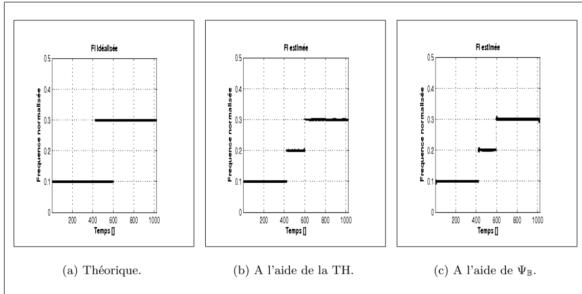
Figure V.1 — Estimation de FI d'un signal multi-composantes à l'aide de \Psi_B et comparaison avec la TH.
