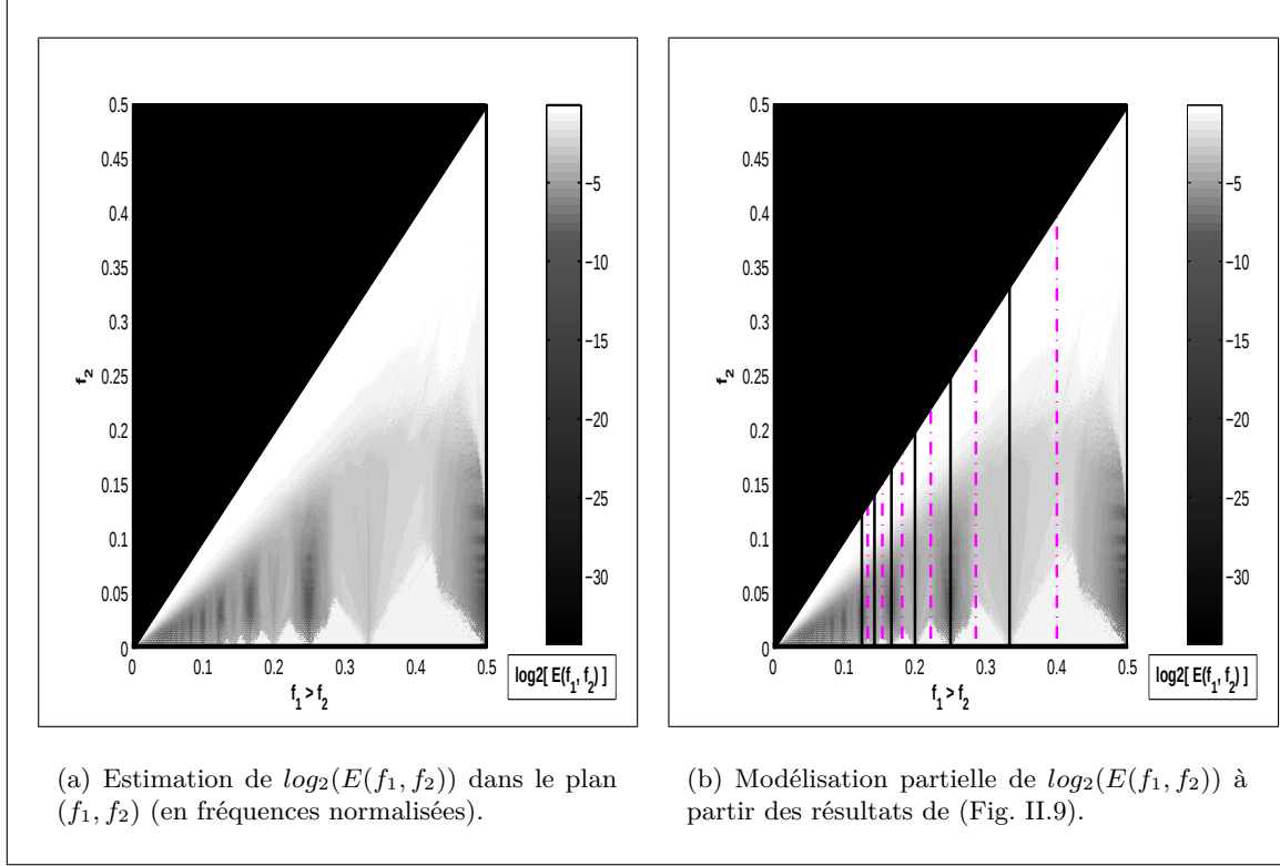
Figure II.11 — Estimation et comportement de l'erreur E(f_1, f_2) associé aux deux premières IMF du signal à 2 « tones ».
