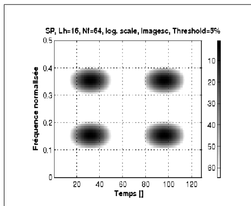
(a) Spectrogramme.
