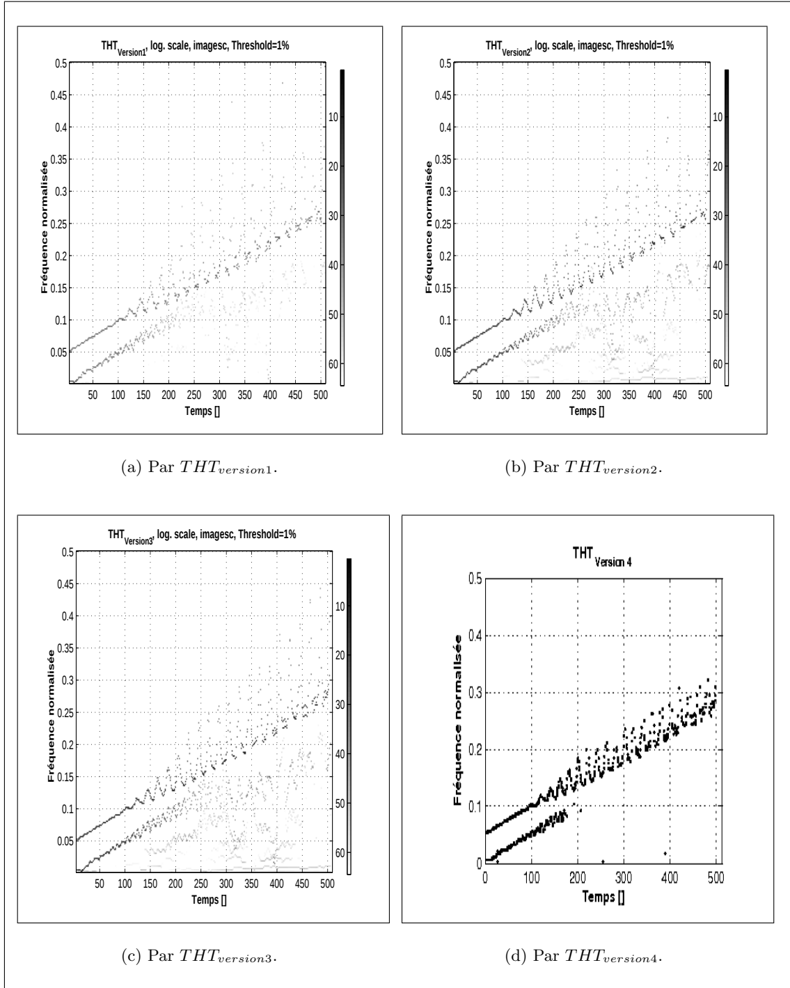
Figure V.7 — Description temps-fréquence d'un signal composé de deux chirps linéaires parallèles par les quatre versions de la THT.
