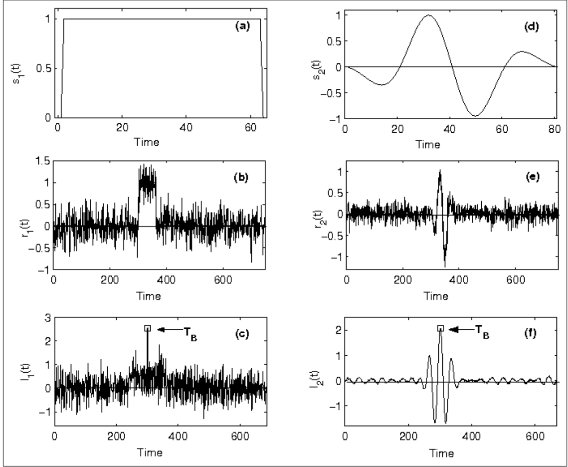
Figure IV.9 — Résultats de détection par M\mathbb{B}F des signaux synthétiques simples ( a = 0.95 , t_0 = 300 ) : (a) Premier signal d'émission, s_1(t) , (b) Écho reçu du premier signal, r_1(t) , (c) Intégrale I , de \Psi_{\mathbb{B}_d} calculée entre le signal émis s_1(t) et l'écho reçu r_1(t) , (d) Second signal d'émission, s_2(t) , (e) Écho reçu du second signal, r_2(t) , (f) Intégrale I , de \Psi_{\mathbb{B}_d} calculée entre le signal émis s_2(t) et l'écho reçu r_2(t) .
