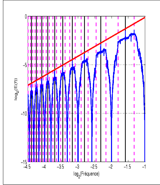
(b) Modélisation de : \log_2(E(\nu)) \rightarrow 0 .
