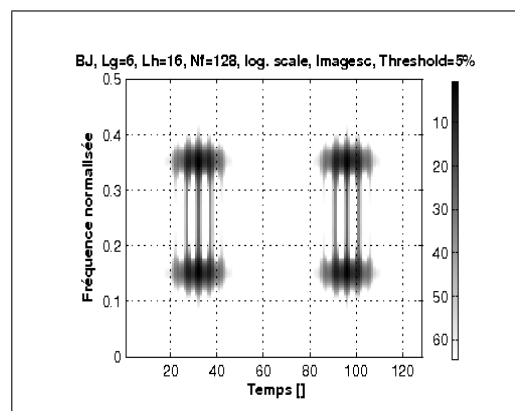
(f) Born-Jordan.
