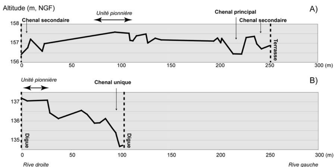
Figure 3.15 – Exemple de profil en travers, A) dans la zone en tresses, B) dans la zone endiguée de la basse vallée de la Drôme
