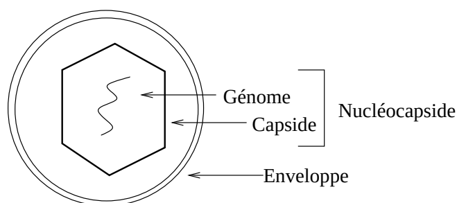
FIG. 4.2 – Virus enveloppé
