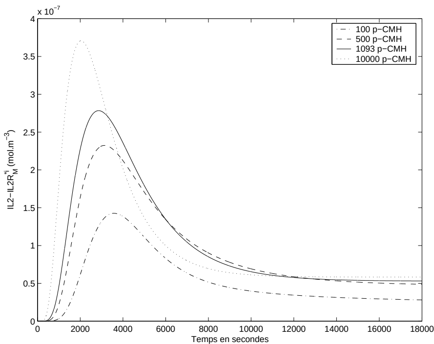
FIG. 11.10 – Concentration de IL2-IL2R M *i pour différentes valeurs de [L]
