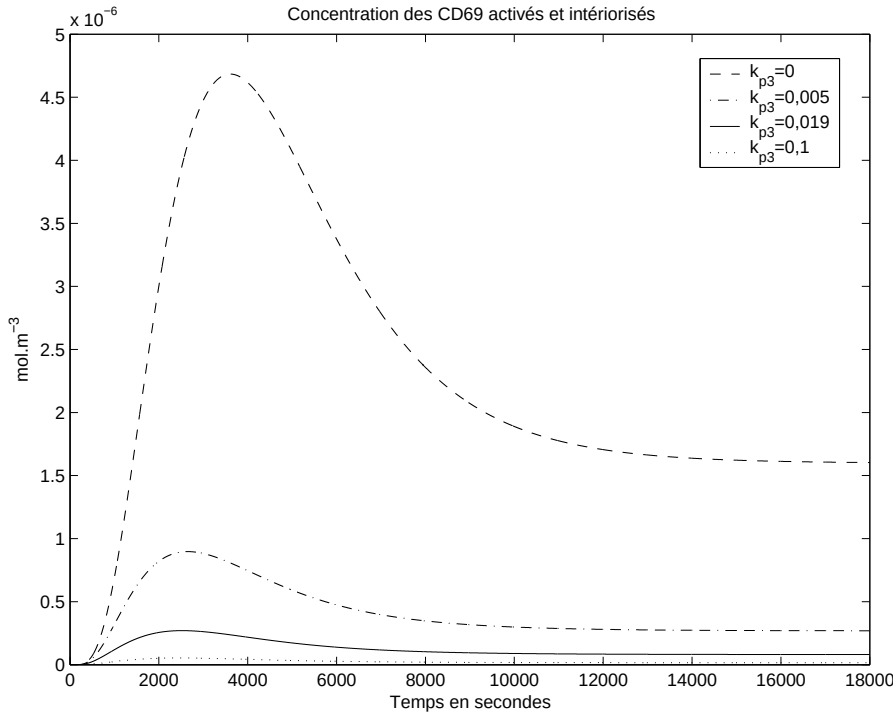
FIG. 11.6 – Concentration de CD69^{*i} pour différentes valeurs de k_{p3}
