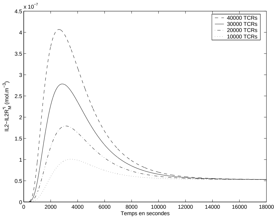
FIG. 11.14 – Concentration de IL2-IL2R M *i pour différentes valeurs de \text{TCR}(t=0)
