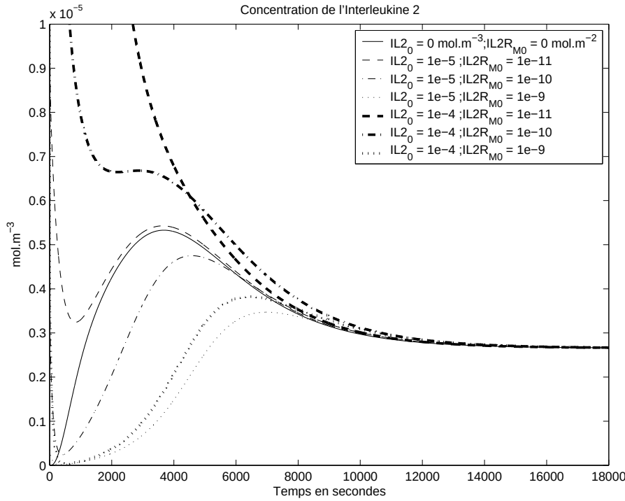
FIG. 11.21 – [IL2] pour différentes concentrations d'IL2 et d'IL2R M au départ
