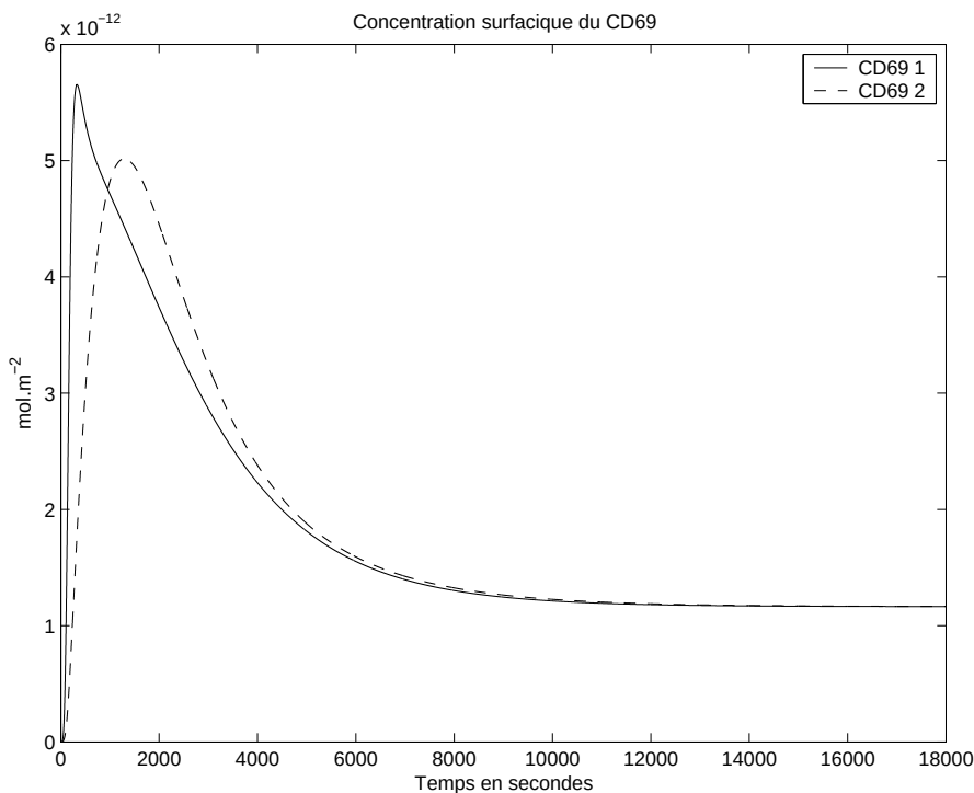
FIG. 10.8 – Concentration de \text{CD69} - 15 ou 22 équations
