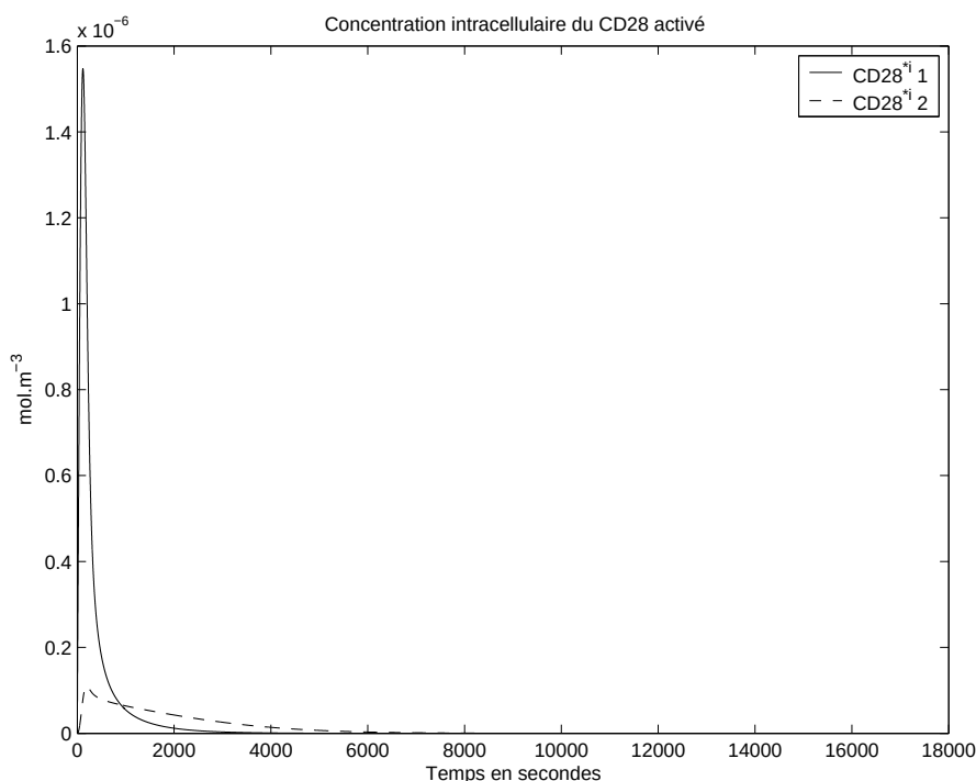
FIG. 10.7 – Concentration de \text{CD28}^{*i} - 15 ou 22 équations
