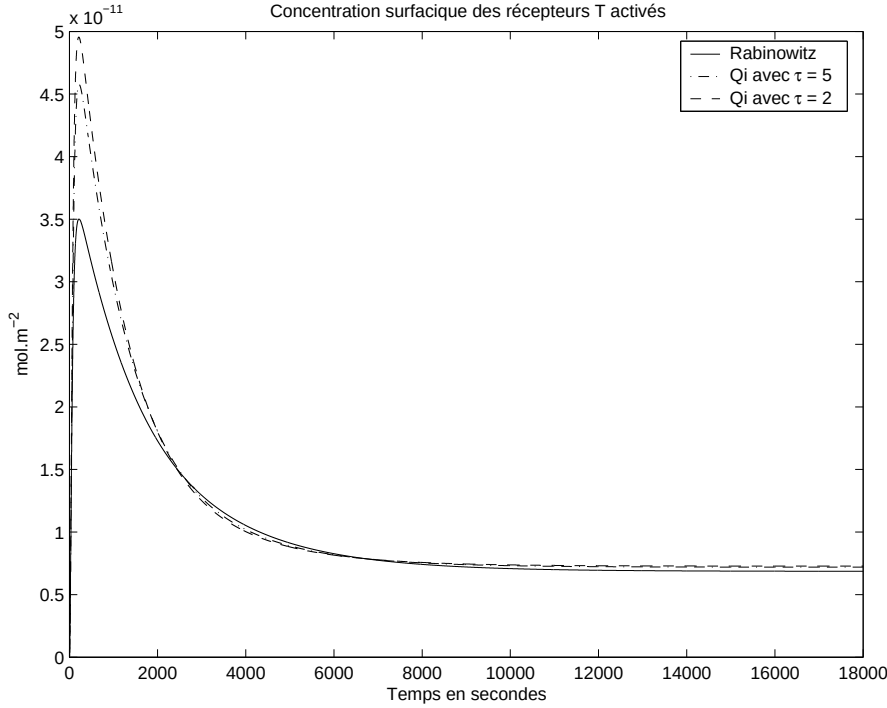
FIG. 11.4 – Concentration en T^* pour différentes valeurs de k_{a1} et k_{offTL}
