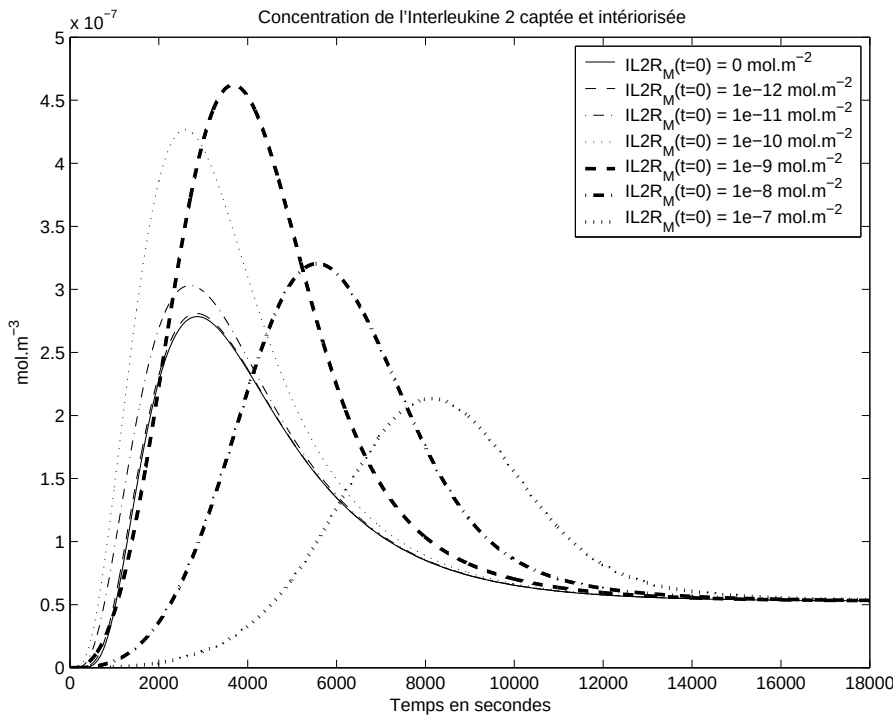
FIG. 11.20 – [IL2 - IL2R_M^*] pour différentes concentrations d' IL2R_M au départ
