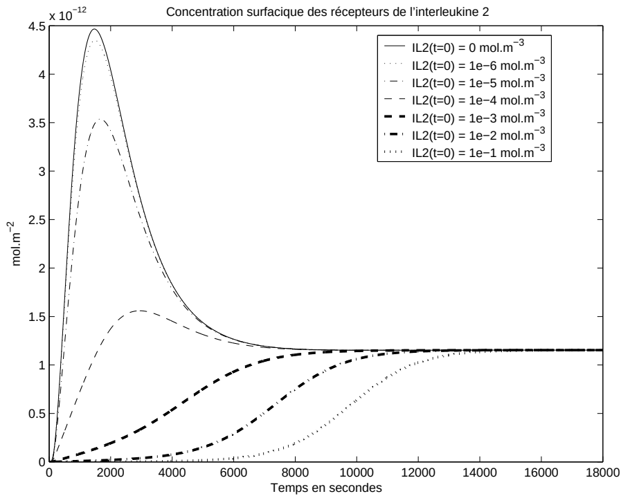
FIG. 11.16 – [IL2R_M] pour différentes concentrations d'IL2 au départ
