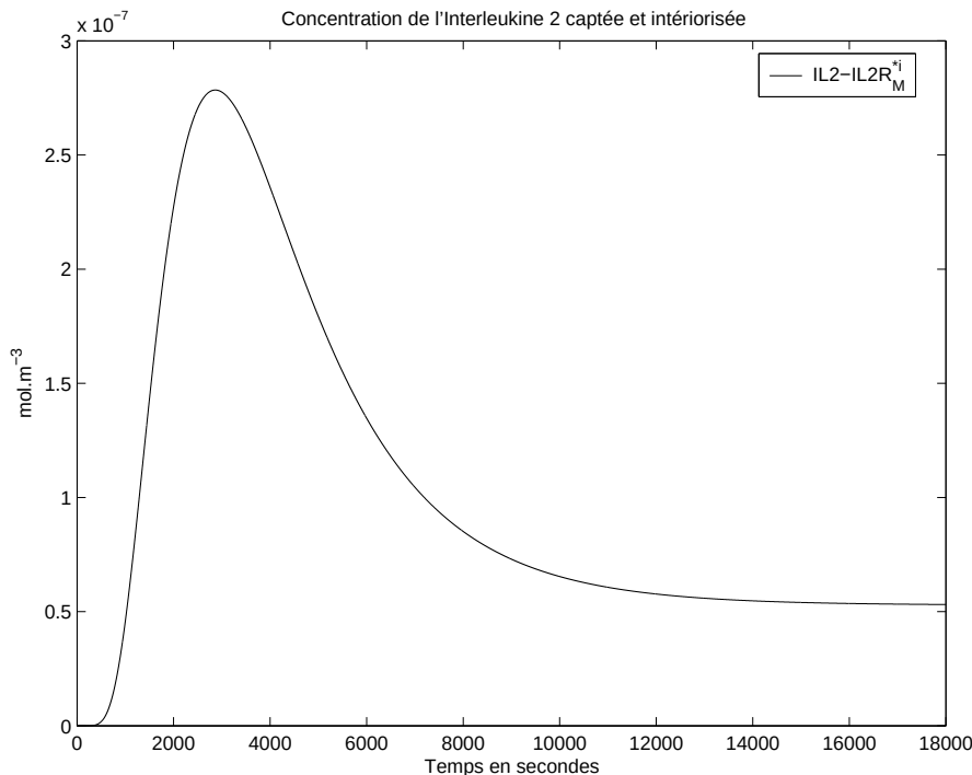
FIG. 10.5 – La concentration en complexe d'interleukine 2 captée et intériorisée pendant 5 heures
