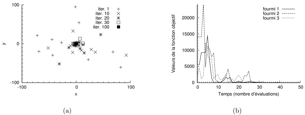
FIG. 3.16 – L'algorithme HCIAC optimisant la fonction B_2 . (a) positions x et y des 10 fourmis à différentes étapes de l'optimisation, (b) valeurs de la fonction objectif trouvées par 3 fourmis durant les 50 premières évaluations.
