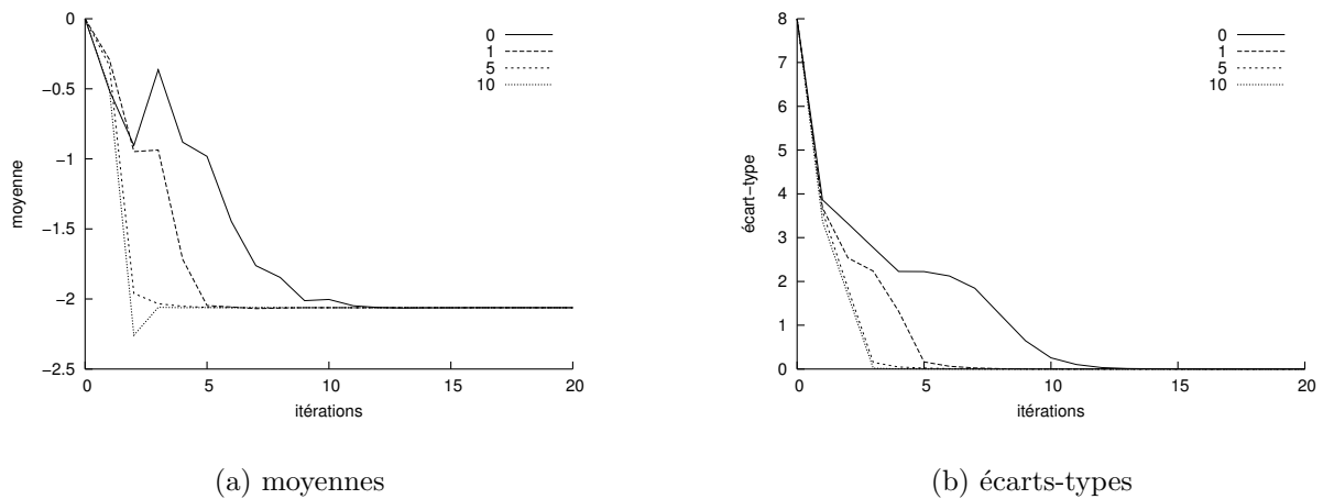
FIG. 4.8 – Évolution de la moyenne et de l'écart-type de la population dans CHEDA_{sn} , pour différentes valeurs de \nu ; sur le problème Dreo1 .
