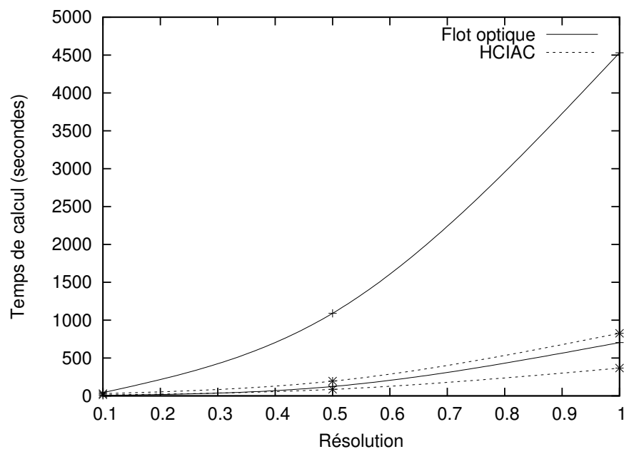
FIG. 5.5 – Comparaison des temps de calcul (en secondes) pour les deux méthodes d'optimisation, les temps minimums et maximums sont indiqués en traits pointillés.
