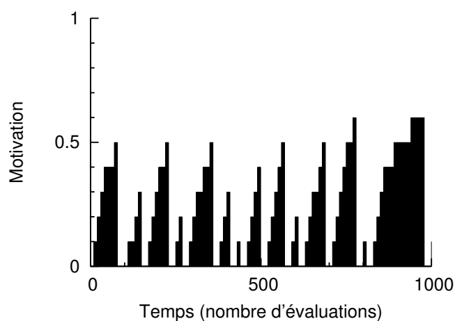
FIG. 3.13 – Dynamique du paramètre de motivation pour une fourmi (le seuil est ici de 0.5).
