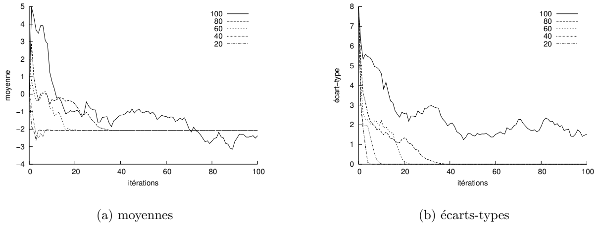
FIG. 4.7 – Évolution de la moyenne et de l'écart-type de la population dans CHEDA_s , pour différentes valeurs de \beta , sur le problème Dreo1 .
