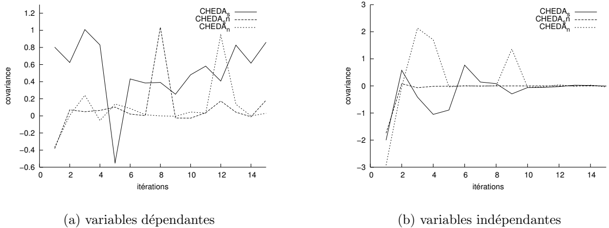
FIG. 4.5 – Évolution de la covariance de la population pour chaque variante, sur les problèmes Rosenbrock ( R_2 ) et B_2 (à deux dimensions).
