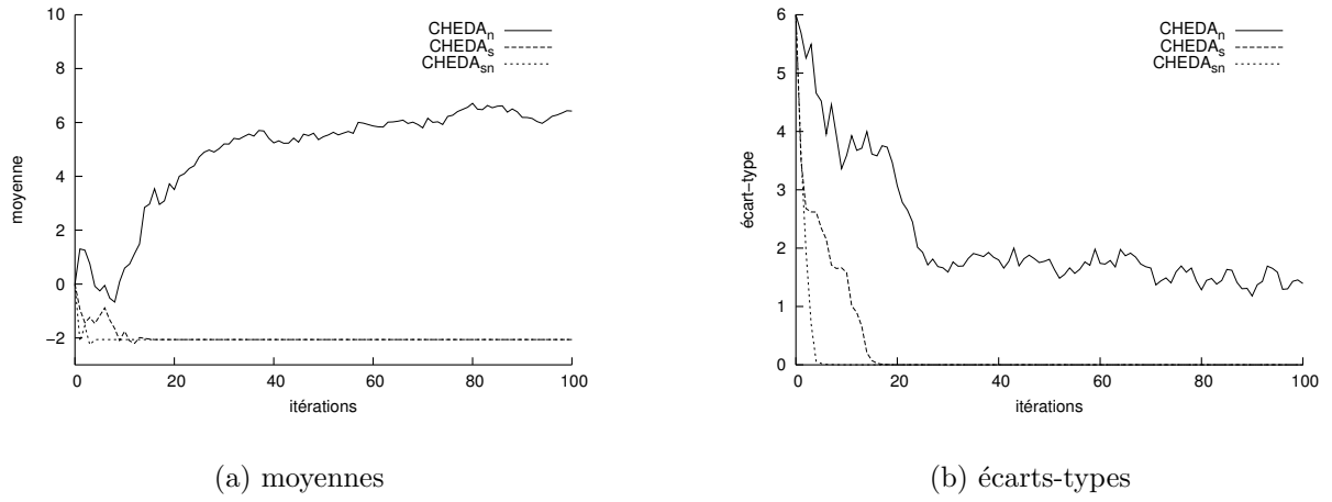
FIG. 4.3 – Évolution de la moyenne et de l'écart-type de la population pour chaque variante, sur le problème Dreot1.
