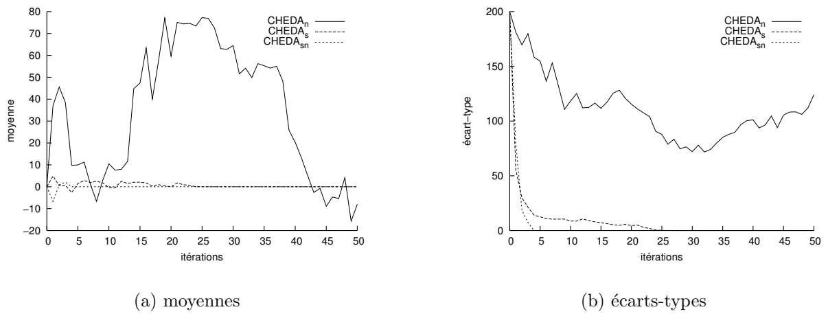
FIG. 4.4 – Évolution de la moyenne et de l'écart-type de la population pour chaque variante, sur le problème Griewangk (à une dimension).
