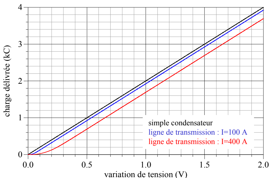
Figure 4.4.a : Charge électrique en fonction de la variation de tension ( C = 2000 F , R = 1 m \Omega )
