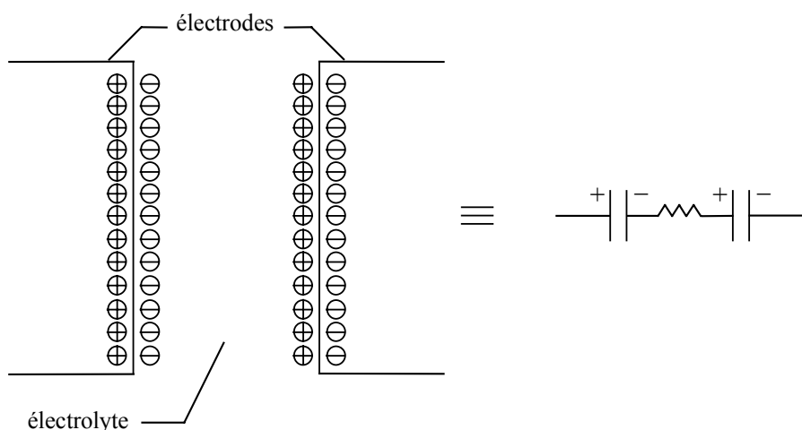
Figure 1.3 : Principe de développement des supercondensateurs
