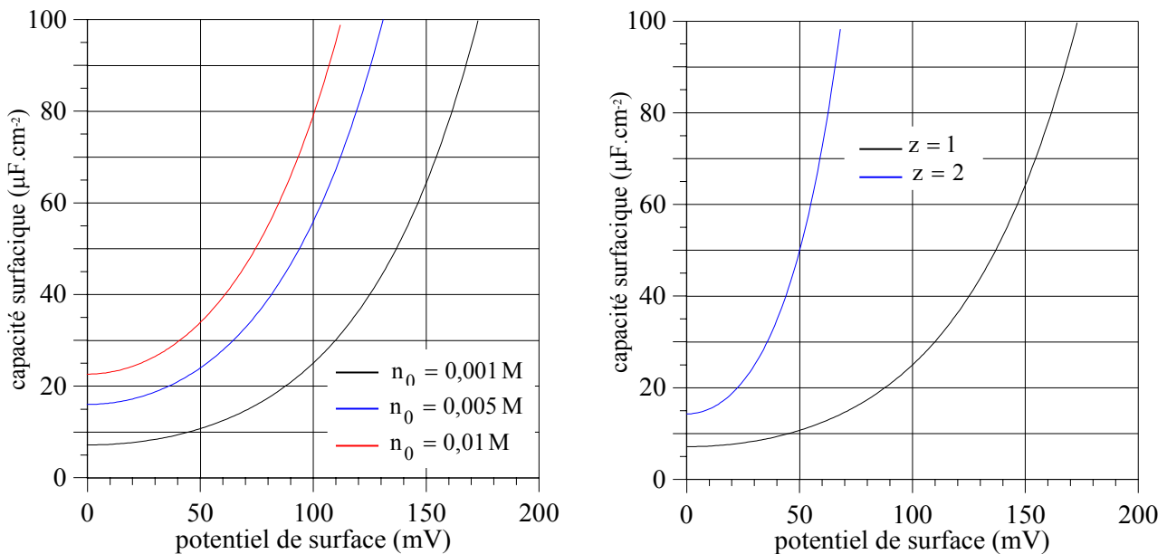
Figure 2.12 : Capacité surfacique (à gauche : z = 1 , à droite : n_0 = 0,001 \text{ M} )
