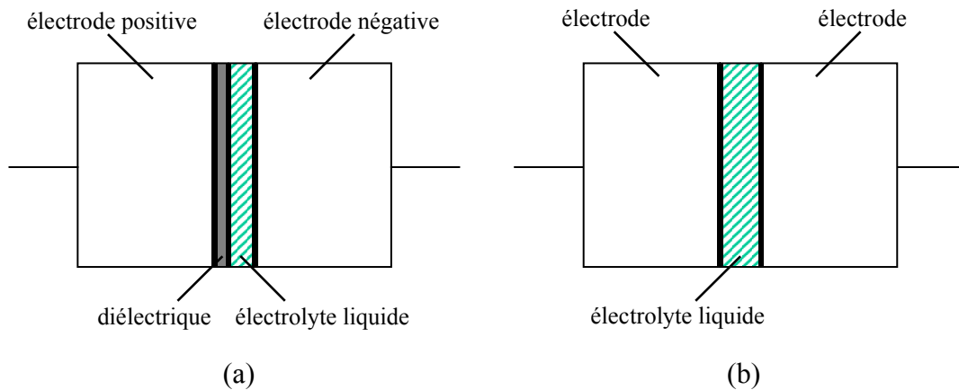
Figure 1.2 : Condensateur électrolytique (a) et supercondensateur (b)
