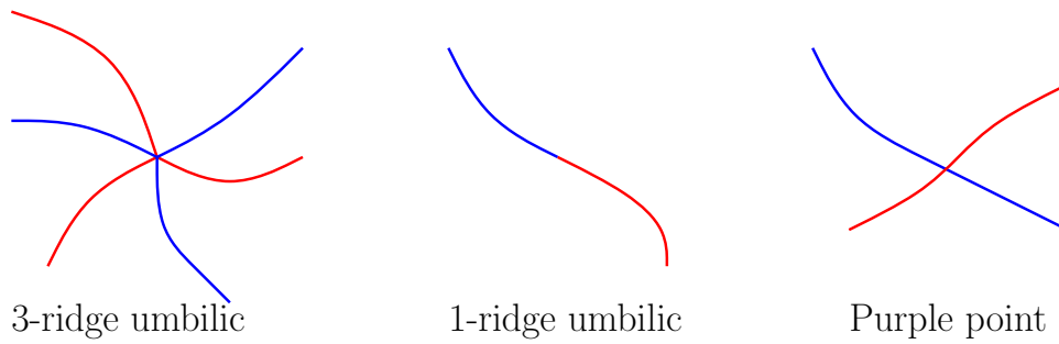
Figure 2.11: Singularités de la courbe des ridges: les courbes rouges et bleues différencient les extrêmes des deux courbures principales. (à gauche et au milieu) Il y a deux types d’ombilics traversés par une ou trois branches de ridges, chacune changeant de couleur à l’ombilic. (à droite) Le croisement d’un ridge bleu et d’un ridge rouge est appelé point purple .
