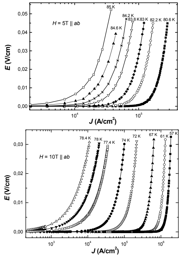
Figure V. 4 : Quelques caractéristiques E(J) de films minces YBa 2 Cu 3 O 7-δ pour différentes températures, les valeurs sont représentées sur les courbes, à deux champs magnétiques extérieurs ( H = 5 \text{ T} et 10 \text{ T} ) parallèles aux plans ab .
