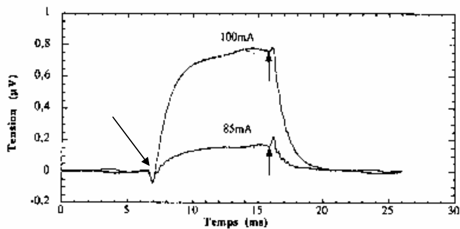
Figure II. 12 : Exemples de signaux d'un film mince d' \text{YBa}_2\text{Cu}_3\text{O}_{7-\delta} en réponse à deux impulsions de courant I_m = 85 \text{ mA} et 100 \text{ mA} ( T = 75 \text{ K} , H = 0 \text{ T} ).
