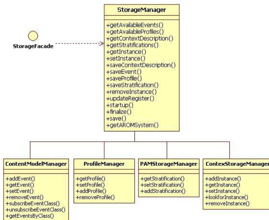
Figure 83. Les classes qui composent la gestion de connaissances du canevas BW- \mathcal{M} .
