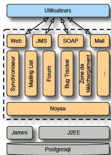
Figure 90. Structure de la plate-forme LibreSource (d'après [Forest 2005b]).
