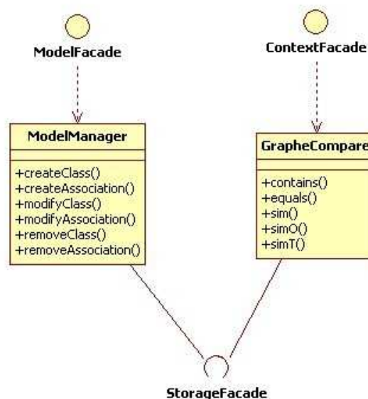
Figure 81. Classes participant à la gestion du modèle.
