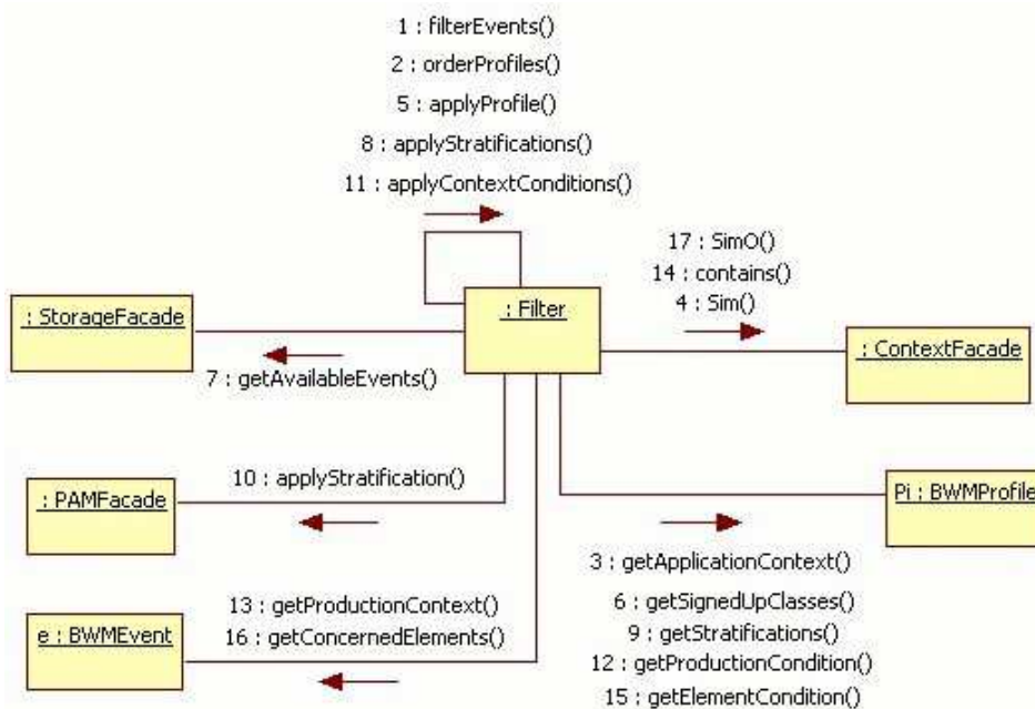
Figure 72. Collaborations mises en œuvre durant la seconde étape du processus de filtrage.
