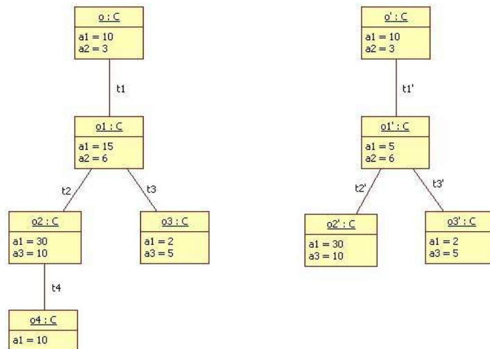
Figure 42. Exemple d'instances qui peuvent être comparées à travers l'opérateur contains
