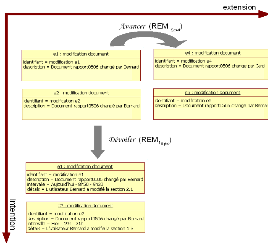
Figure 61. Exemple de l'application des opérations sur les stratifications en extension et en intention.
