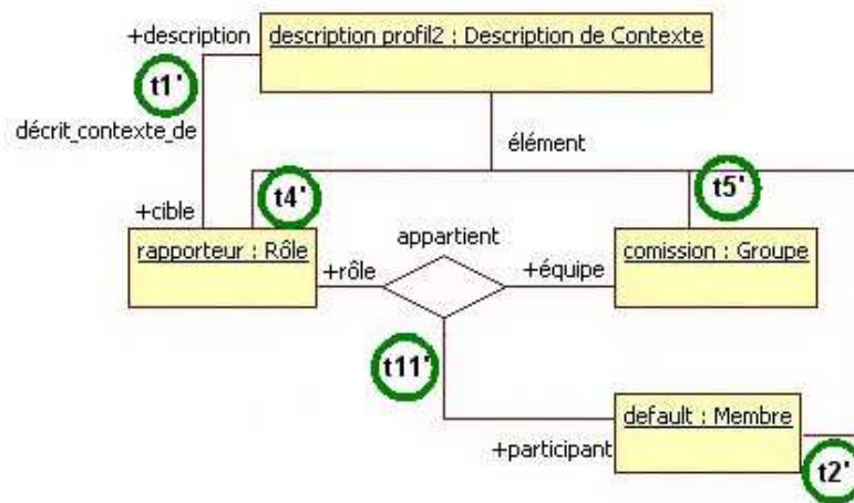
Figure 41. Exemple d'une description de contexte pour une situation générale d'un rôle dans un groupe donné 82 .
