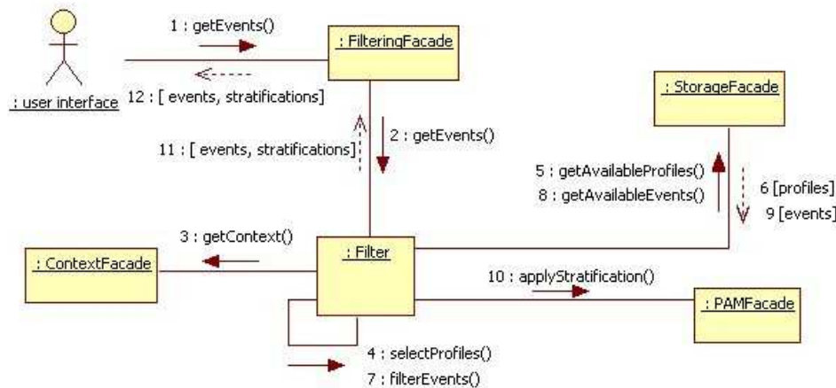
Figure 70. Diagramme de collaboration résumant le filtrage des événements.
