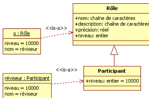
Figure 33. Exemple de deux objets du modèle de contexte comparés à l'aide de l'opérateur equals .
