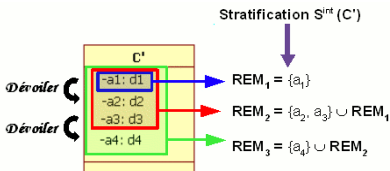
Figure 48. Exemple de stratification intensionnelle sur une classe.
