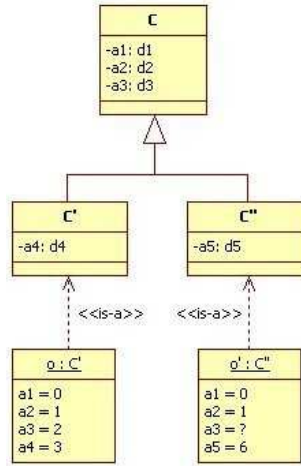
Figure 32. Exemple de deux objets qui peuvent être comparés par l'opérateur equals .
