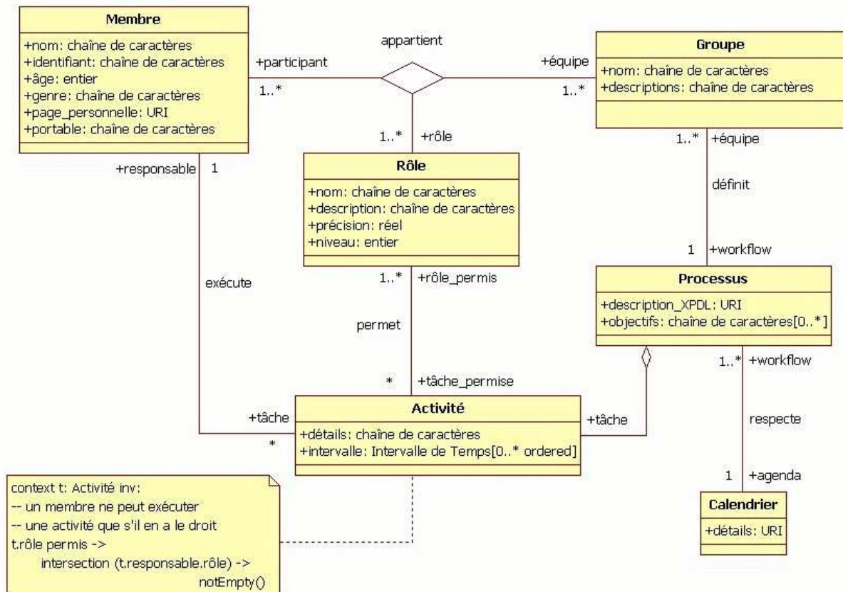
Figure 18. Les classes et les relations concernant l'utilisateur et le groupe.
