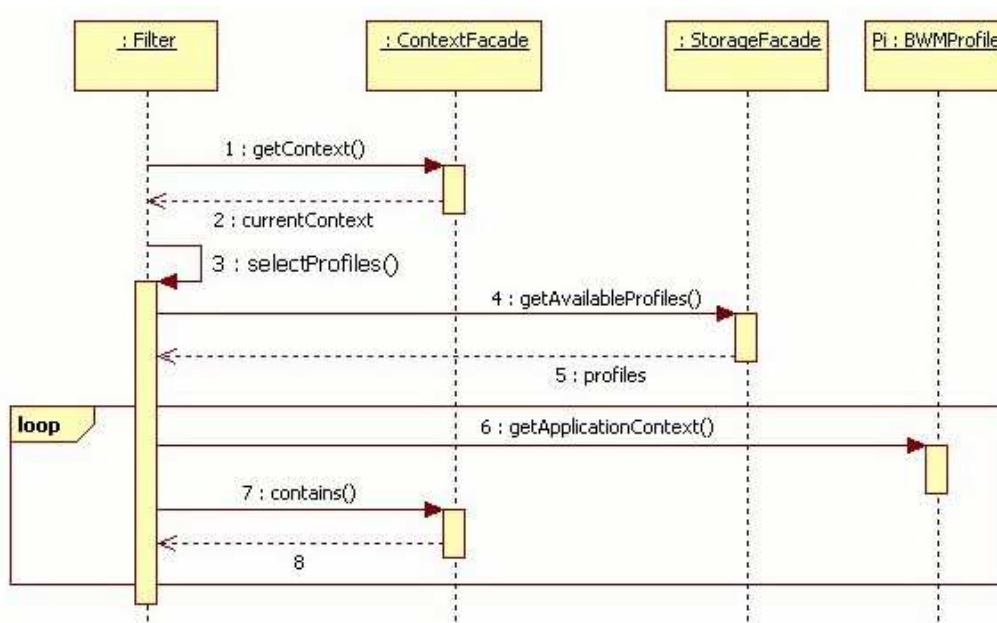
Figure 71. Diagramme de séquence mettant en évidence les collaborations qui ont lieu durant la sélection des profils.
