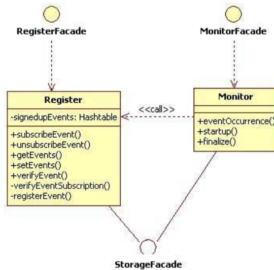
Figure 66. Classes composant le moniteur.
