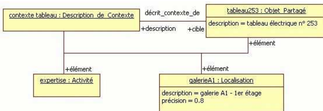
Figure 25. Exemple d'utilisation du modèle pour l'expression des informations contextuelles liées à un objet partagé.
