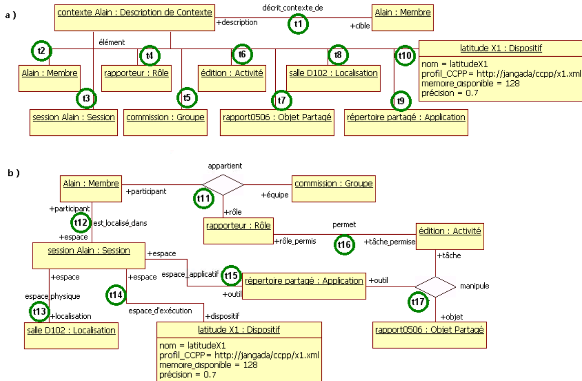
Figure 40. Instances (objets et tuples) présentes dans le graphe décrit par un objet de la classe Description de Contexte lié à un utilisateur en particulier 81 .
