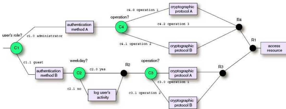
Figure 10. Exemple de graphe contextuel pour un problème de politique de contrôle d'accès à une ressource (d'après [Mostéfaoui 2004]).
