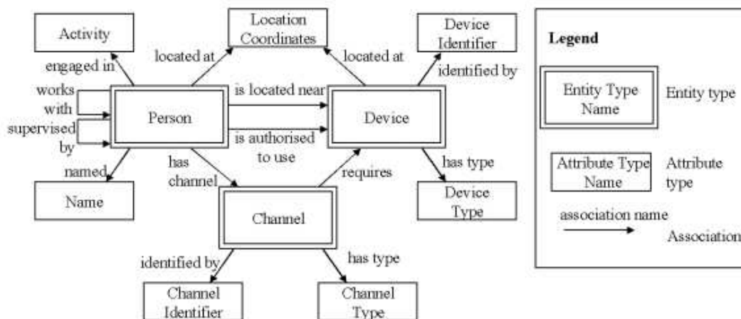
Figure 11. Exemple de représentation de contexte de Henricksen et al. [Henricksen 2002].
