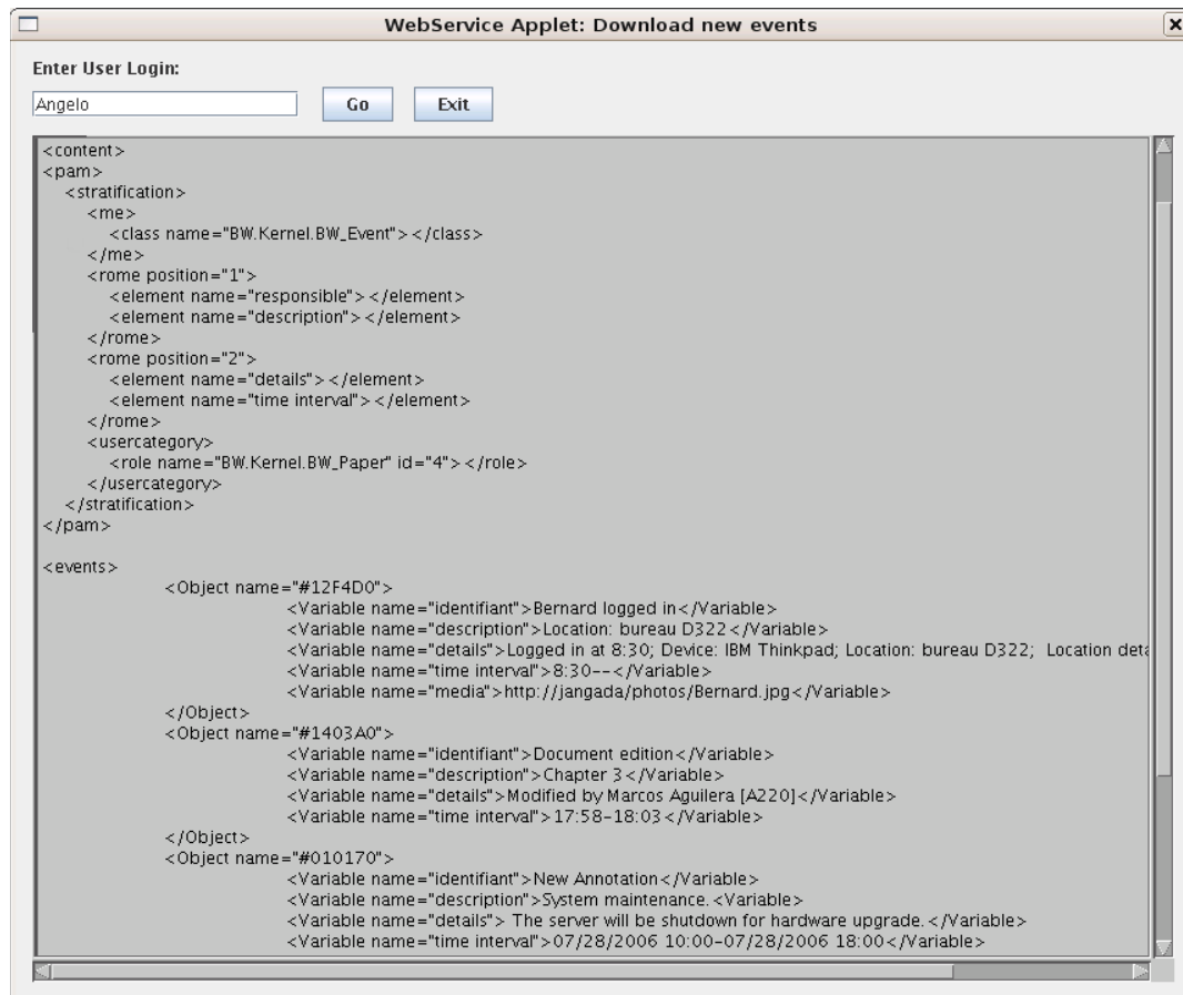
Figure 89. Exemple de retour de l'appel getEvents au service Web BW- \mathcal{M} .
