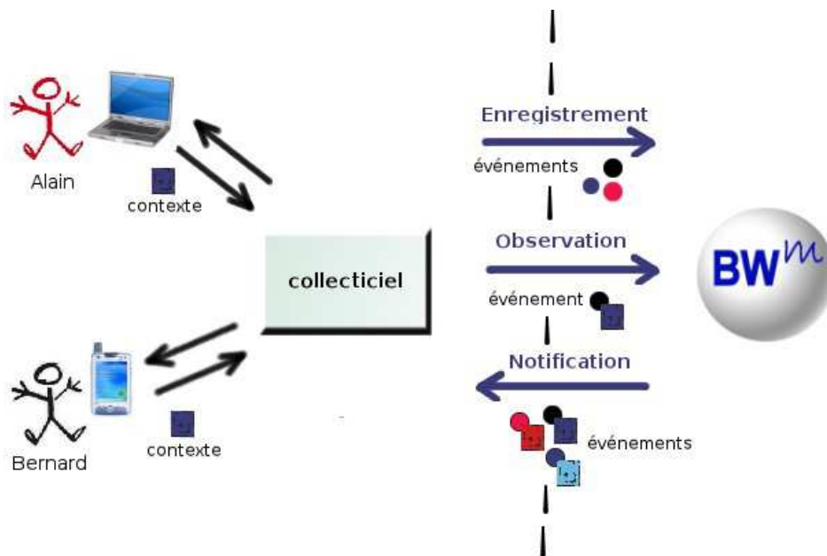
Figure 63. Les phases de fonctionnement du canevas BW-M .
