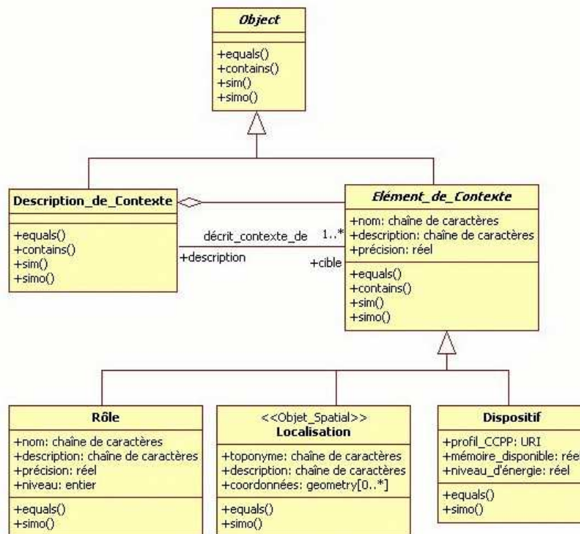
Figure 35. Les opérations proposées vues dans le modèle UML.
