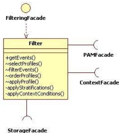
Figure 69. Éléments du canevas BW- \mathcal{M} intervenant sur le filtrage des événements.
