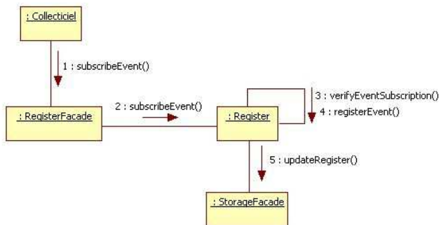
Figure 67. Processus d'enregistrement d'une nouvelle classe d'événement.
