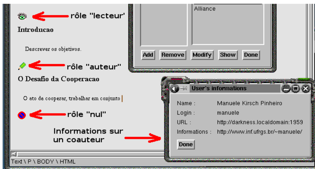
Figure 8. Indicateurs des rôles effectifs dans l'éditeur AllianceWeb.
