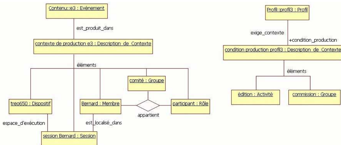
Figure 58. Comparaison entre le contexte dans lequel un événement a été produit et une condition de production sur un profil.
