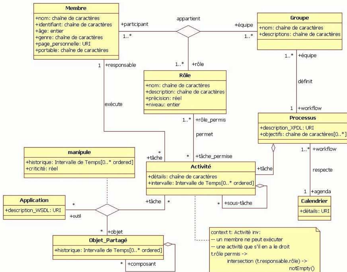
Figure 20. Les éléments qui composent le contexte collaboratif.
