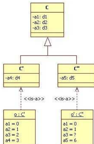
Figure 32. Exemple de deux objets qui peuvent être comparés par l'opérateur equals .
