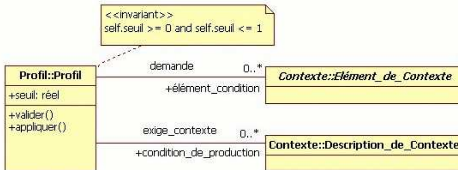
Figure 53. Conditions contextuelles établies par les profils.
