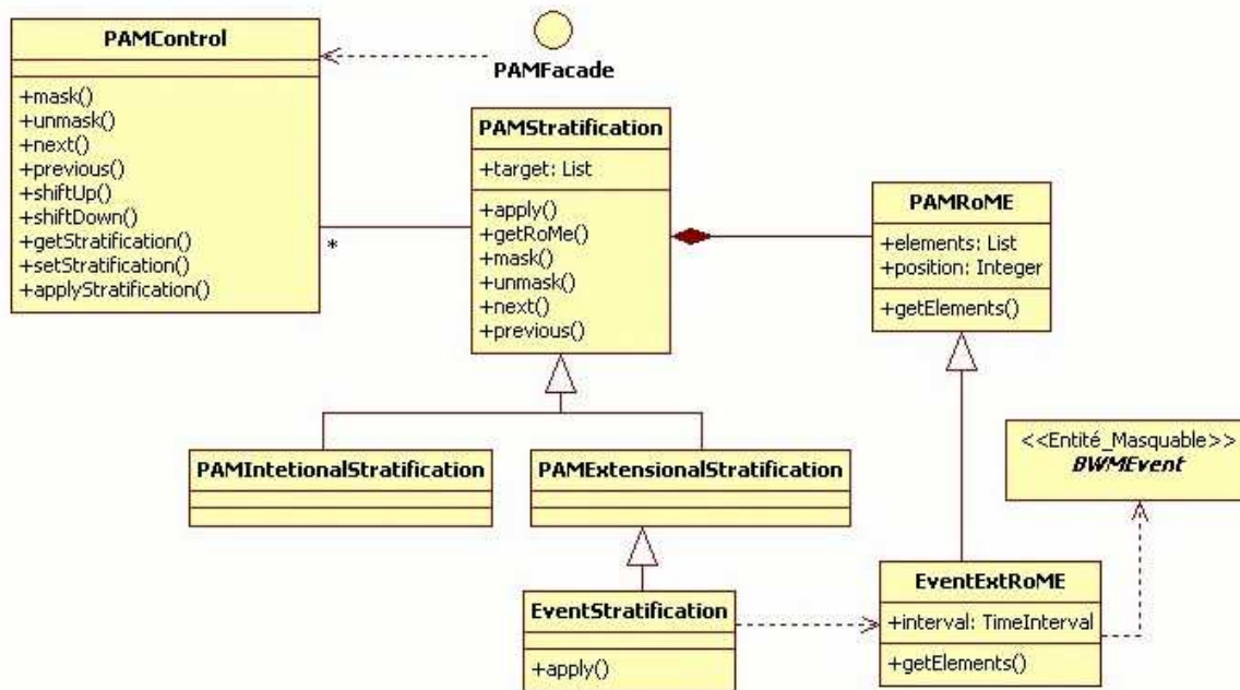
Figure 74. Implémentation du modèle d'accès progressif.
