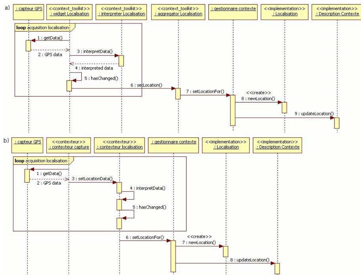
Figure 28. Diagrammes de séquence qui illustrent deux possibilités pour le processus d'acquisition de la localisation.
