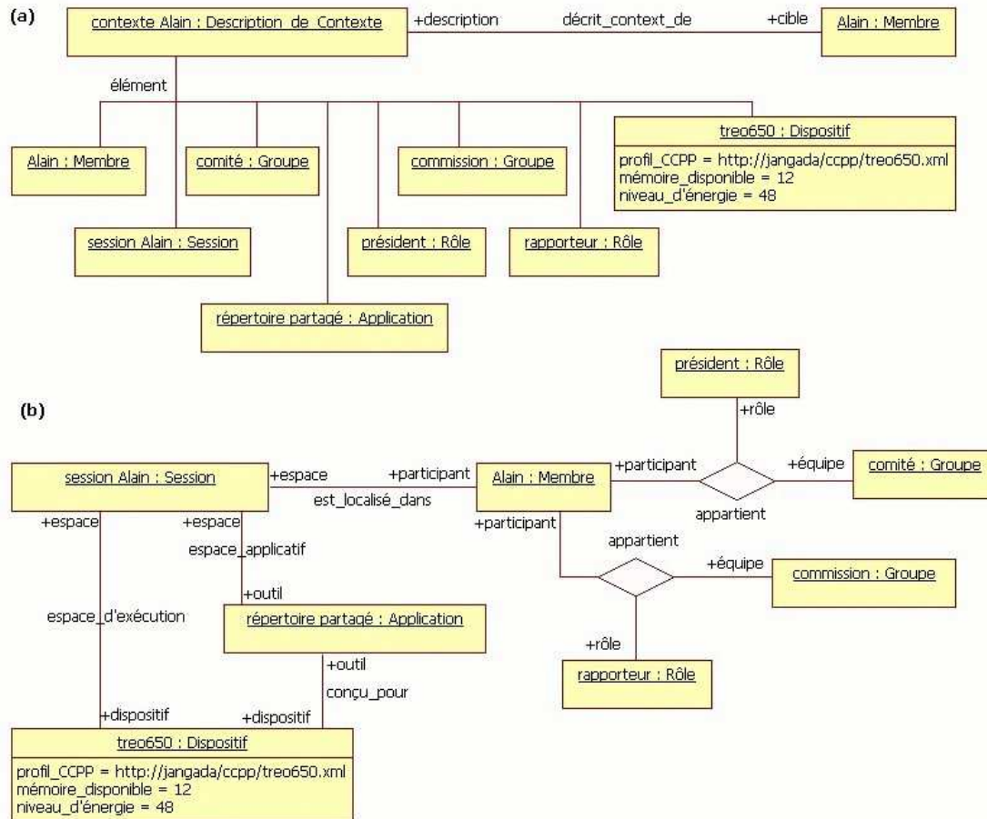
Figure 24. Contexte de l'utilisateur Alain suite à un déplacement. En (a) les éléments qui composent la description de contexte, et en (b) leurs relations.
