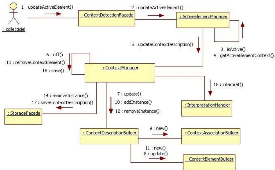
Figure 79. Diagramme de collaboration présentant un exemple de mise à jour du contexte courant d'un élément actif.
