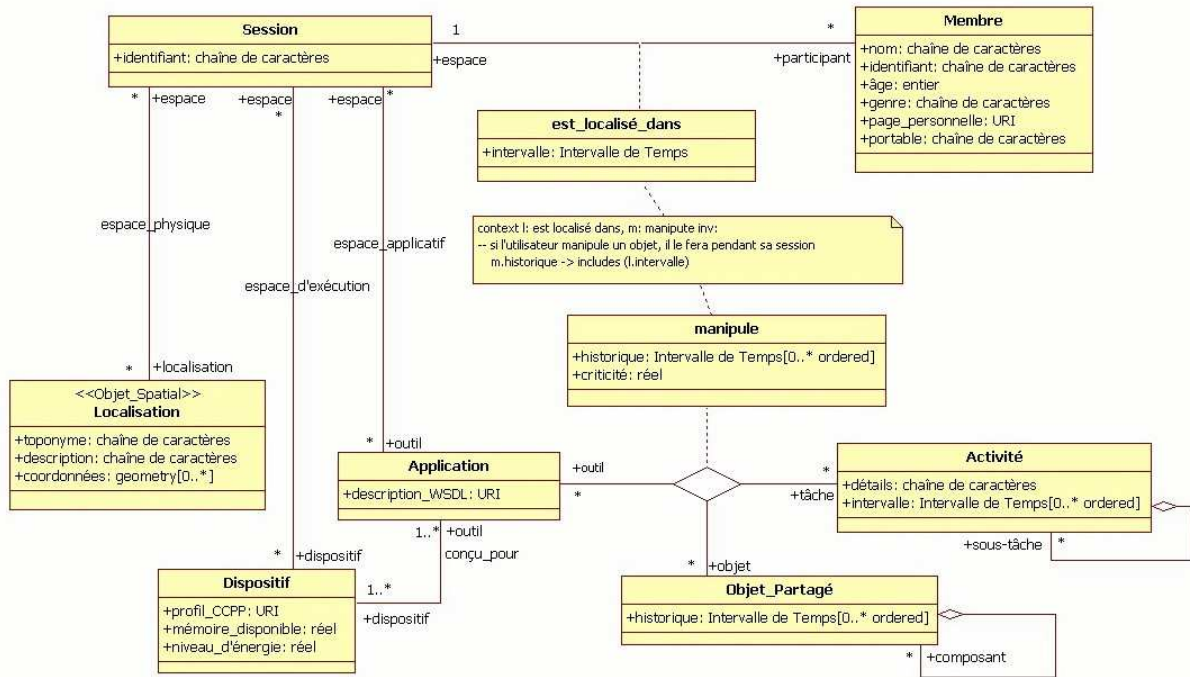
Figure 21. Le contexte physique, ses éléments et les relations qu'ils entretiennent.
