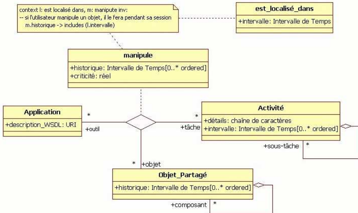
Figure 19. Relations entre la classe Objet_Partagé et les classes Activité et Application .
