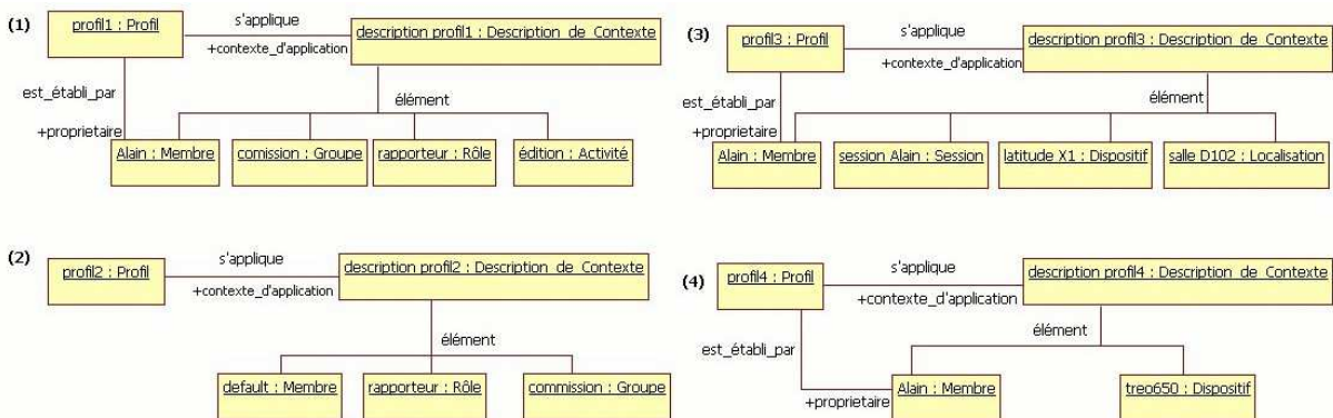
Figure 56. Les contextes d'application associés aux profils disponibles pour un utilisateur donné 87 .
