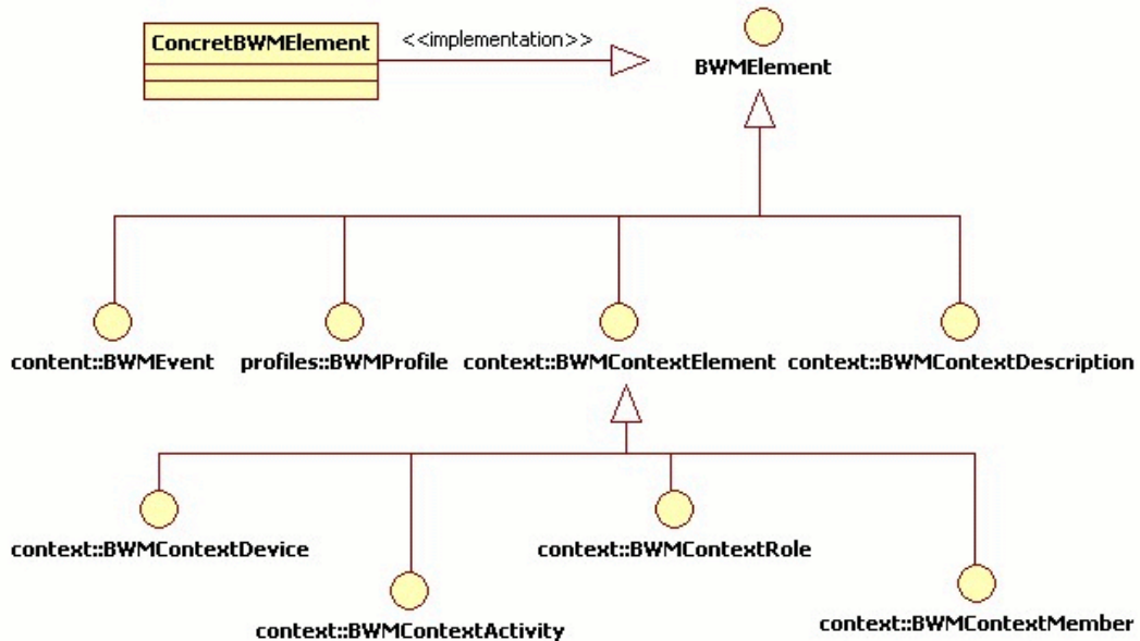
Figure 85. Contenu du paquetage kernel.
