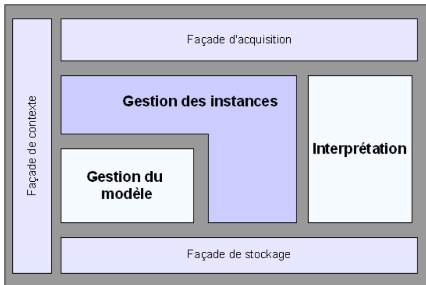
Figure 75. Éléments de l'unité de gestion de contexte du canevas BW- \mathcal{M} .
