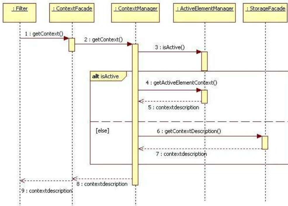
Figure 80. Diagramme de séquence illustrant une requête émanant de la sous-unité de filtrage.
