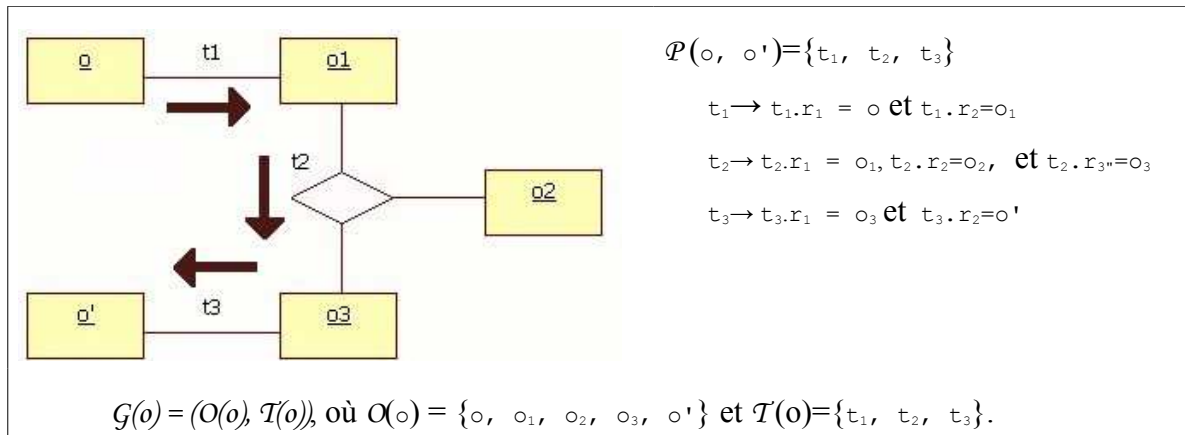
Figure 39. Exemple de chemin liant deux objets o et o' .
