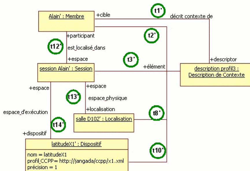
Figure 43. Description de Contexte décrivant une situation où l'utilisateur Alain se trouve dans la salle de réunion et utilise son ordinateur portable (les tuples sont énumérés pour une meilleure identification).
