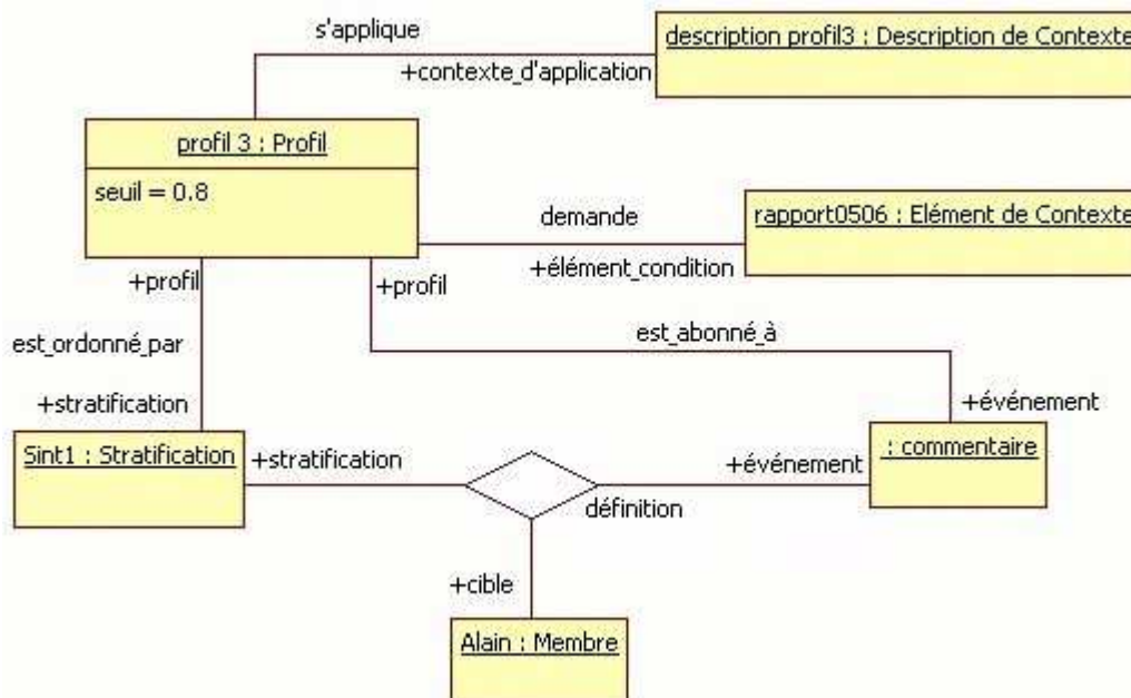
Figure 54. Exemple de profil défini pour l'utilisateur Alain comptant une condition contextuelle.
