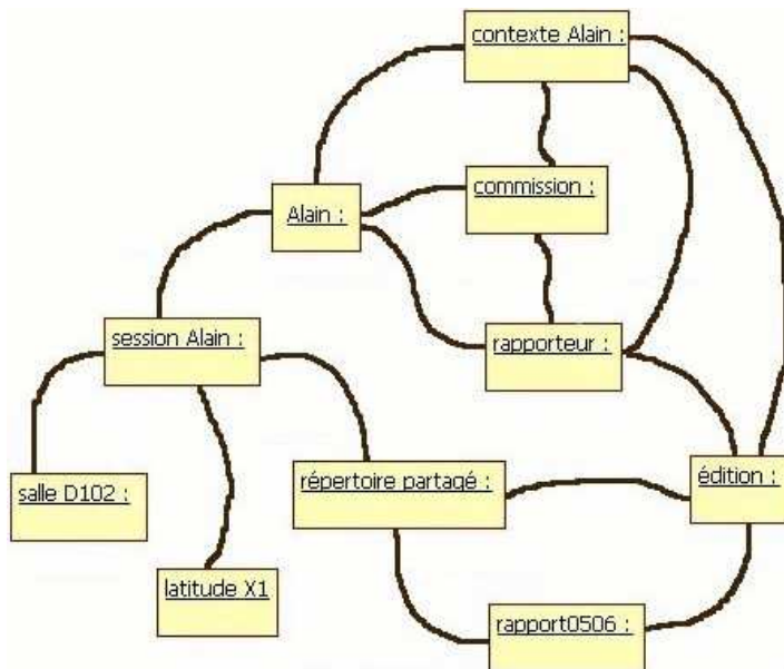
Figure 37. La représentation du graphe défini par l'objet de la classe Description de Contexte et les relations représentés dans la Figure 36 (quelques arêtes de ce graphe ont été omises afin de simplifier la présentation).
