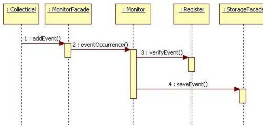
Figure 68. Traitement de l'occurrence d'un événement.
