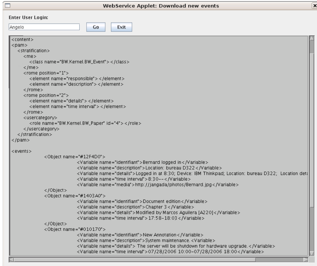
Figure 89. Exemple de retour de l'appel getEvents au service Web BW- \mathcal{M} .
