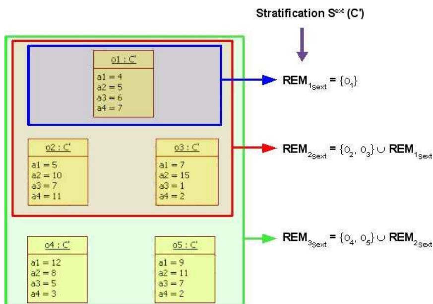
Figure 49. Exemple de stratification extensionnelle sur une classe.
