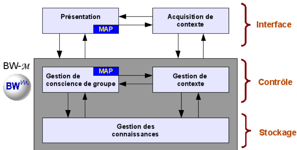
Figure 64. Architecture adoptée par le canevas BW- \mathcal{M} .
