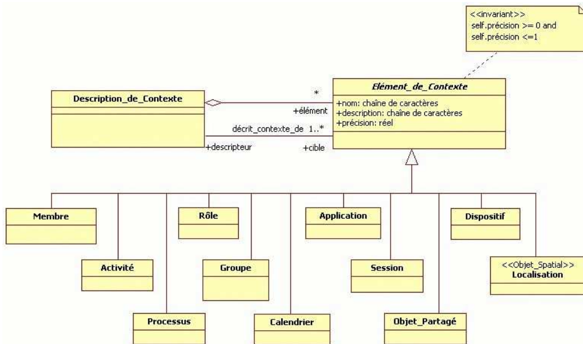
Figure 16. La description du contexte vue comme une composition d'éléments de contexte. 51
