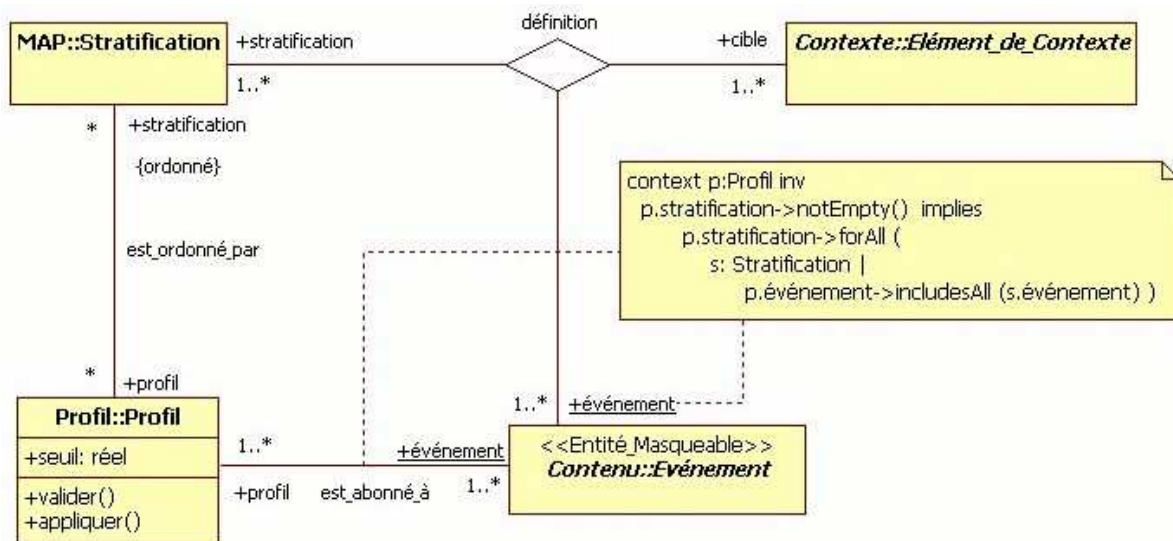
Figure 52. Un profil est abonné à un ensemble d'événements, organisés selon un ensemble de stratifications définies pour un élément cible.
