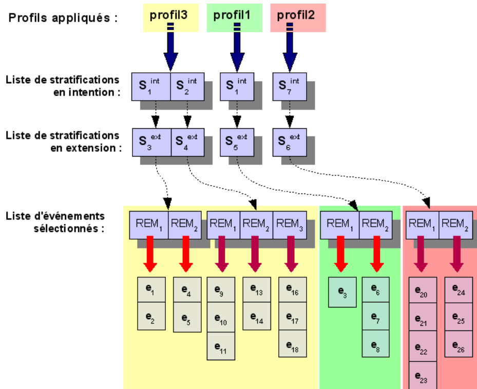
Figure 60. Structures résultant de la seconde étape du processus de filtrage.
