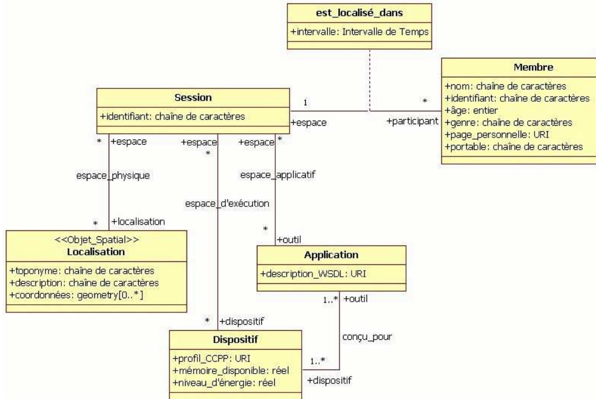
Figure 17. Classes et relations représentant un utilisateur qui se localise dans un espace réel et virtuel.
