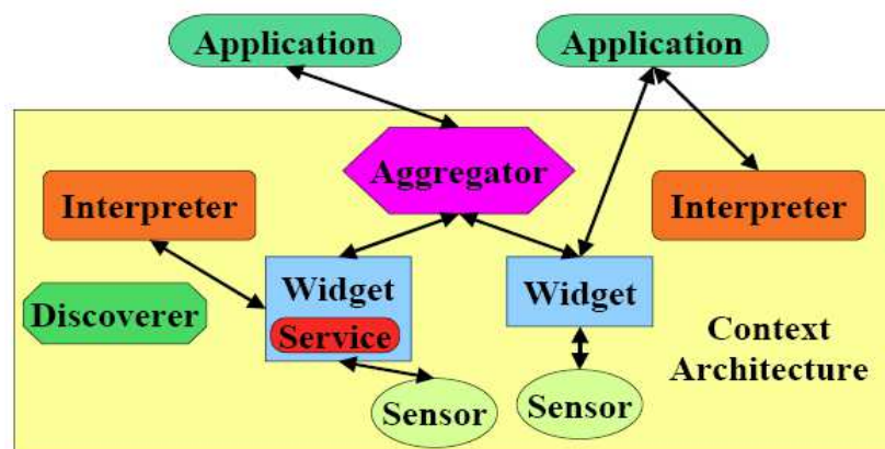
Figure 12. L'architecture du Context Toolkit d'après [Dey 2000].
