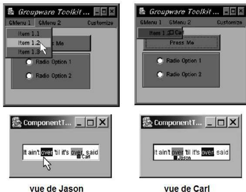
Figure 3. Deux exemples de widgets partagés disponibles dans la boîte à outils MAUI (un menu et une zone de texte) [Hill 2004]. À gauche, leur vue chez l'utilisateur Jason, et à droite leur vue distante, telle qu'un autre utilisateur, Carl, les percevra.
