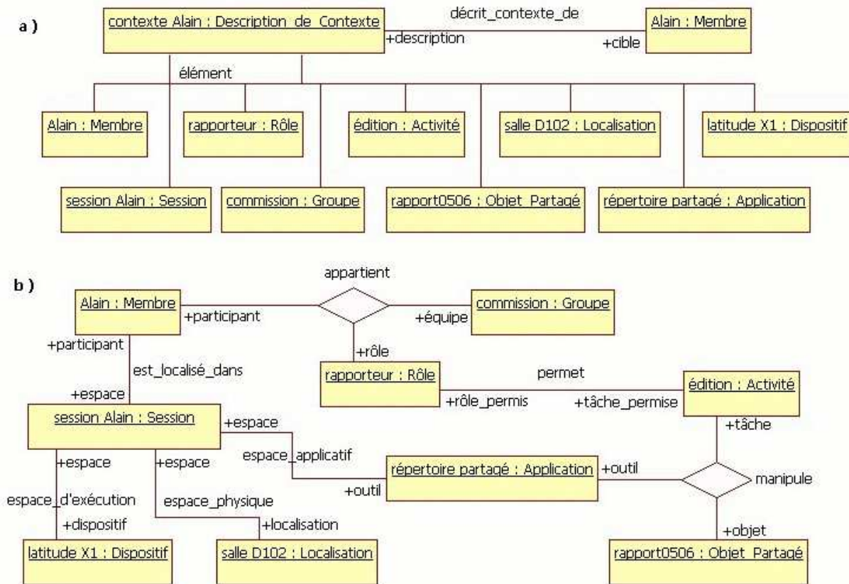
Figure 36. La représentation (en UML) d'un objet de la classe Description de Contexte, avec toutes les relations, directes (a) et indirectes (b), qu'il entretient avec d'autres instances de la base de connaissance.
