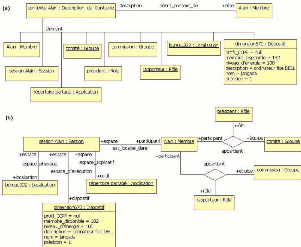
Figure 22. Exemple de description de contexte. En (a) les éléments qui composent cette description et, en (b) les relations entre ces éléments.
