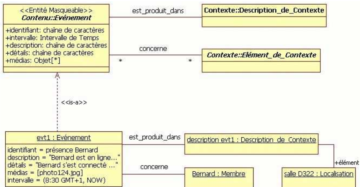
Figure 50. La classe événement représentant un type d'information de conscience de groupe et un exemple d'instance de cette classe.
