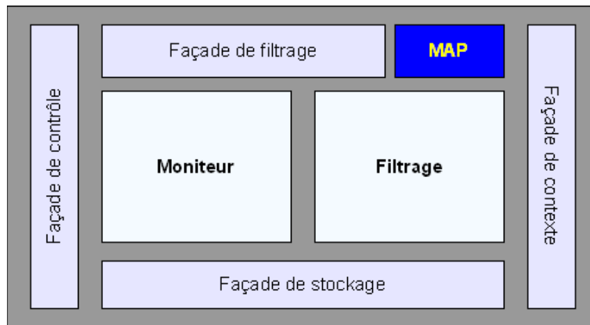
Figure 65. Structure interne de l'unité de gestion de conscience de groupe.
