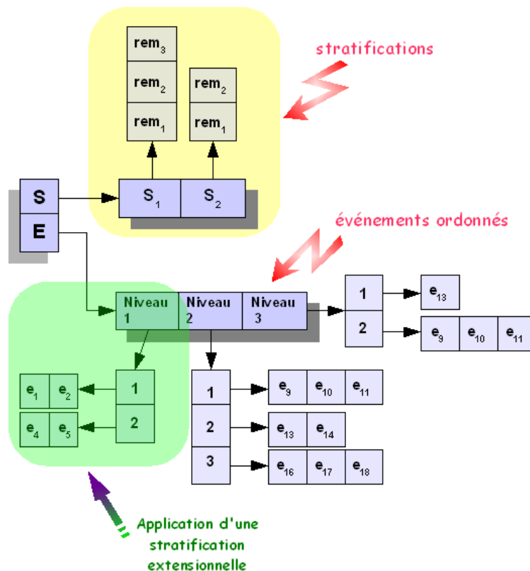
Figure 73. Structure de données retournée par le processus de filtrage.
