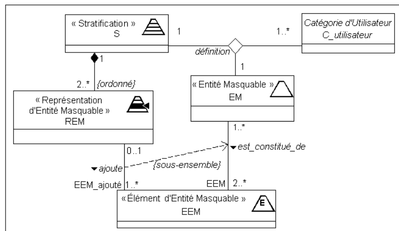
Figure 47. Modèle d'Accès Progressif, décrit à l'aide des stéréotypes en UML (d'après [Villanova 2002]).
