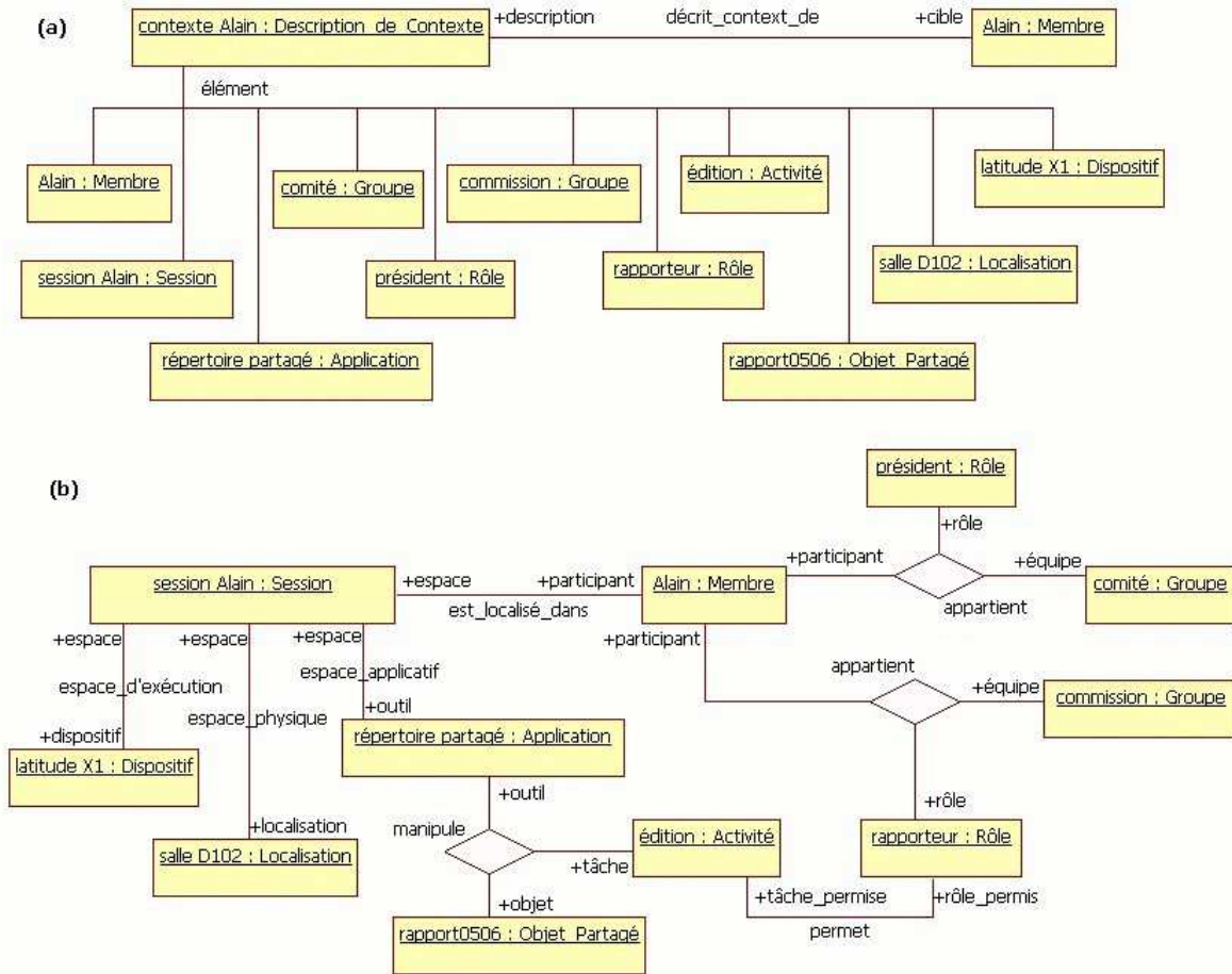
Figure 55. Un exemple du contexte d'un utilisateur, avec tous les objets qui le composent en (a), et en (b), les relations qui lient ces objets entre eux.
