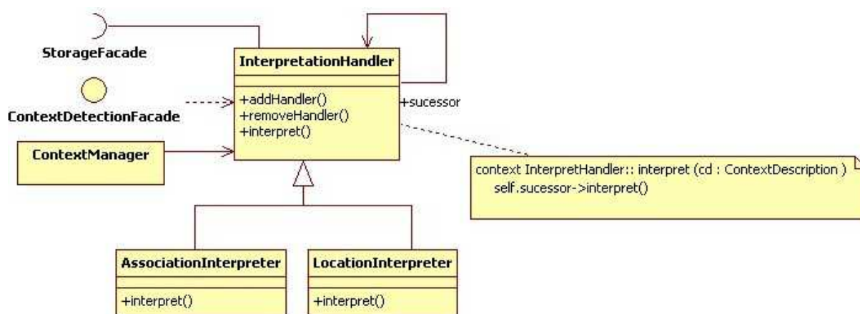
Figure 76. Structure responsable de l'interprétation des informations contextuelles.
