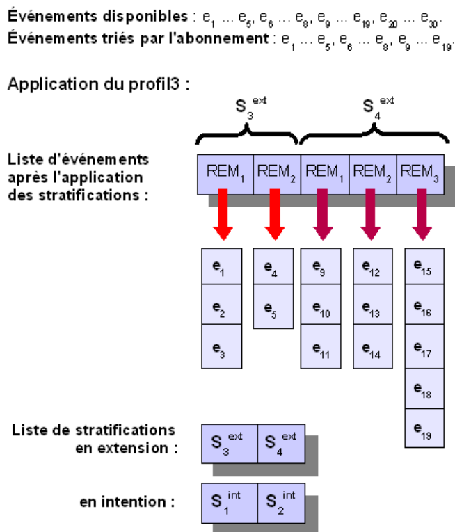
Figure 57. Exemple d'application d'un profil sur un ensemble d'événements.
