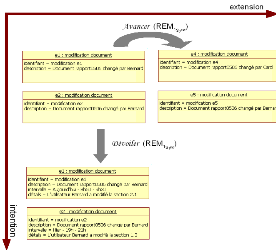
Figure 61. Exemple de l'application des opérations sur les stratifications en extension et en intension.
