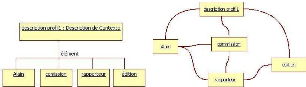
Figure 38. A droite, la représentation (en UML) de l'objet description_profil1 , instance de la classe Description de Contexte , et ses relations directes. A gauche, le graphe défini par cet objet.
