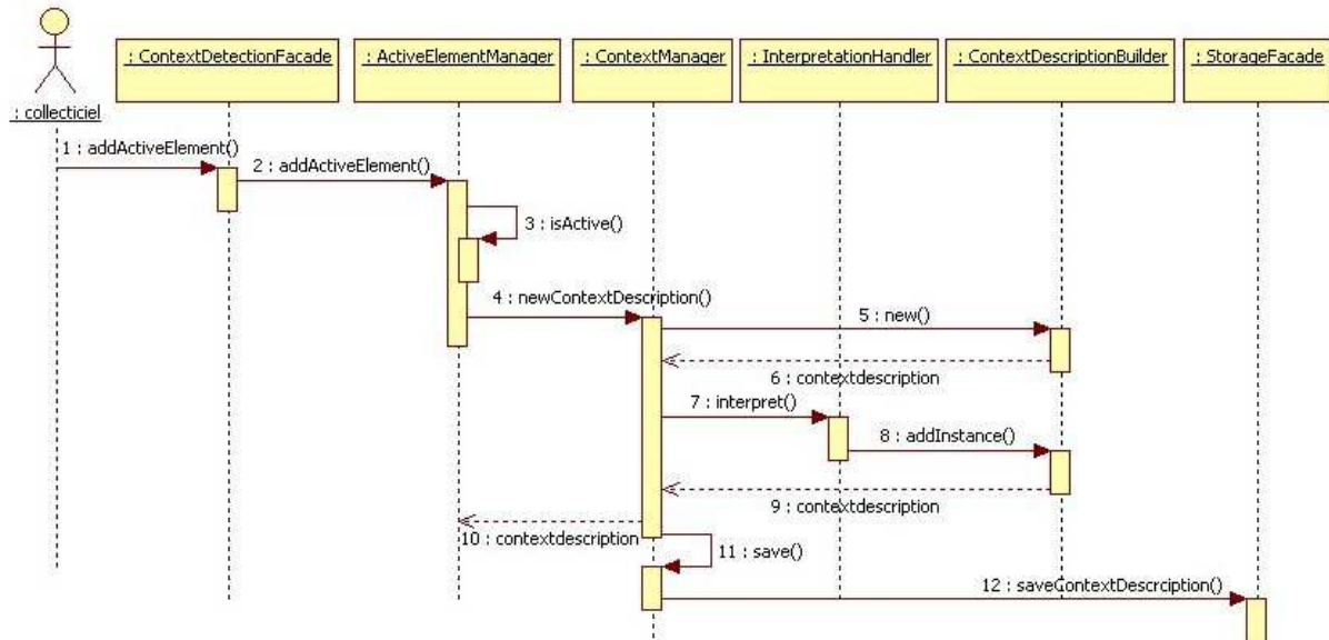
Figure 78. Diagramme de séquence représentant le processus déclenché à l'intérieur du canevas BW-M par l'introduction d'un nouvel élément actif dans le système.
