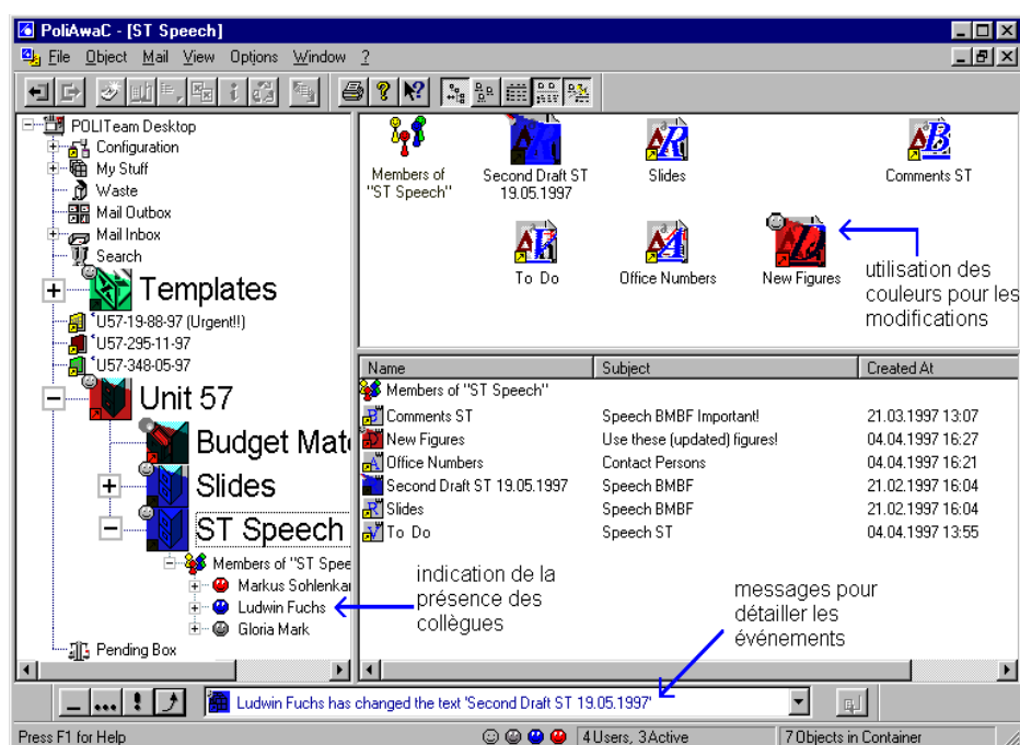
Figure 4. L'environnement POLITeam [Sohlenkamp 1998] et ses mécanismes de conscience de groupe.
