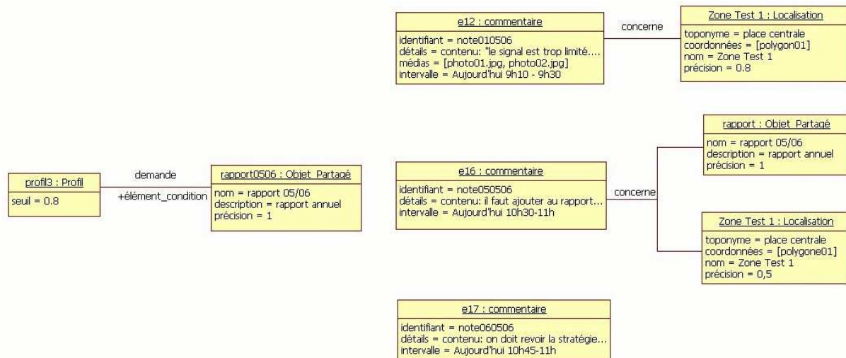
Figure 59. Comparaison entre un élément condition associé à un profil et les éléments de contexte concernés par certains événements.
