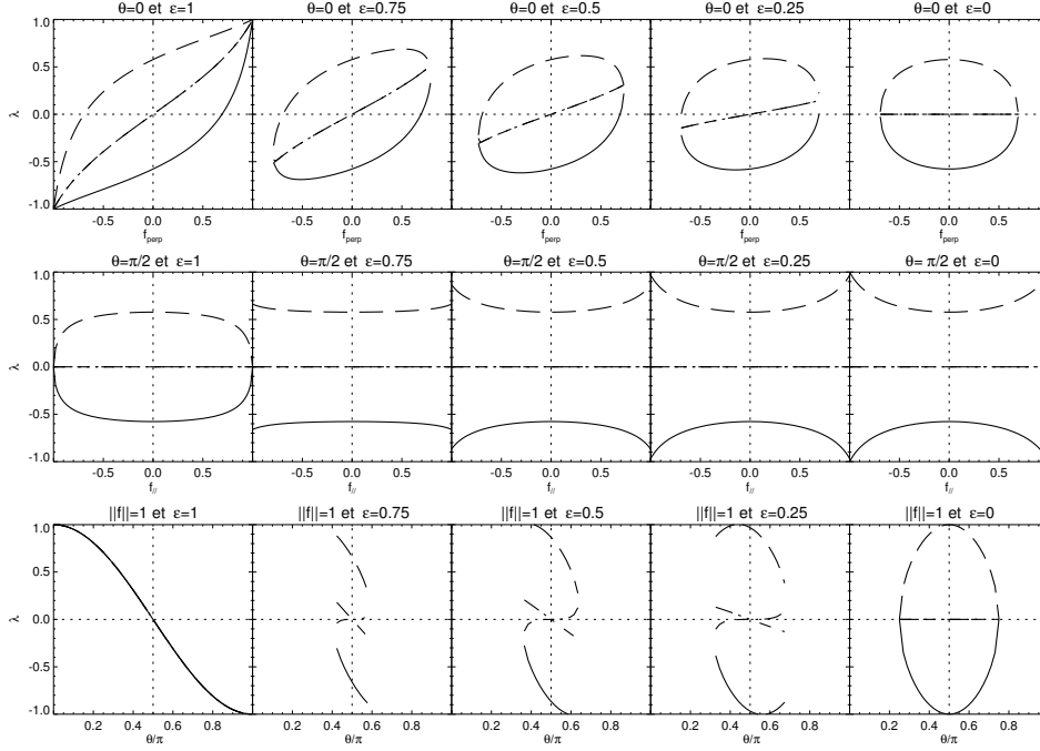
FIG. 2.2 – Valeurs propres analytiques de la matrice jacobienne normalisées par c en fonction de \theta , f et \epsilon .
