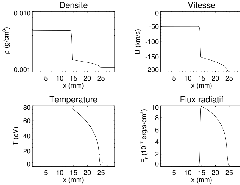
FIG. 4.2 – Profils caractéristiques d'un choc radiatif.
