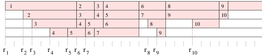
Figure 4.4. Un ordonnancement irréductible
