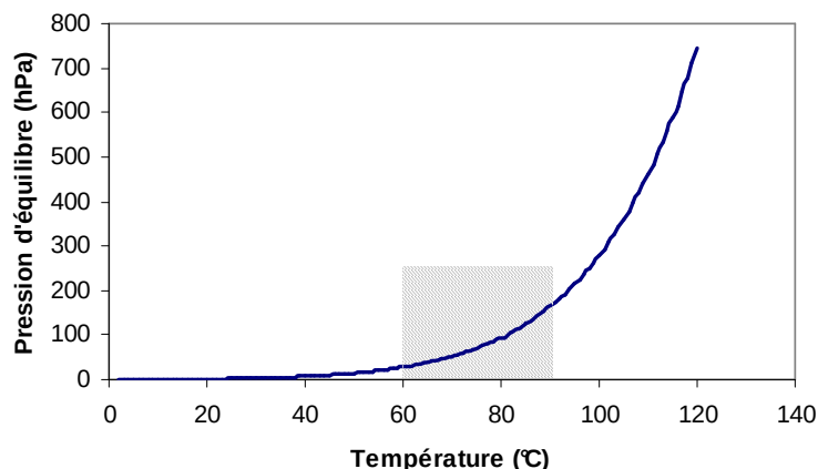
Figure 2.2 : Courbe d'équilibre thermodynamique P(H_2O)=f(T) avec les domaines de stabilité de Li_2SO_4 \cdot H_2O et Li_2SO_4 .
