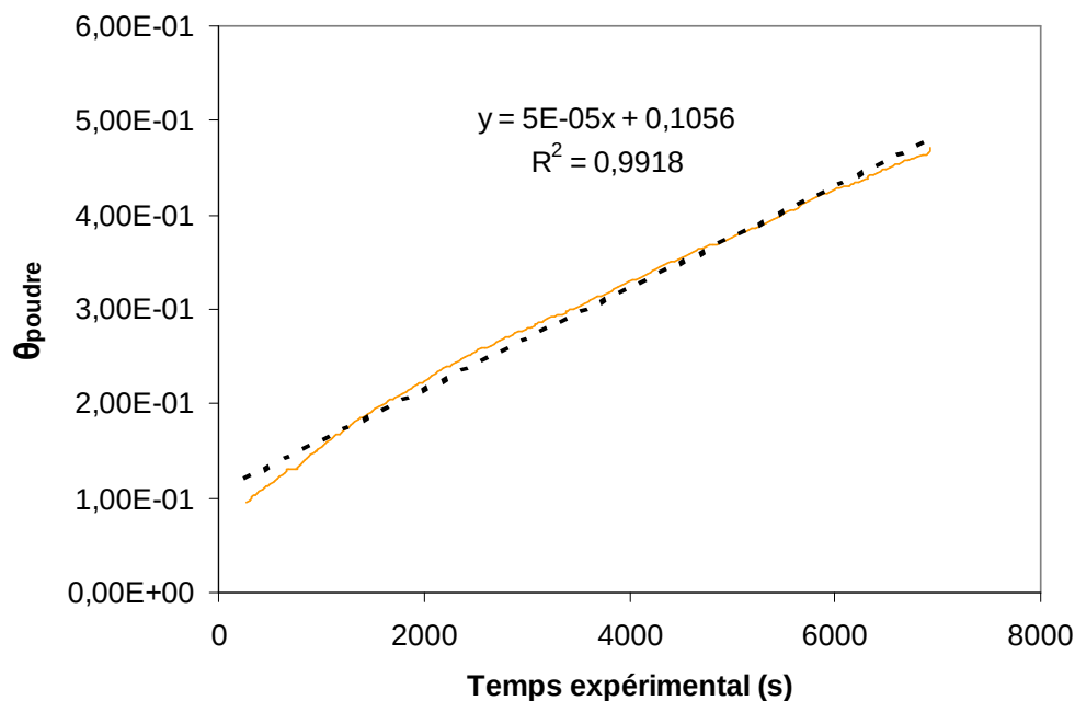
Figure 3.10 : Représentation du temps adimensionné en fonction du temps expérimental pour une poudre déshydratée à 80°C sous une pression de vapeur d'eau de 2,6 hPa.
