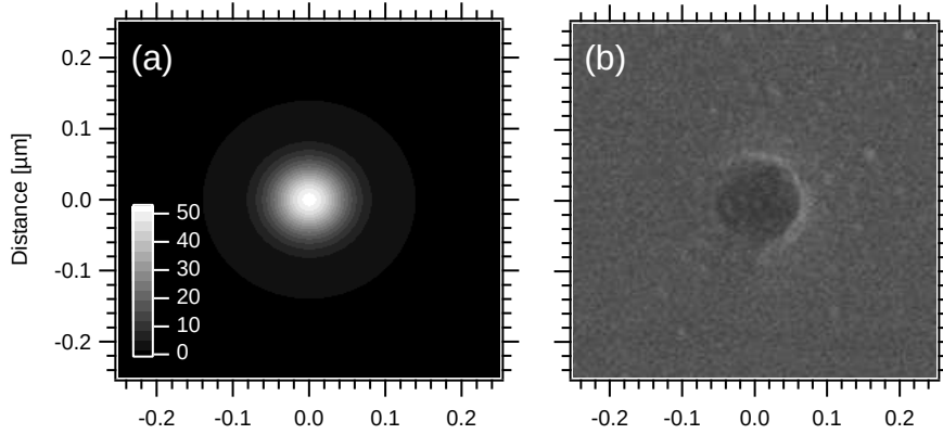
FIG. 7.7 – Comparaison entre la distribution d'intensité donnée par la solution de Mie (a) et les cratères observés par MEB (b). Le calcul correspond à l'irradiation d'une sphère de silice ( n = 1,6 ) de rayon R = 250 nm à la longueur d'onde \lambda_{las} = 193 nm. On constate une exaltation sur une zone de diamètre (mesuré à 1/e^2 ) d'environ 150 nm. Comme le montre l'image (b) correspondant à une fluence de 430 \text{ mJ cm}^{-2} , il existe une bonne adéquation entre cette taille et la dimension des cratères observés sur Si pour des fluences variant de 300 à 700 \text{ mJ cm}^{-2} .
