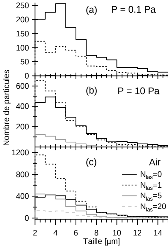
FIG. 7.3 – Distributions en taille des particules de carbone après irradiation avec une fluence F_{las} = 450 \text{ mJ cm}^{-2} sous différentes atmosphères. Pour chaque pression, les histogrammes sont donnés après 1, 5 et 20 tirs lasers.
