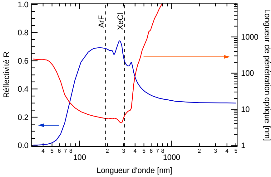
FIG. 4.1 – Réflectivité R_s et longueur de pénétration optique \delta_{opt} = 1/\alpha = \lambda/4\pi\kappa du silicium en fonction de la longueur d'onde \lambda_{las} . Les courbes sont réalisées d'après les données de la référence [84].
