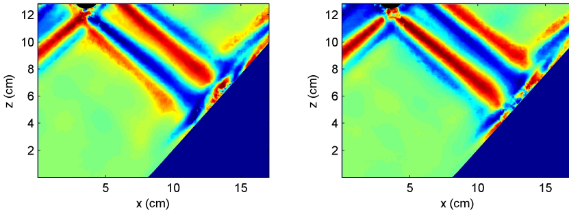
a) b) Fig. 8.6. Gradients horizontal (a) et vertical (b) de densité visualisés par strioscopie synthétique lors d'une expérience de réflexion critique.
