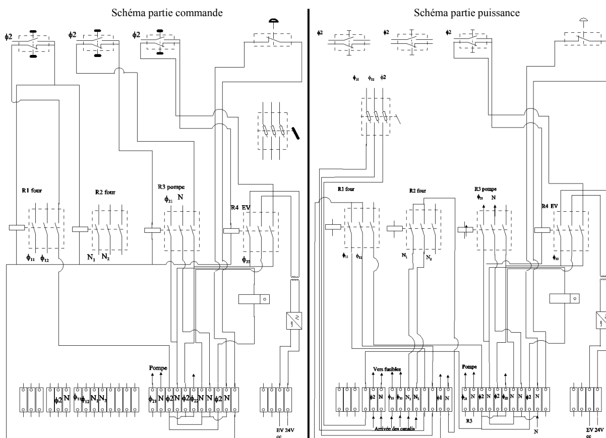
Figure 156. Schémas de câblage des parties de commande et de puissance de l'armoire électrique.
