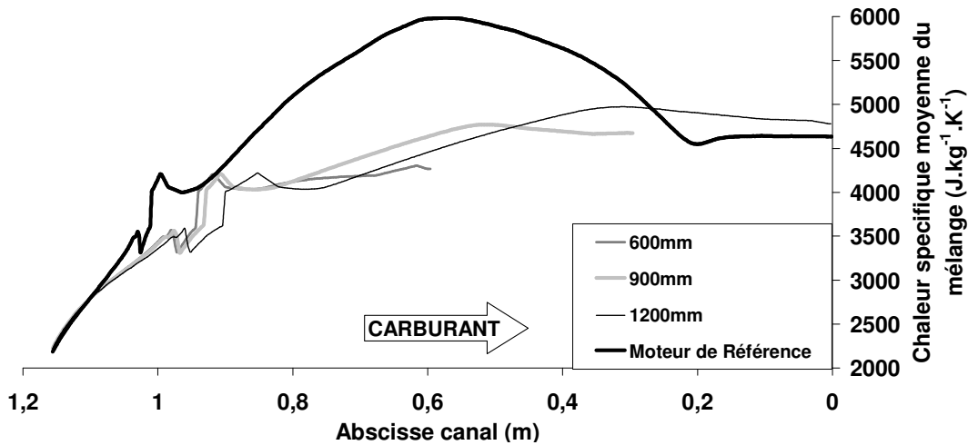
Figure 143. Profil de capacité thermique du fluide le long du canal pour une configuration entretoises (largeur 8 mm) avec un débit de 0,1 \text{ g.s}^{-1} et une température maximum de four de 1300^\circ\text{C} .
