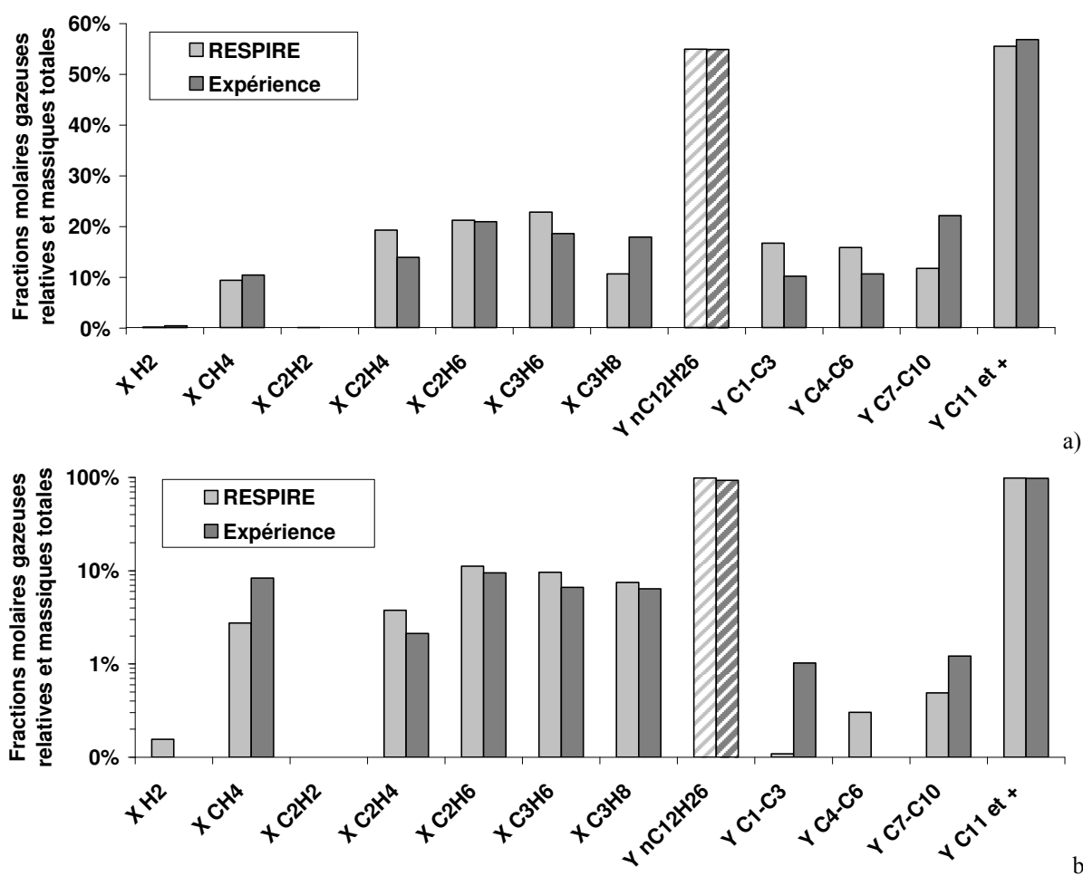
Figure 125. Répartition molaire des espèces de la phase gazeuse et fraction massique du n-dodécane dans les produits de pyrolyse à : 50 bars, 0,05 g.s -1 et 773 K (a); 50 bars, 0,1 g.s -1 et 923 K (b)
