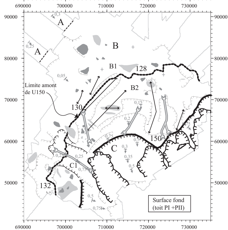
Figure III-40B Interprétation de la carte isohypse temps double : principaux traits morphologiques de la surface au fond (voir carte en Annexe C).
