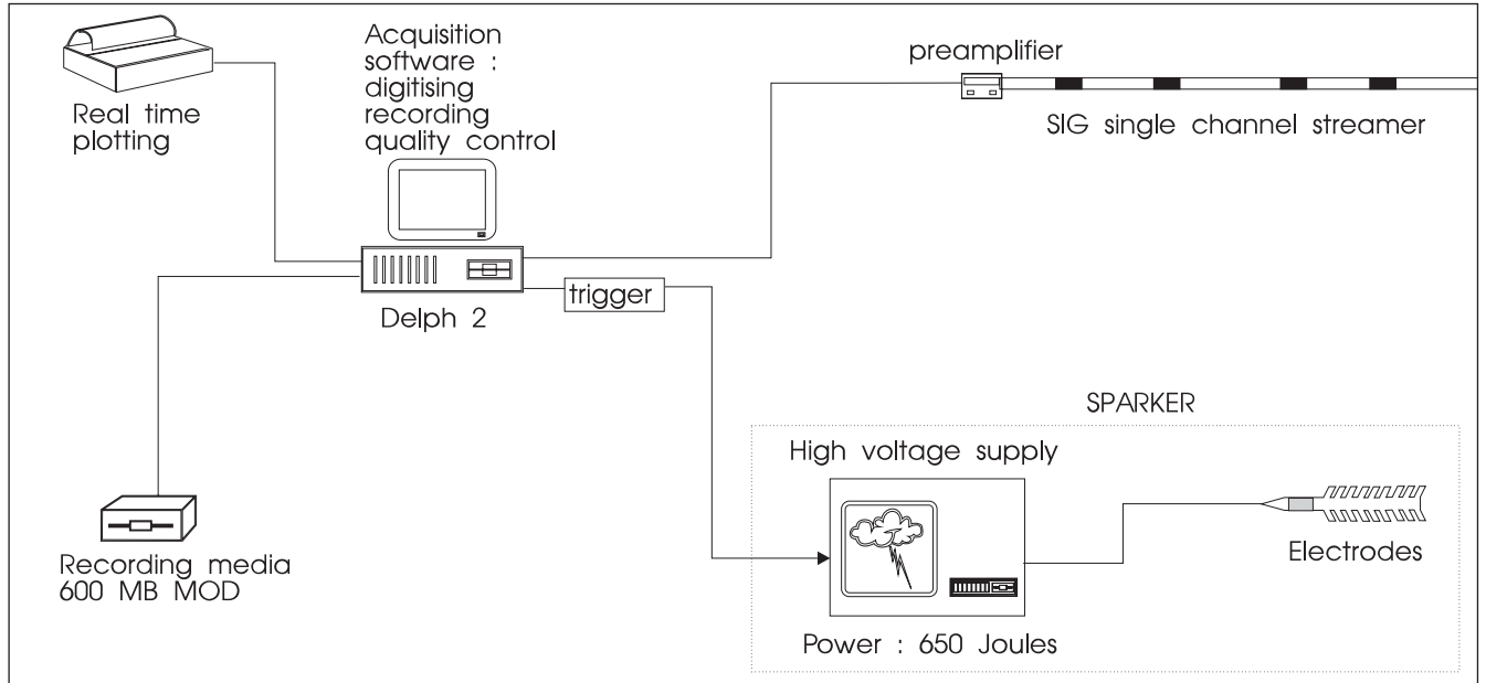
Figure III-5 Synoptique d'acquisition de la sismique très haute résolution (H. Nouzé, 1998).
