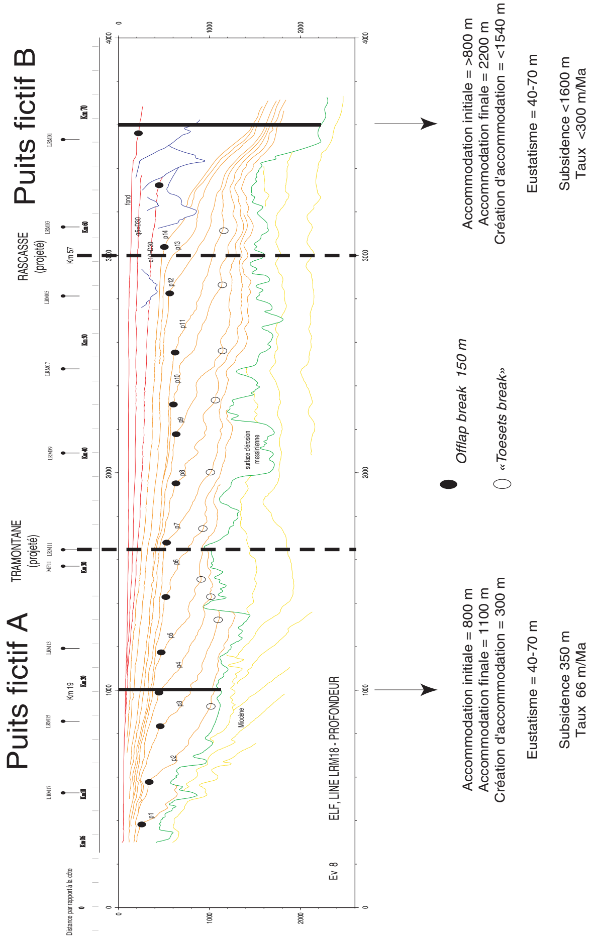
Figure VII-9 Calcul de l'accommodation et de la subsidence en deux puits fictifs A et B. L'accommodation initiale correspond au début du Pliocène, l'accommodation finale correspond à l'actuel.
