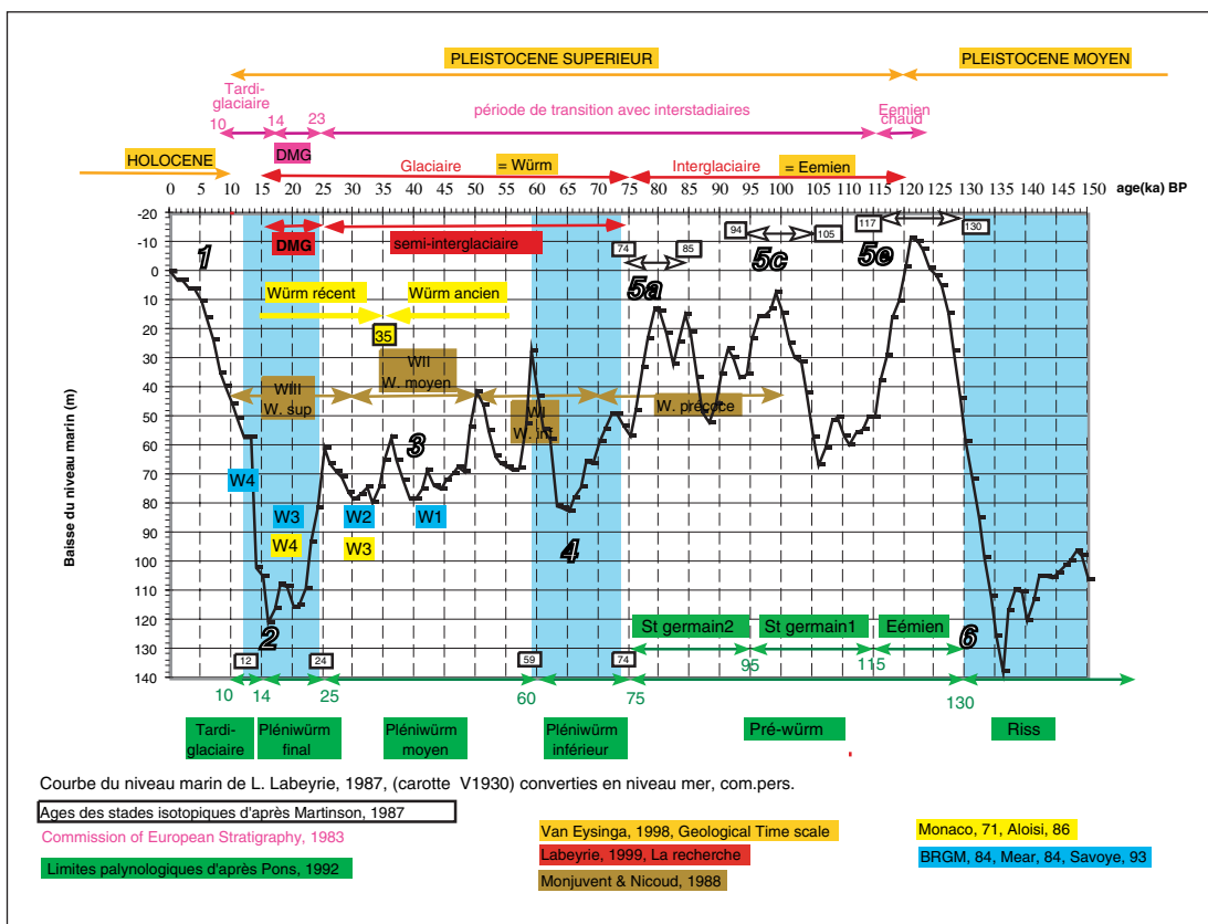
Figure II-36 Compilation des cor- rélation entre les chronologies strati- graphie, isotopique, palynologique et glaciaire, pour les derniers 150 ka (Dernier cycle gla- ciaire/interglaciaire).
