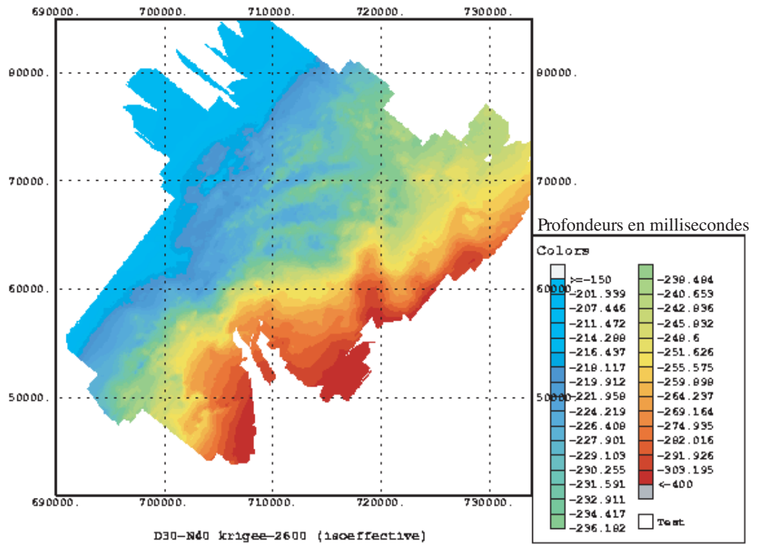
Figure III-15 Carte isohypse (temps-mstd) interpolée (krigée) de la surface D30.
