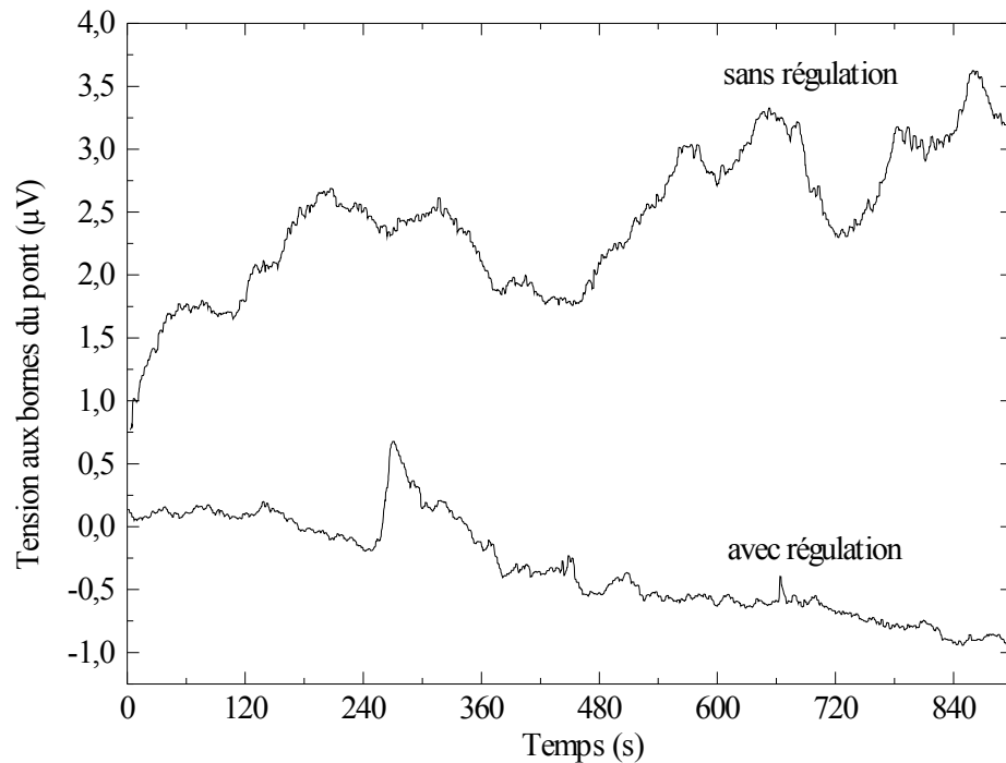
figure 3-56: Evolution de la tension aux bornes du méandre avec et sans la régulation de température.
