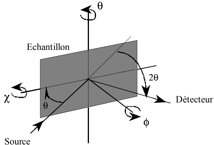
figure 2-5: Configuration de mesure pour l'enregistrement de \phi -scans.
