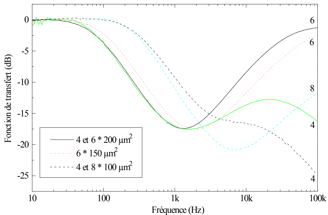
figure 3-22: Fonctions de transfert normalisées à 0 dB au plateau, mesurées sur des ponts de largeurs 4, 6 ou 8\ \mu\text{m} et de longueurs 100, 150 ou 200\ \mu\text{m} (série BOLO2)
