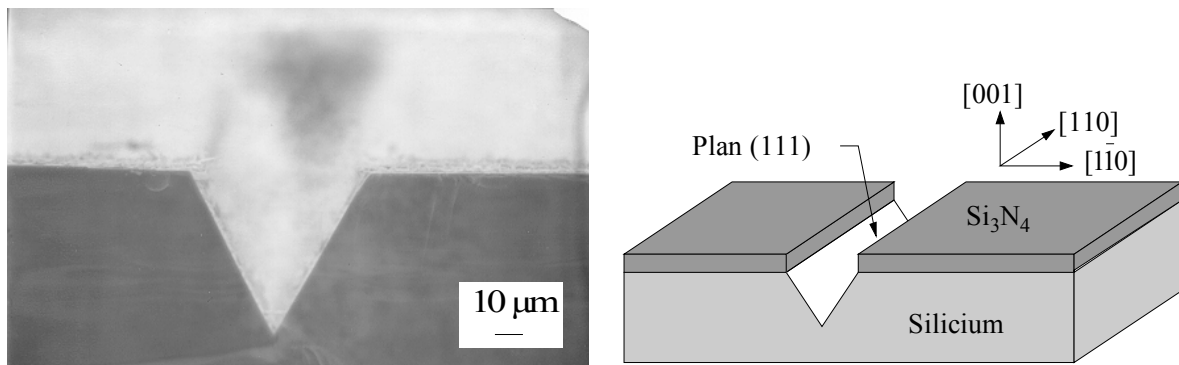
figure 2-32: Profil de gravure du silicium lorsque la fente est alignée par rapport à [110] .
