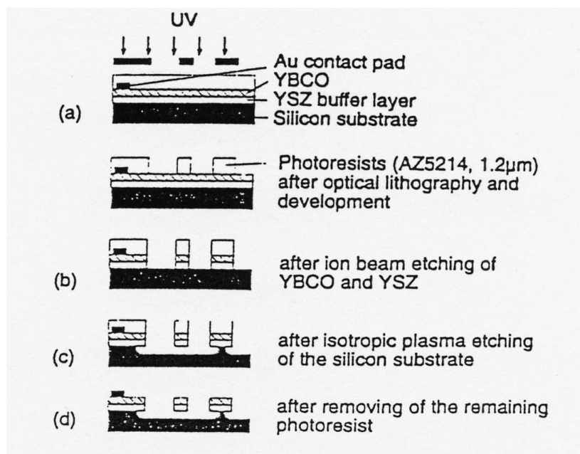
figure 1-14: Procédé de fabrication d'un bolomètre suspendu YBaCuO par gravure ionique réactive développé par Barth et al. [58].
