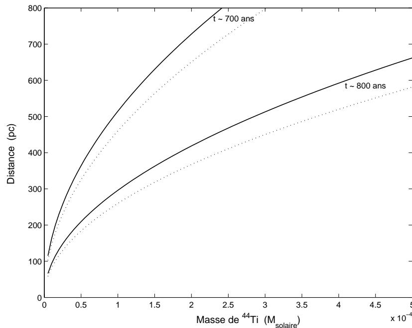
FIGURE 6.5 – Distance en fonction de la masse de ^{44}\text{Ti} produite pour un âge supernova de 700 et 800 ans. La distance d est déterminée par la relation 6.2 pour deux périodes de ^{44}\text{Ti} : 90,4 ans (en trait plein) et 87,5 ans (en pointillé).
