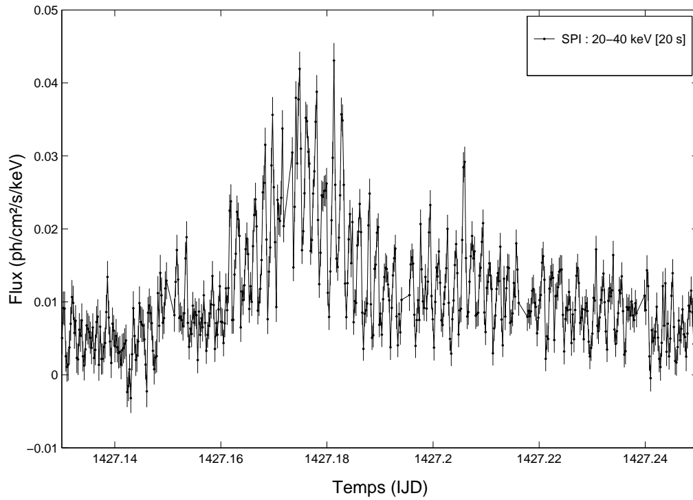
FIGURE 6.26 – Courbe de lumière SPI du sursaut de Vela X-1 durant l’orbite 139 avec une résolution en temps de 20 s.
