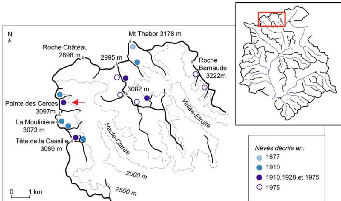
Figure D-48: Cartographie des névés décrits au PAG.
