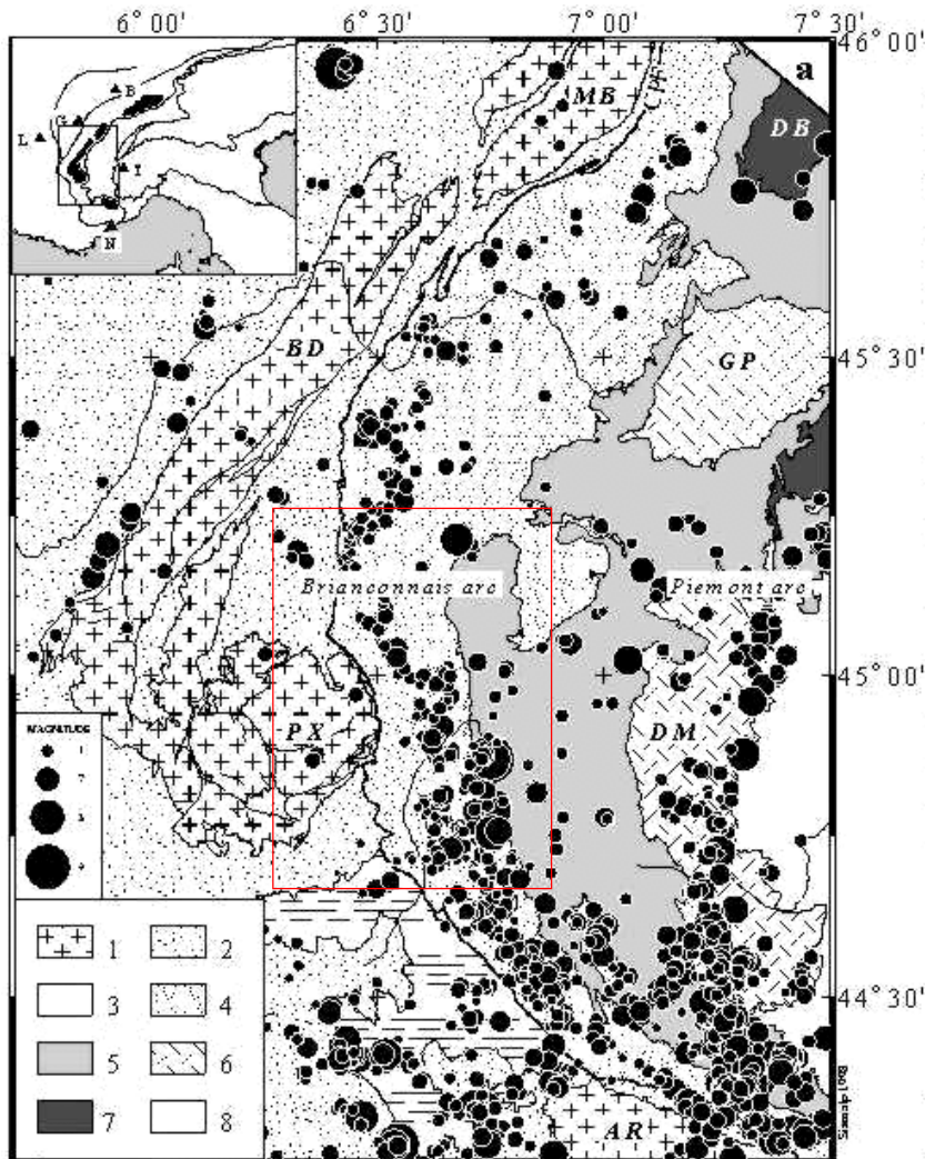
Figure C-71 : Carte de la sismicité actuelle (Sue, 1998 ; Sue et al. , 1999)
