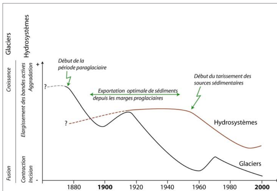
Figure D-115 : Evolution des hydrosystèmes à l'aval de marges glaciaires soumise à des entraves (Ex. Mme Carle, Tabuc).
