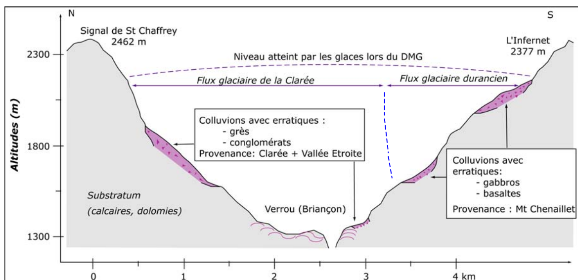
Figure C-11 : Niveau atteint par le glacier Clarée - Durance au niveau du bassin de Briançon.
