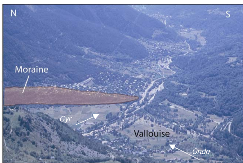
Figure C-43 : Aperçu de la moraine de Vallouise (rive gauche de la Gyronde).
