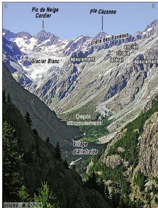
Figure C-75 : Aperçu du dépôt d'éroulement du Pré de Madame Carle.
