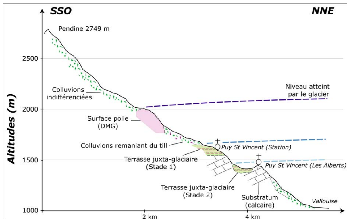
Figure C-42 : Les principales étapes de l'amincissement du glacier de la Gyronde après le Pléniglaciaire, dans le bassin de Vallouise.
