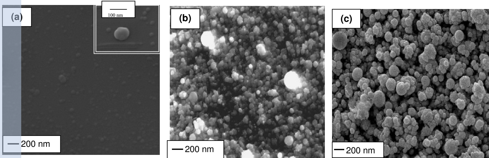
Figure 3-3 : Images de films (a) ta-C, (b) nickel et (c) tantale élaborés à une fluence moyenne de 2,6 \text{ J/cm}^2 , obtenues par microscopie électronique à balayage à émission de champ.
