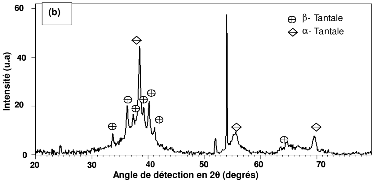
Figure 3-18 : spectre de diffraction des rayons X du film C :Ta 15% at. sous incidence rasante (a) de 0,3^\circ et (b) de 0,7^\circ
