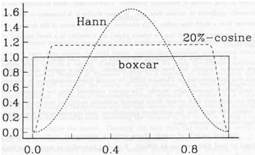
Fig. 1 Comparaison des fenêtres rectangulaire, de Hanning et 20% cosin bell.
