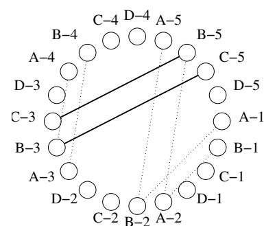
FIG. 4.6: Graphe de correspondances, identification du segment L2.
