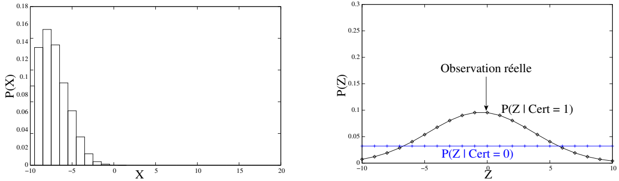
FIG. 4.41: Situation A : estimation de l'état (à gauche) et comparaison des mesures prédites avec la réalité.
