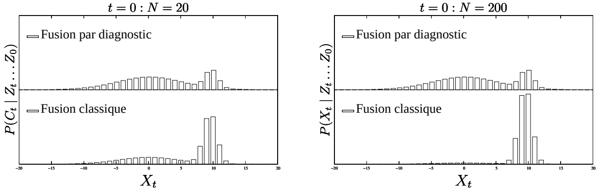
FIG. 4.32: État des filtres après observation d'un faux-positif à t = 0 .
