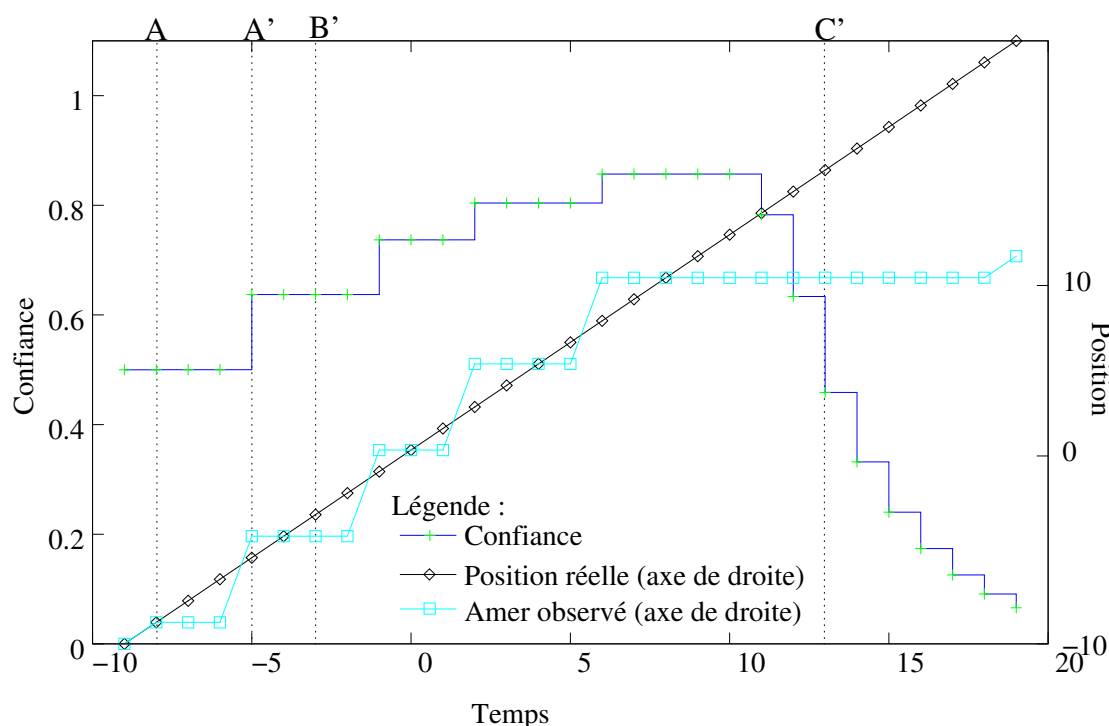
FIG. 4.46: Évolution de la confiance au cours du mouvement.
