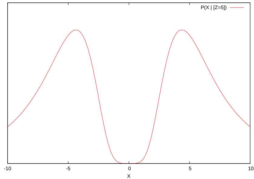
FIG. 2.4: Distribution de probabilité correspondant à la question P(X \mid [Z = 5]) .
