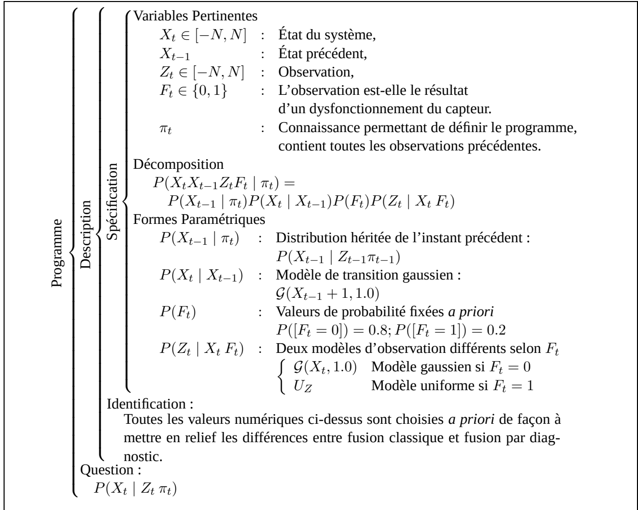
FIG. 4.29: Filtre bayésien par fusion classique
