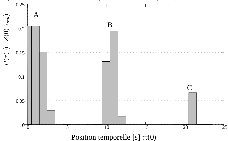
Estimation de la localisation temporelle initiale P(\tau(0) | Z(0) T_{sm}) . Les trois hypothèses exprimées par les trois pics de la distribution correspondent aux points de vue A, B et C sur le tracé du trajet. La position réelle est la position A.
