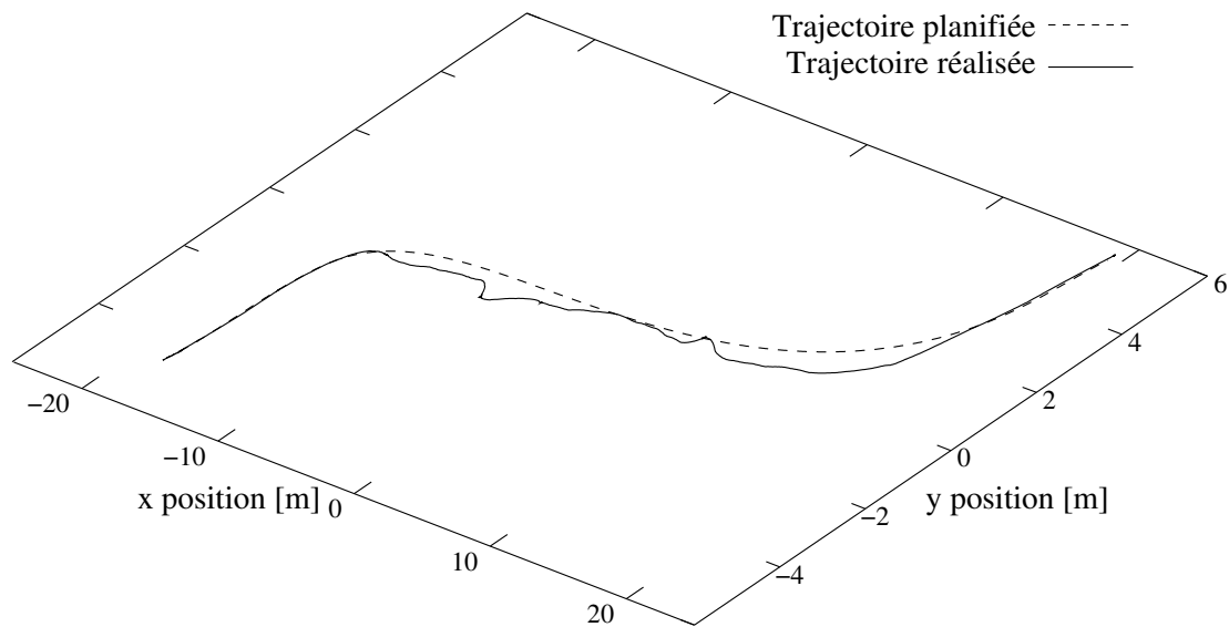
FIG. 7.14: Comparaison d'une trajectoire planifiée et de la trajectoire exécutée correspondante. La trajectoire est fortement déformée par la différence d'échelle entre les deux axes.
