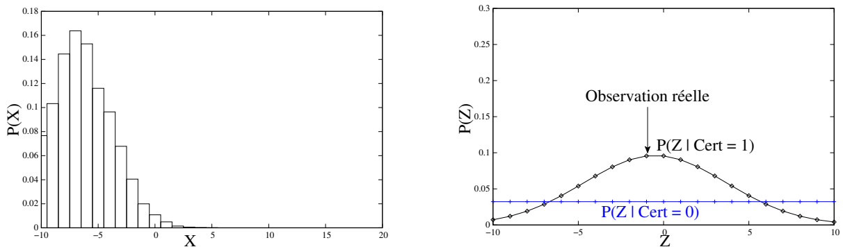
FIG. 4.42: Situation B : estimation de l'état (à gauche) et comparaison des mesures prédites avec la réalité.
