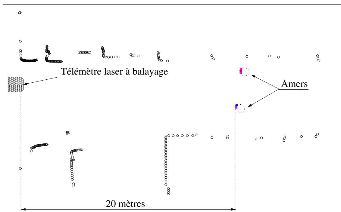
FIG. 7.10: Exemple de résultat renvoyé par le Sick sur le parking de l'INRIA.
