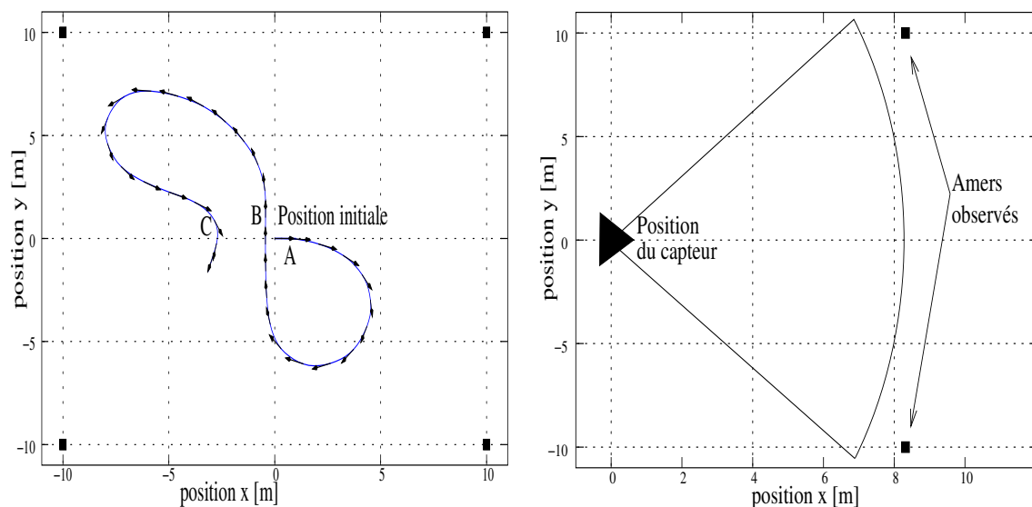
A gauche : Trajet initial dans un environnement avec quatre amers sur un carré (carrés noirs). Pour plus de clarté, le trajet géométrique est représenté ici, mais c'est le trajet sensorimoteur qui est utilisé par la localisation. A droite : Perception initiale dans le repère capteur.
