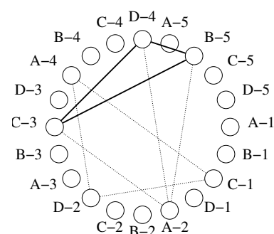
FIG. 4.17: Graphe de correspondances, identification du triangle T4.
