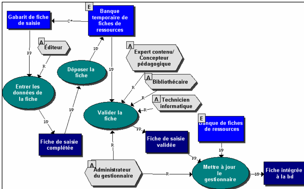
Figure 8 Exemple de détail de scénario générique (un modèle de l'élaboration d'une banque de ressource)
