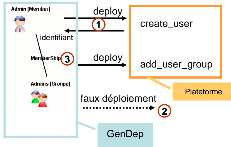
Figure 86 Ecriture d'une méthode deploy différée, réalisée par le lien.
