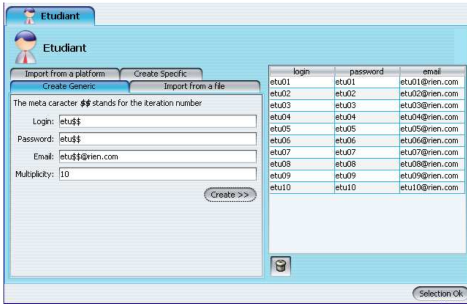
Figure 90 Génération itérative utilisant un masque de profilage
