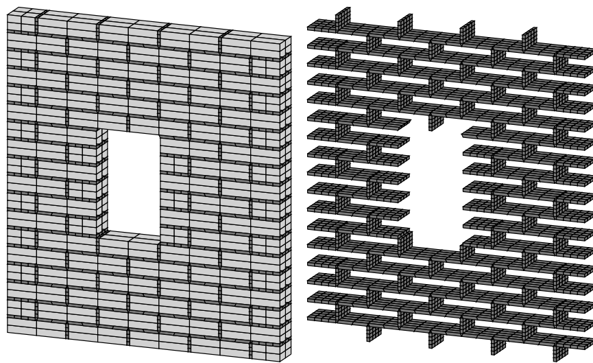
FIGURE 7.24 – Maillage tridimensionnel du problème
